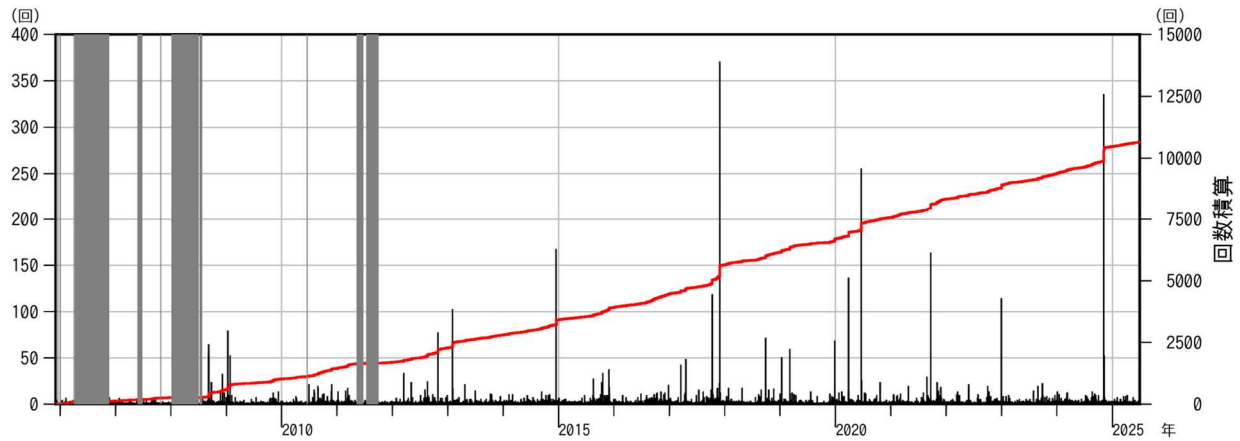
図 3 白山 日別地震回数と積算回数（2005 年 12 月 1 日～2025 年 6 月 30 日）
