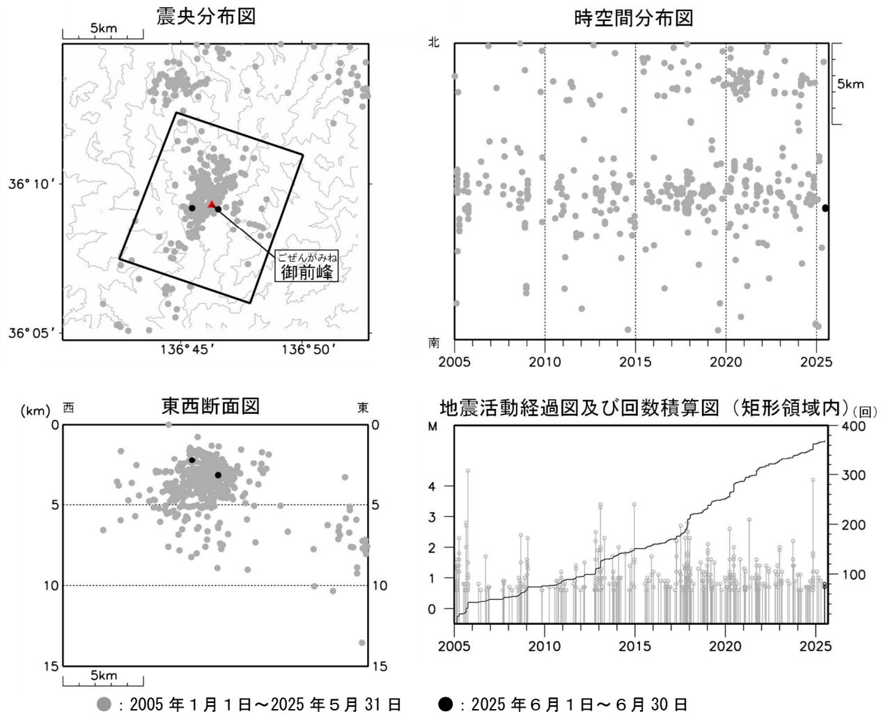
図 4 白山 広域地震観測網による山体・周辺の地震活動（2005 年 1 月 1 日～2025 年 6 月 30 日）
