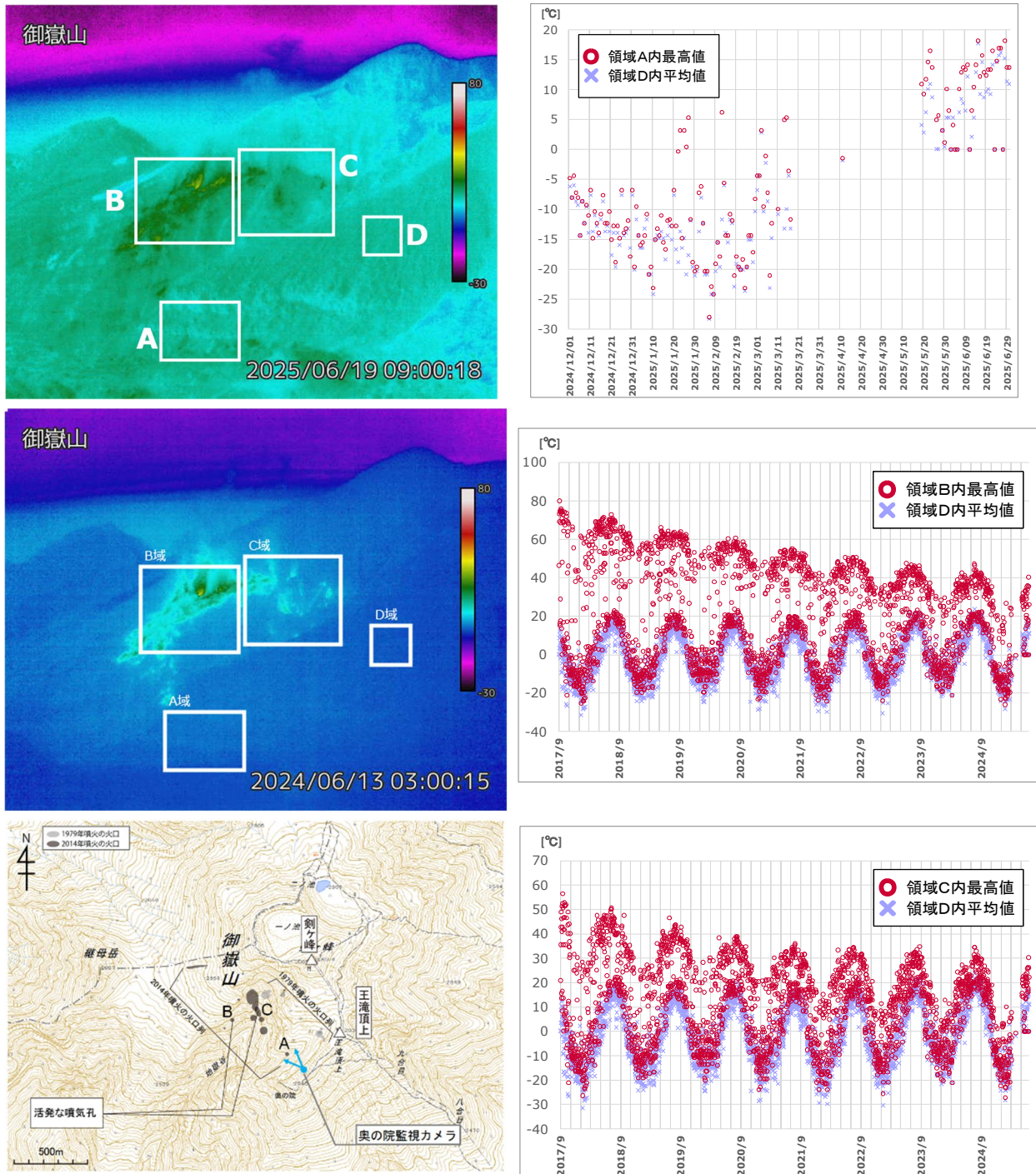
図3 御嶽山 奥の院赤外熱映像カメラによる地獄谷火口における最高温度の推移 (2017 年 9 月 13 日～2025 年 6 月 30 日)
