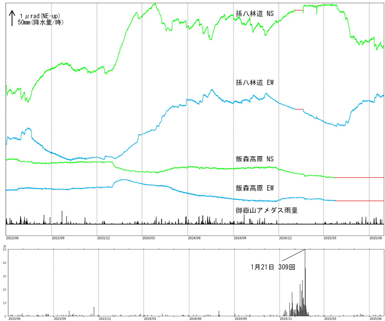
図7 御嶽山 傾斜変動と日別地震回数の推移（2023年6月1日～2025年6月30日） データは時間平均値で、孫八林道観測点のデータは潮汐補正済みです。 赤線部分は欠測を示します。 2024年1月以降、「令和6年能登半島地震」に伴うとみられる変動が認められます。
