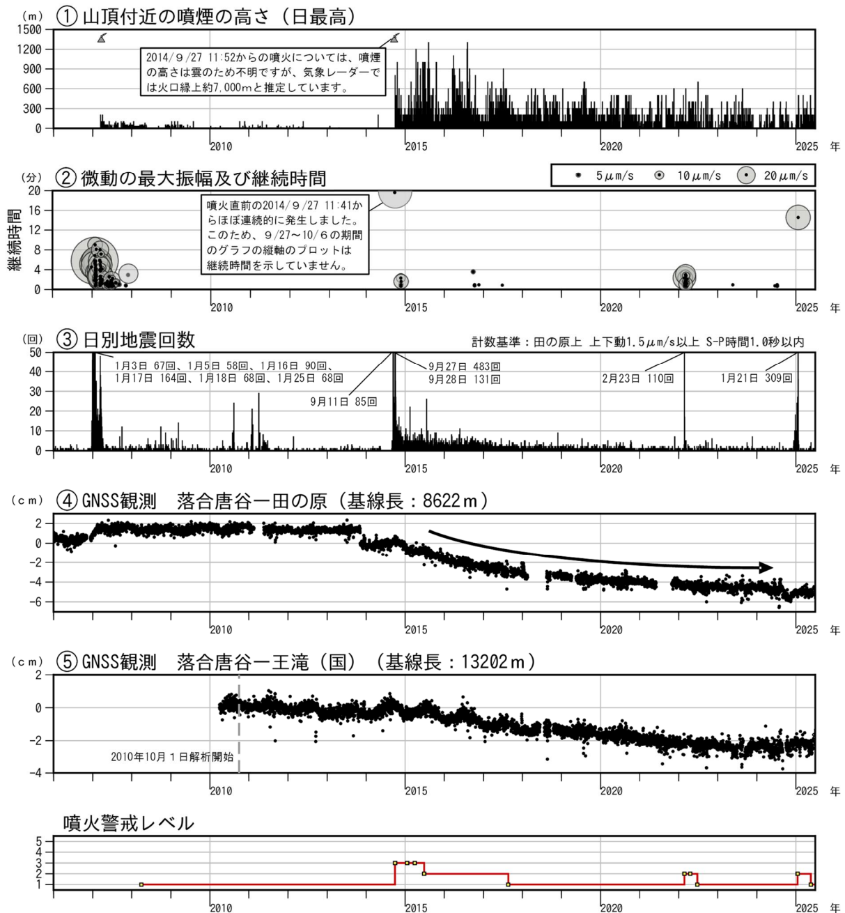
図1 御嶽山 長期間の火山活動経過図（2006年1月1日～2025年6月30日）
