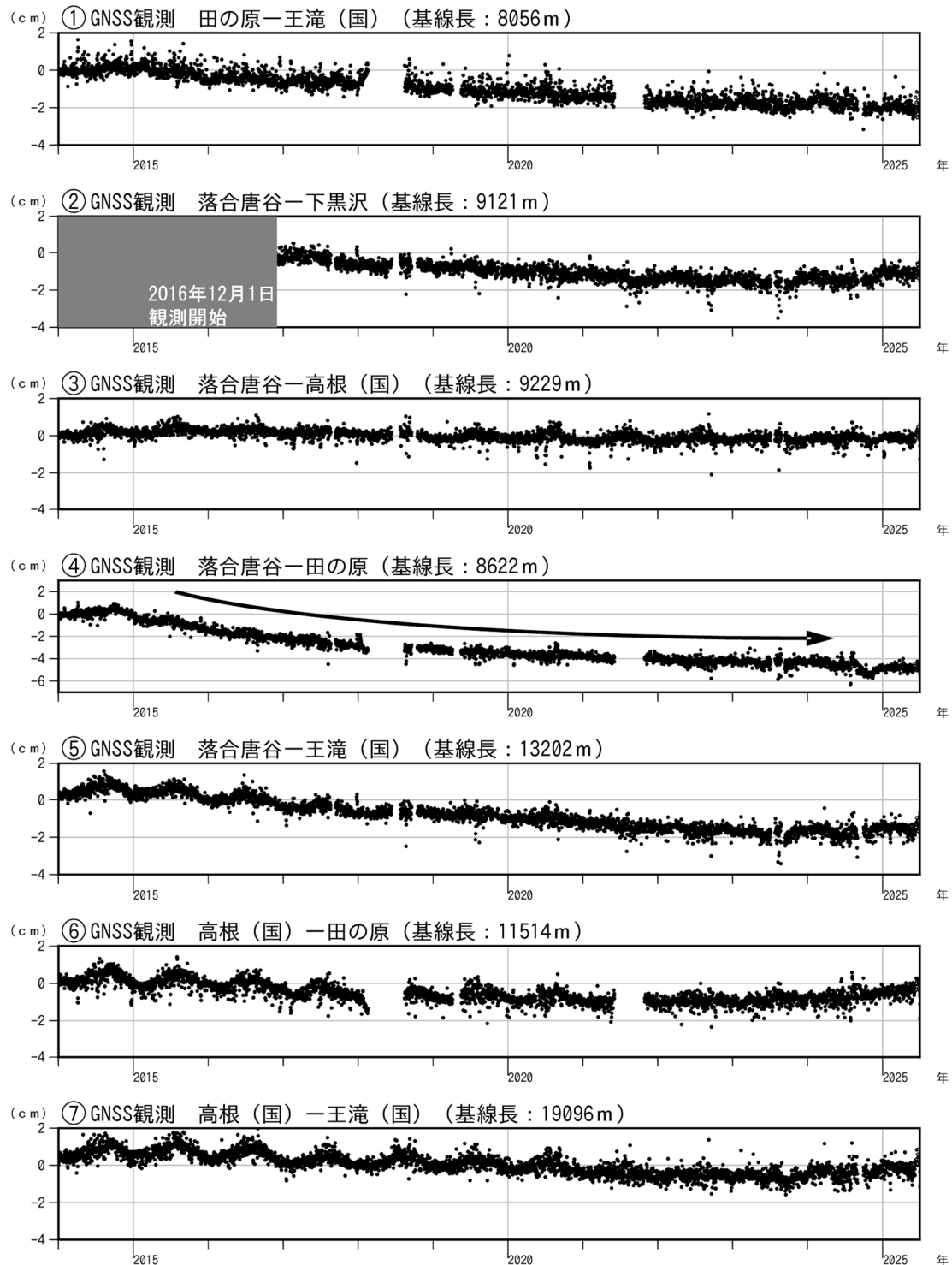
図5 御嶽山 GNSS 連続観測結果（2014 年 1 月 1 日～2025 年 6 月 30 日）
