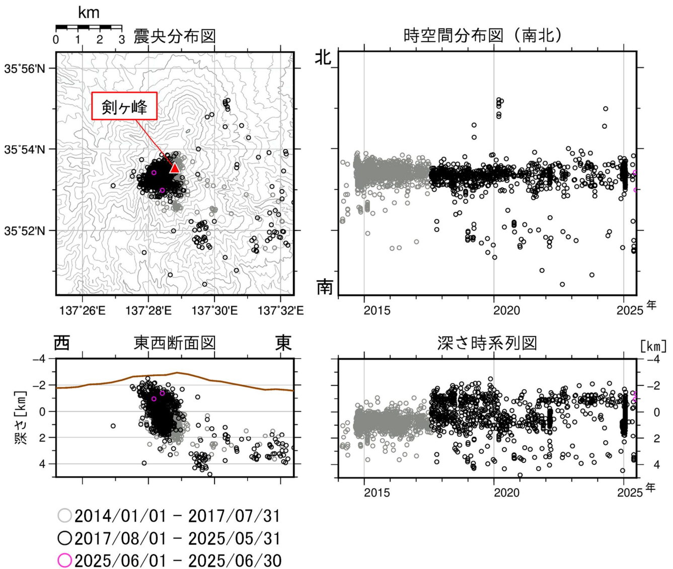
図4 御嶽山 震源分布図（2014年1月1日～2025年6月30日）
