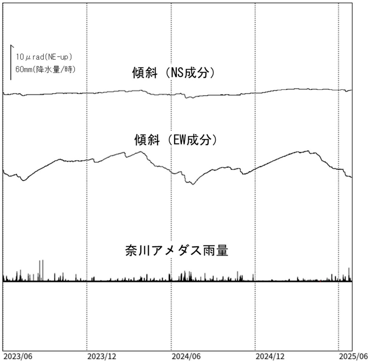
図4 乗鞍岳 三本滝観測点における傾斜データ（2023年6月1日～2025年6月30日） ・傾斜計による観測では、火山活動によるとみられる変動は認められません。
