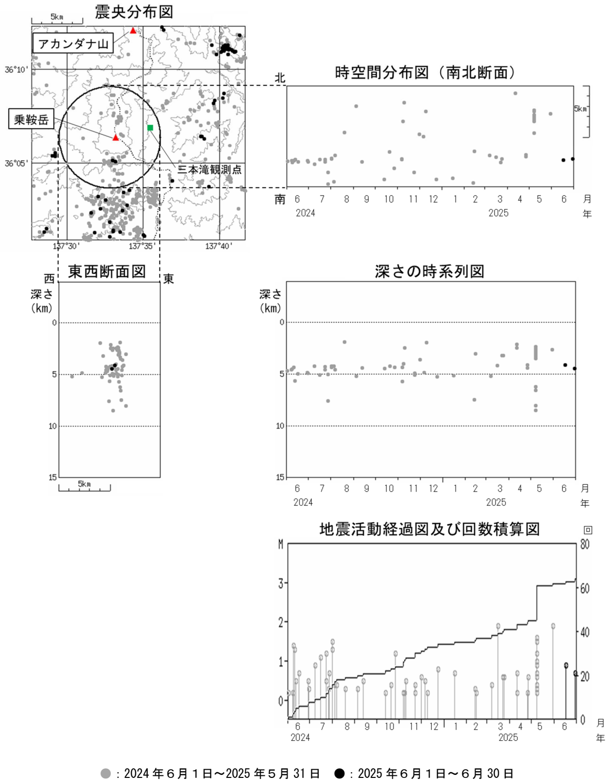
図3 乗鞍岳 広域地震観測網による山体・周辺の地震活動(2024年6月1日～2025年6月30日)
