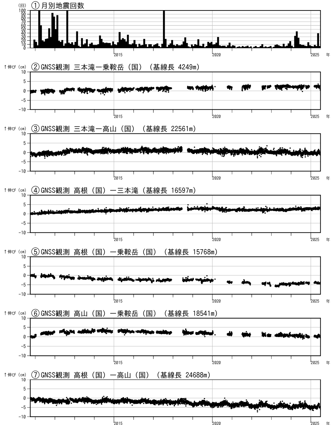
図 2 乗鞍岳 火山活動経過図 (2010 年 10 月 1 日～2025 年 6 月 30 日)
