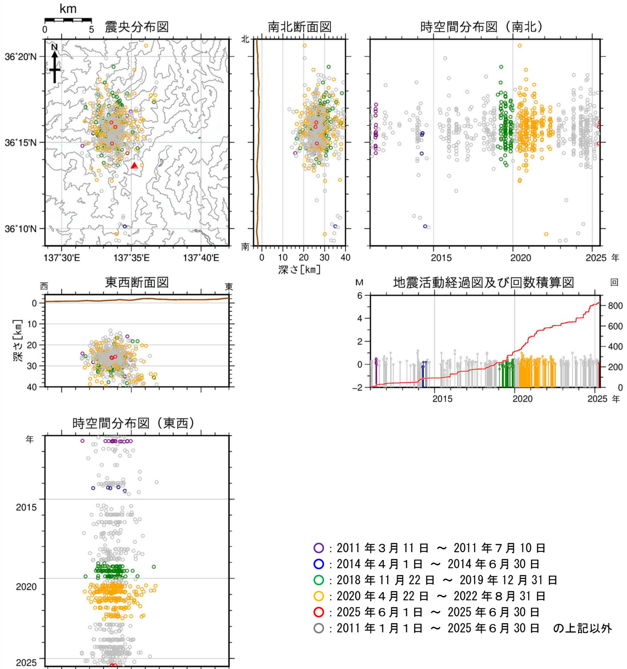
図10 焼岳 広域地震観測網による深部低周波地震の震源分布図（2011年1月1日～2025年6月30日）
