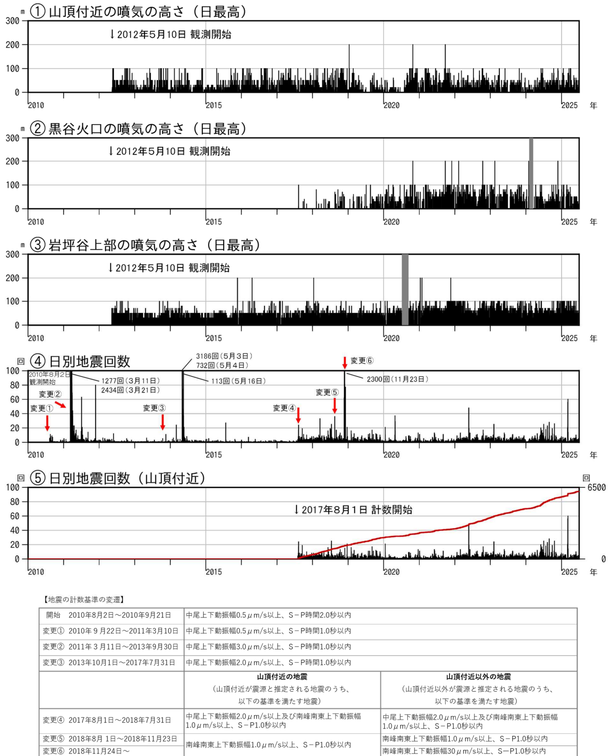
図5 焼岳 噴気の高さと地震回数の推移(2010年8月2日～2025年6月30日)
