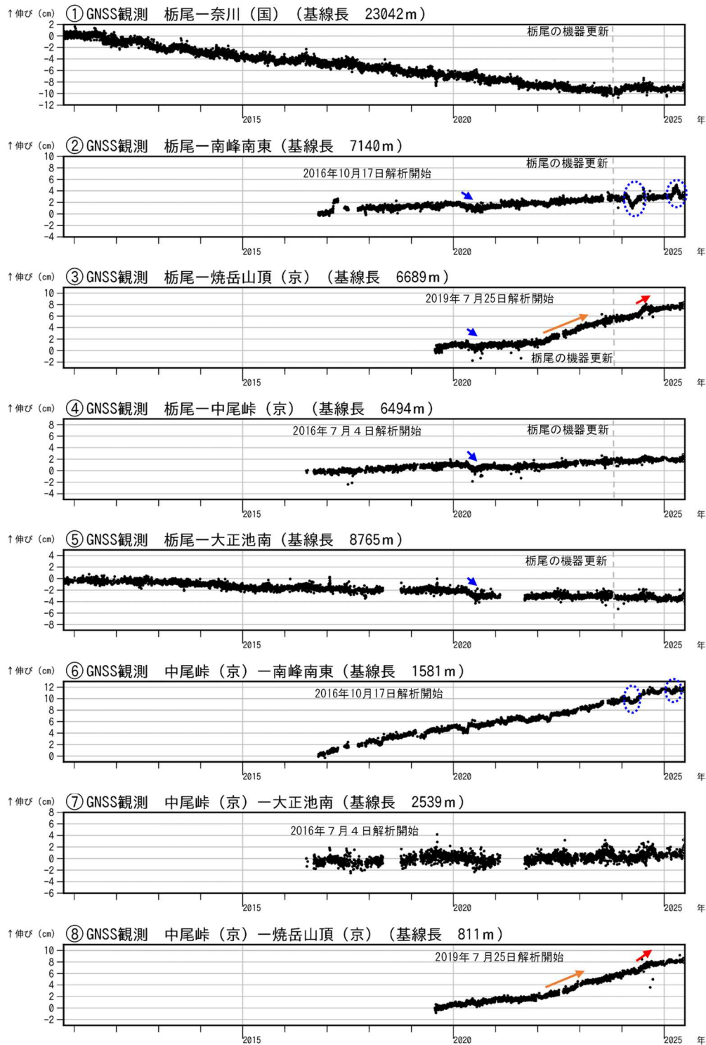
図6 焼岳 GNSS 連続観測による基線長変化（2010年10月1日～2025年6月30日）
