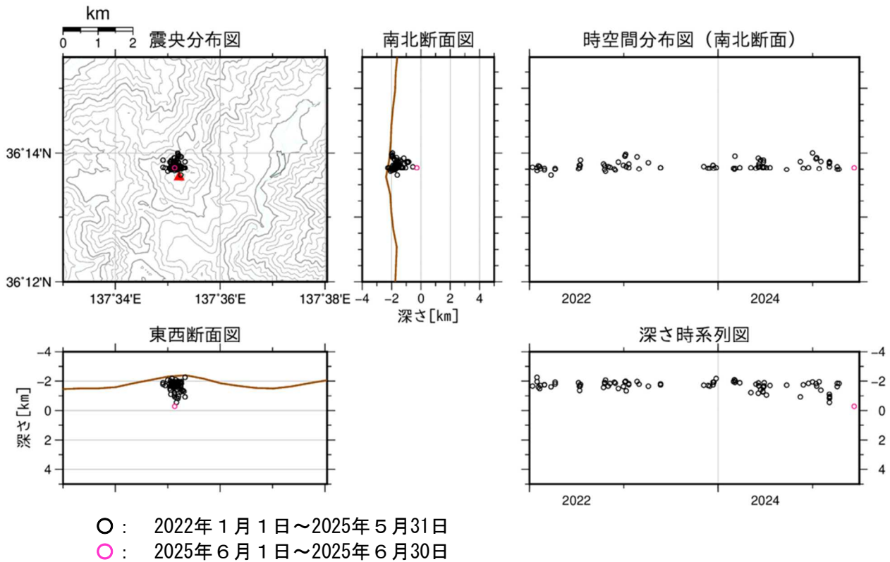
図2 焼岳 山頂付近の地震の震源分布図（2022年1月1日～2025年6月30日）
