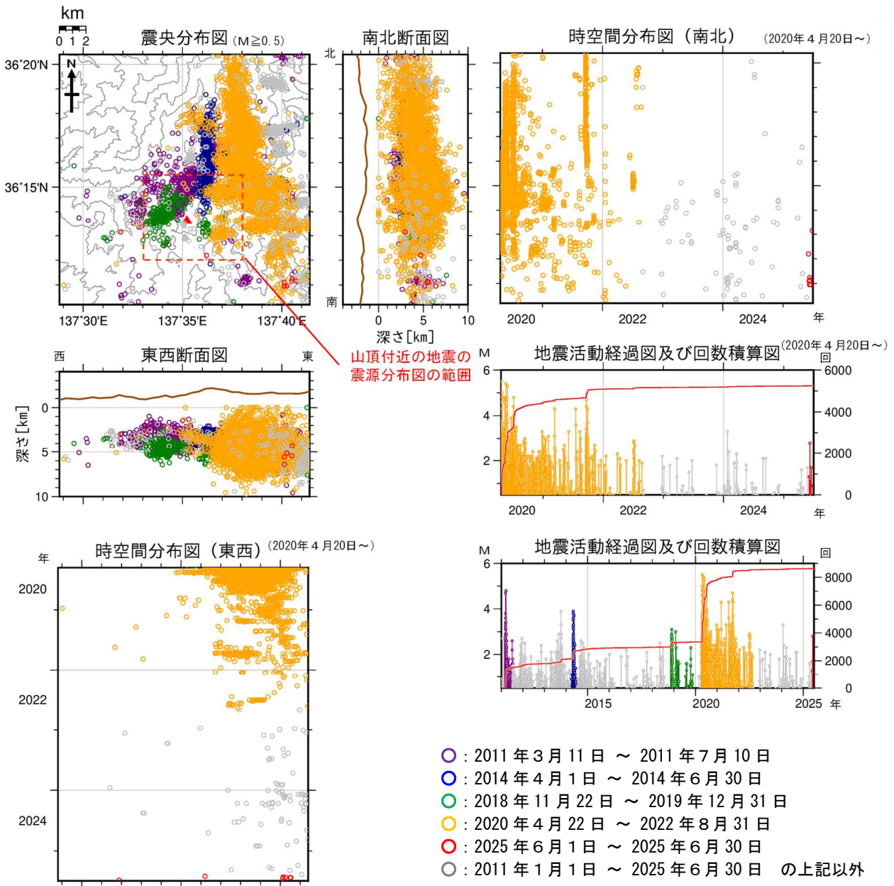
図9 焼岳 広域地震観測網による山体及び周辺の地震活動(2011年1月1日～2025年6月30日)
