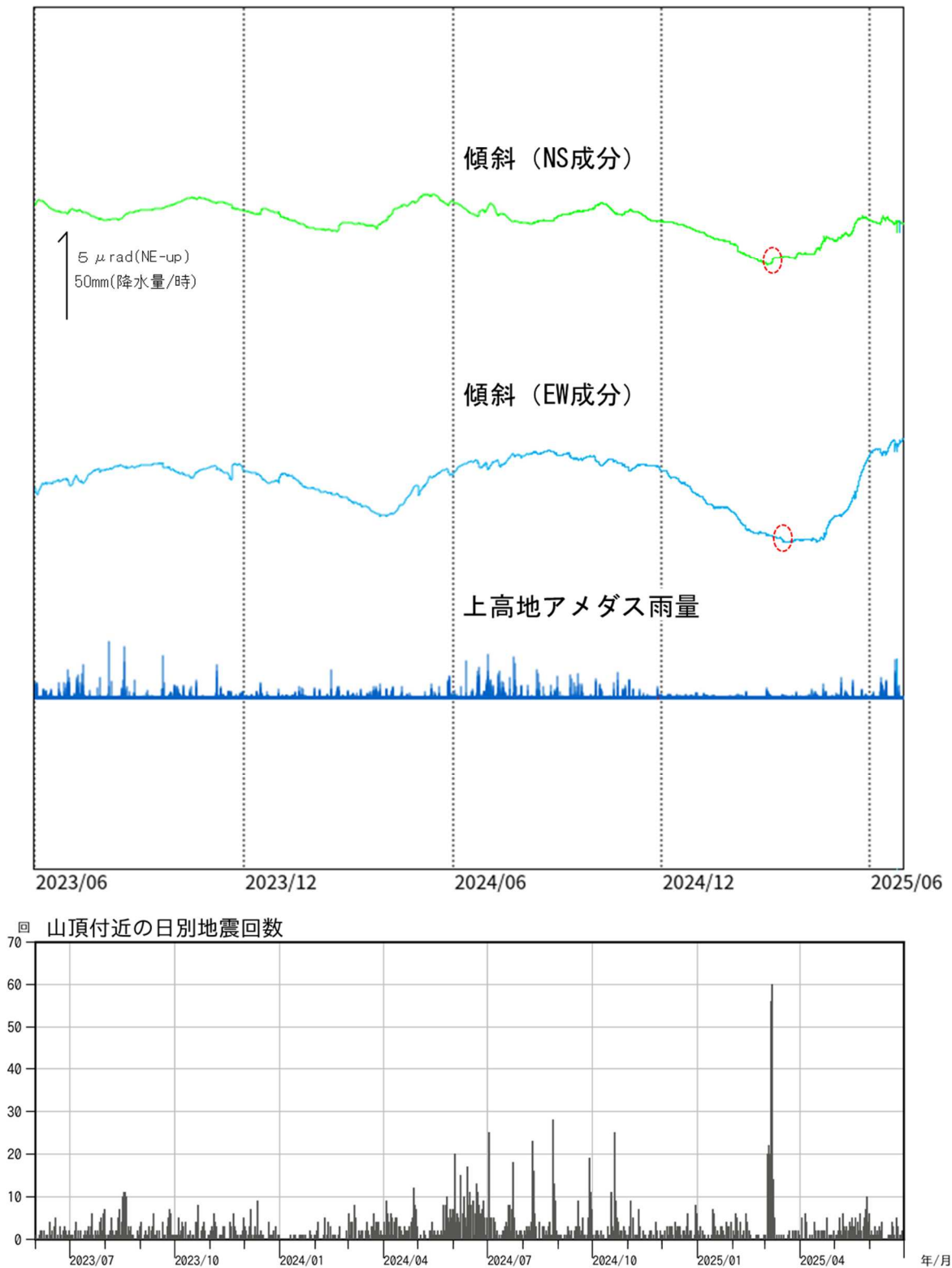
図8 焼岳 南峰南東観測点における傾斜データ（2023年6月1日～2025年6月30日）
