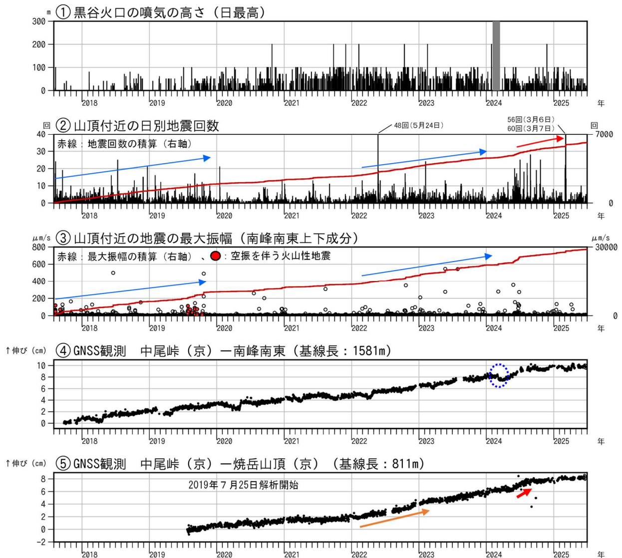
図1 焼岳 火山活動経過図（2017年8月1日～2025年6月30日）
