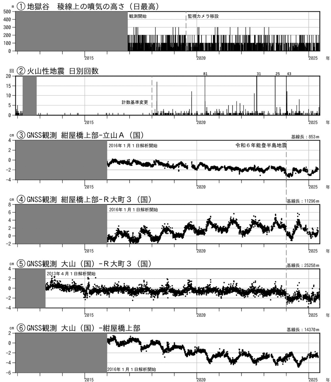
図3 弥陀ヶ原 火山活動経過図（2011年12月1日～2025年6月30日）
