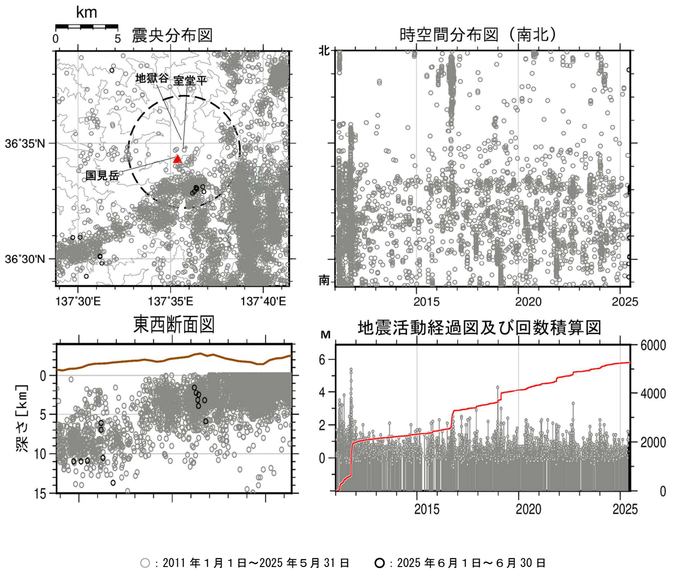
図2 弥陀ヶ原 広域地震観測網による山体・周辺の地震活動（2011年1月1日～2025年6月30日） 震央分布図中の円は弥陀ヶ原の計数対象地震（室堂平でS-P時間1秒以内）のおよその範囲を示しています。 広域地震観測網により震源決定したもので、深さは全て海面以下として決定しています。なお、2020年9月以降については、地震観測点の標高を考慮する等、震源決定の手法を変更しています。 図中の震源要素は一部暫定値が含まれており、後日変更することがあります。
