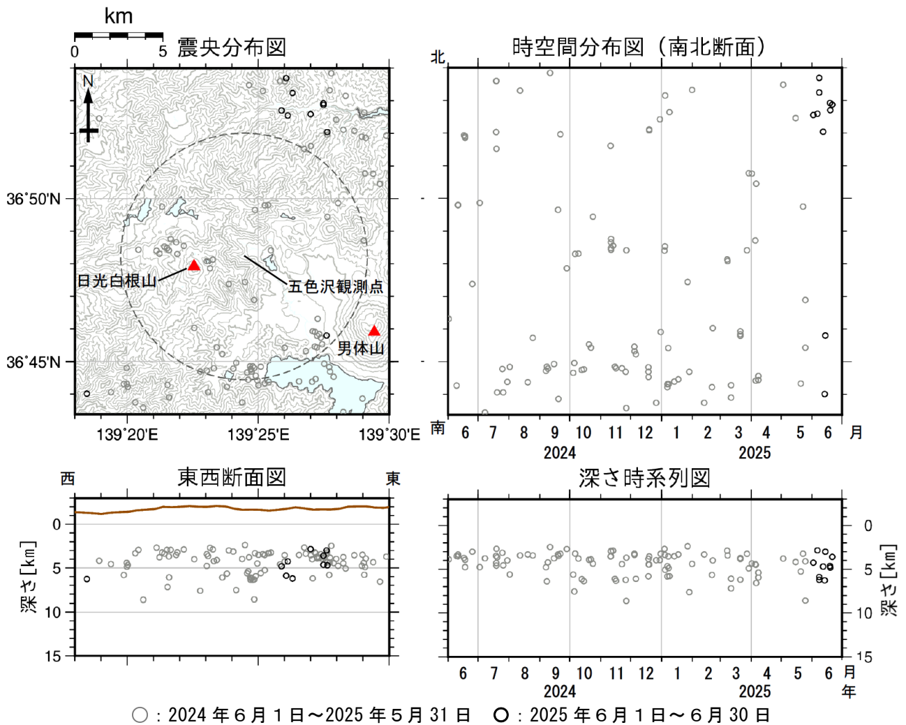
図3 日光白根山 広域地震観測網による山体周辺の地震活動 (2024 年 6 月 1 日～2025 年 6 月 30 日)
