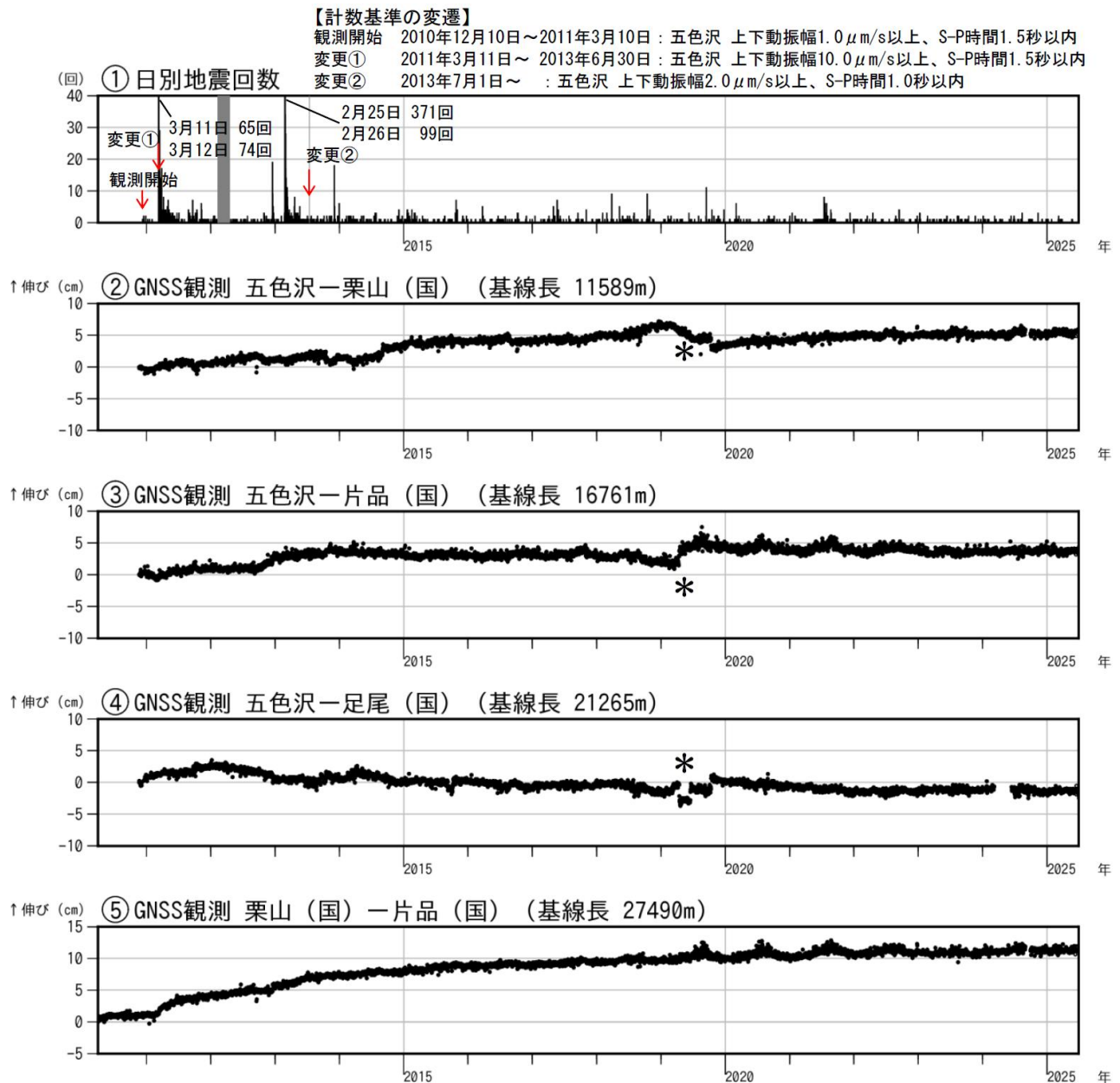
図2 日光白根山 火山活動経過図（2010年4月1日～2025年6月30日）
