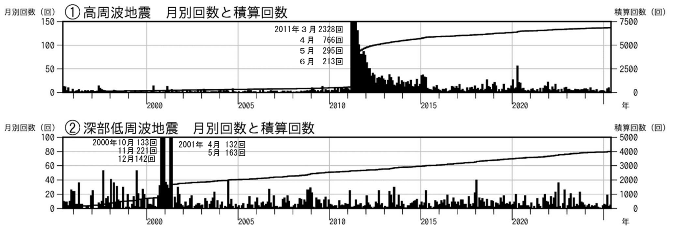
図2 富士山 月別地震回数（1995 年 6 月 1 日～2025 年 5 月 31 日）
