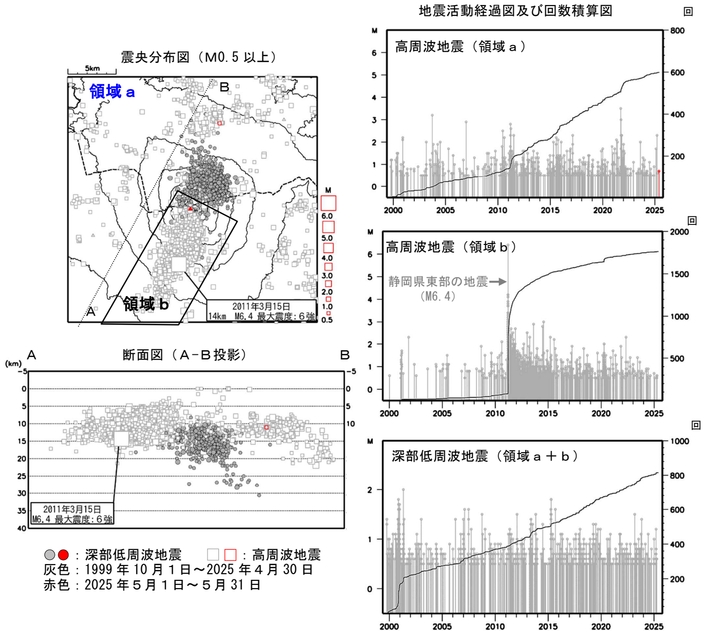
図 3 富士山 広域地震観測網による山体及び周辺の地震活動（1999年10月1日～2025年5月31日）
