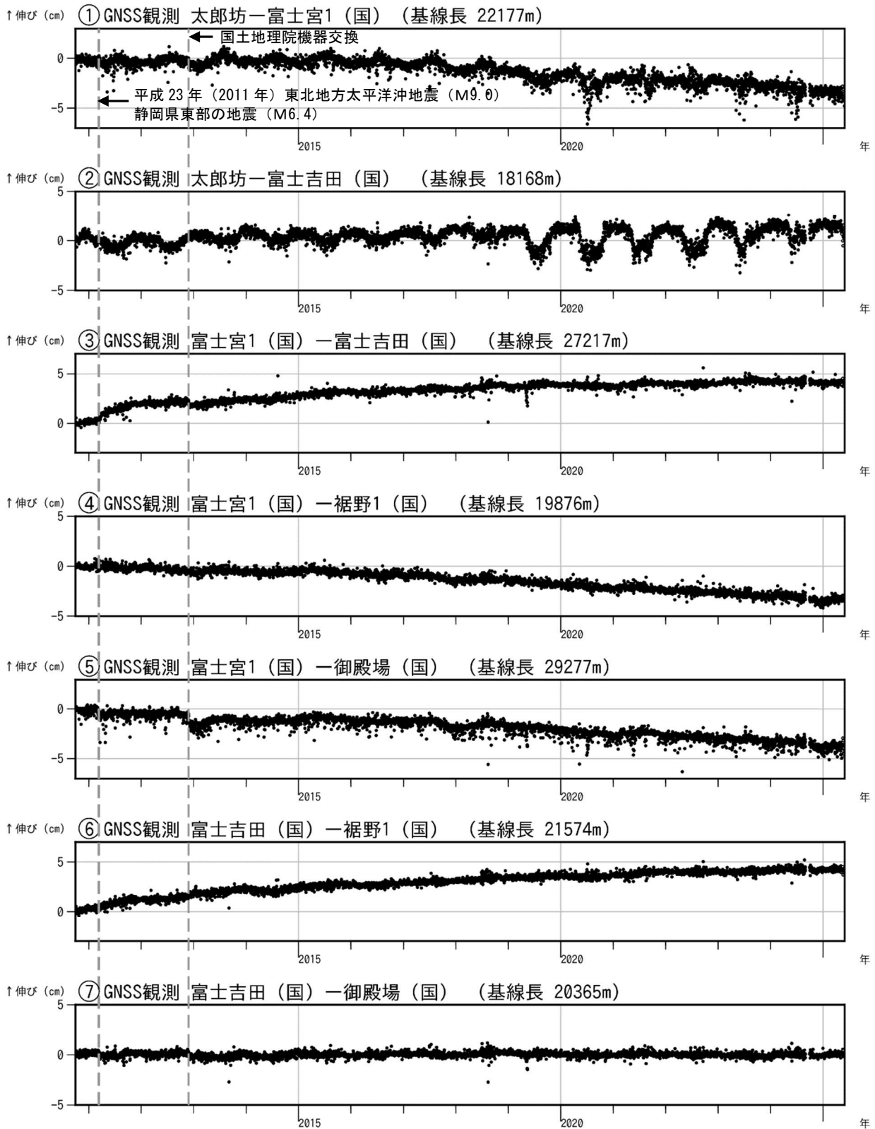
図4 富士山 GNSS 連続観測による基線長変化 (2010 年 10 月 1 日～2025 年 5 月 31 日)
