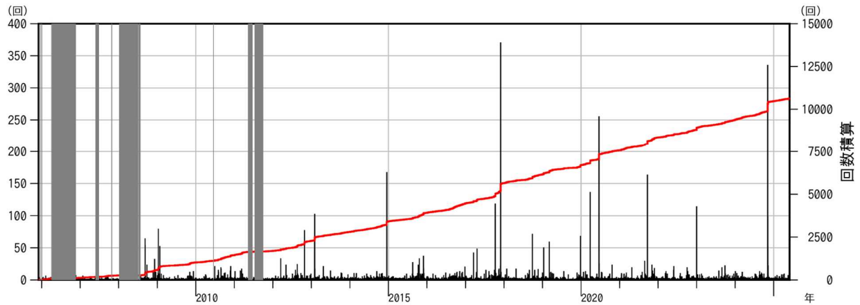
図 3 白山 日別地震回数と積算回数（2005 年 12 月 1 日～2025 年 5 月 31 日）
