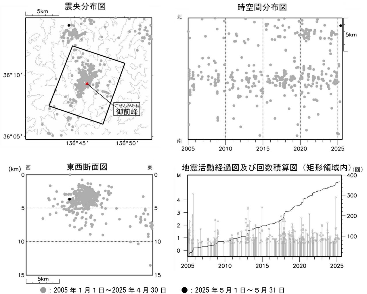
図 4 白山 広域地震観測網による山体・周辺の地震活動（2005 年 1 月 1 日～2025 年 5 月 31 日）
