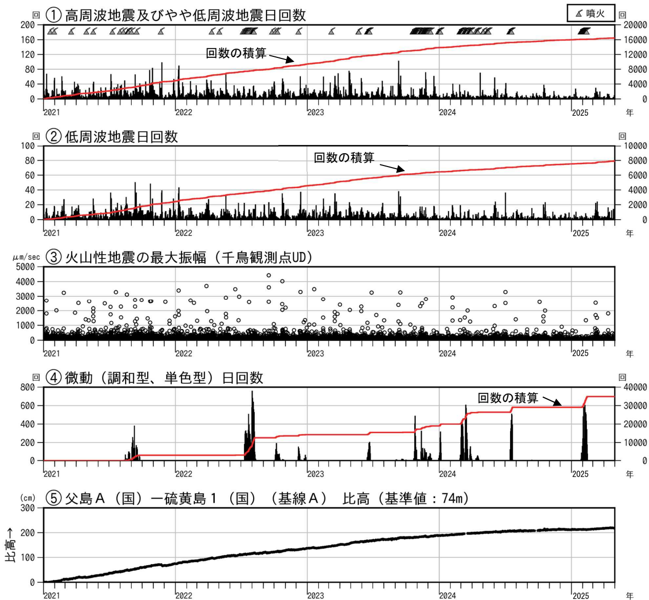
図5 硫黄島 火山活動経過図（2021年1月1日～2025年4月30日）
