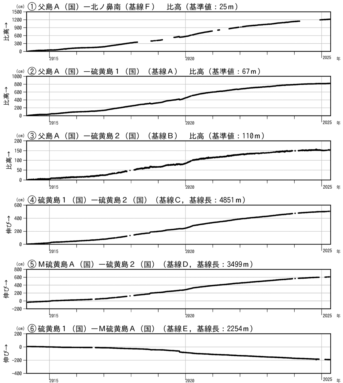
図6 硫黄島 GNSS 連続観測結果（2014年3月1日～2025年4月30日）
