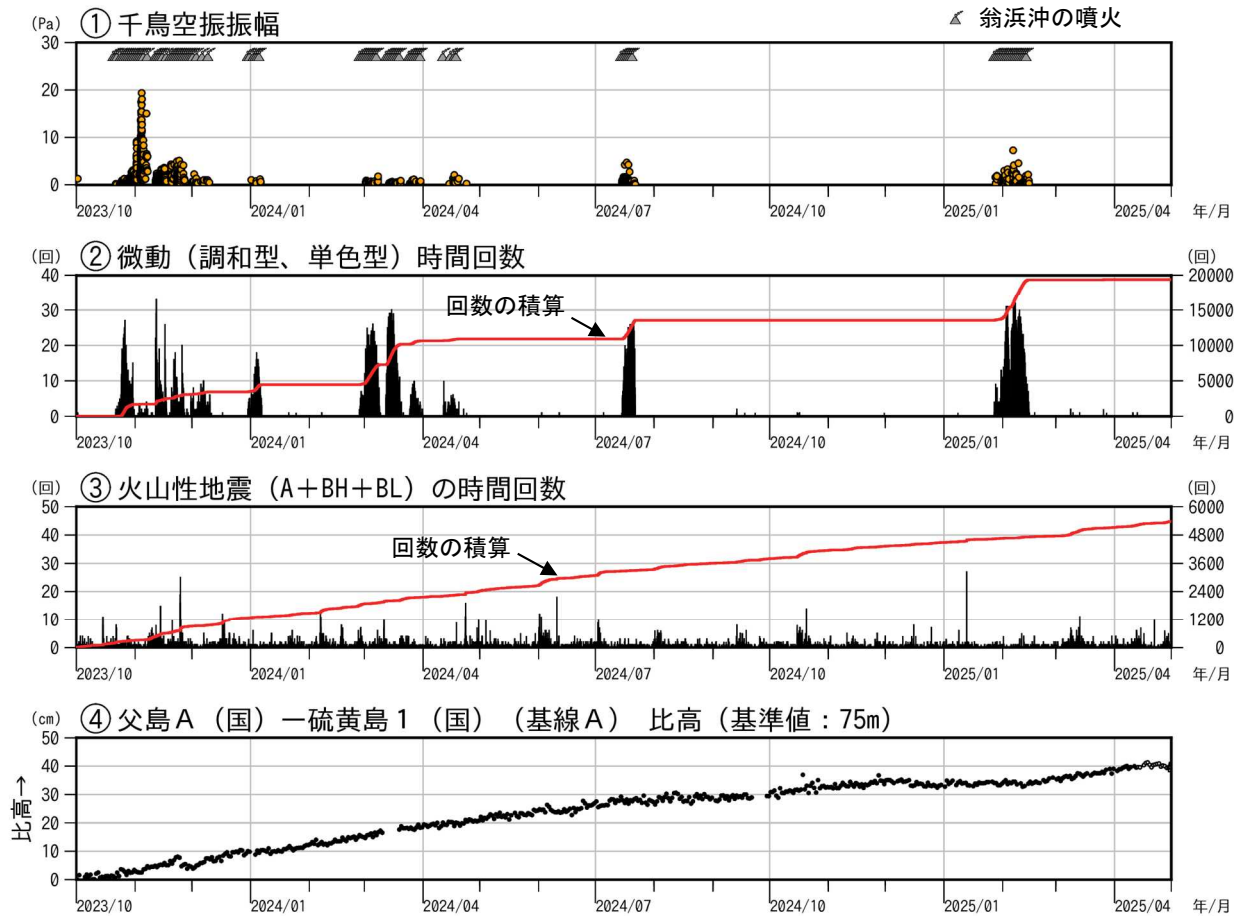
図4 硫黄島 火山活動経過図（2023年10月1日～2025年4月30日）
