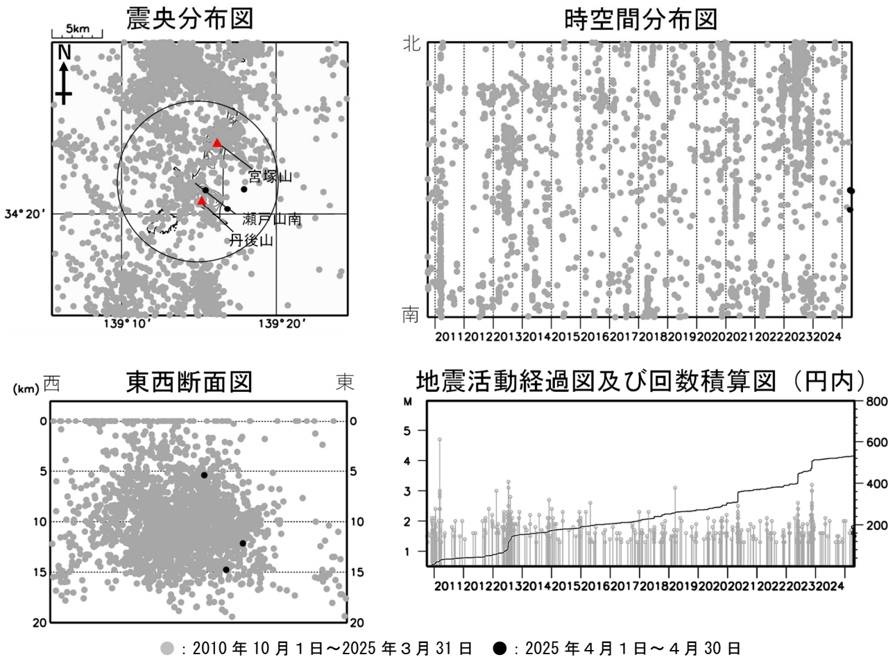
図 3 新島 広域地震観測網による山体・周辺の地震活動（2010 年 10 月 1 日～2025 年 4 月 30 日） 広域地震観測網により震源決定したもので、深さは全て海面以下として決定しています。なお、2020 年 9 月以降については、地震観測点の標高を考慮する等、震源決定の手法を変更しています。 M（マグニチュード）は地震の規模を表し、M1.3 以上の地震を示しています。 図中の震源要素は一部暫定値が含まれており、後日変更することがあります。 計数対象（瀬戸山南から半径約 8 km、深さ約 20km 以内）以外の地震が含まれるため、図 2－①の日別地震回数（高周波地震）とは異なります。 震央分布図中の円は火山性地震の回数の計数対象（瀬戸山南から半径 8 km、深さ 20km 以内）の範囲を示しています。 ・地震活動は低調に経過しました。
