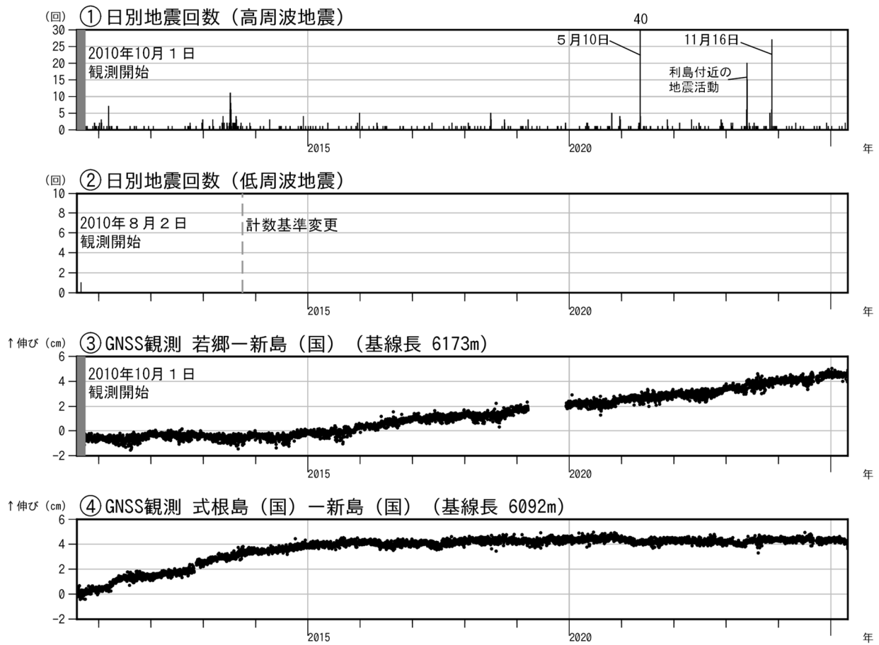
図2 新島 火山活動経過図(2010年8月2日～2025年4月30日)
