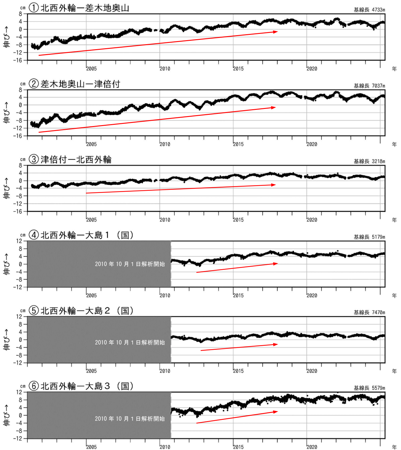
図3-1 伊豆大島 GNSS 連続観測による基線長変化(2001年1月～2025年4月30日)
