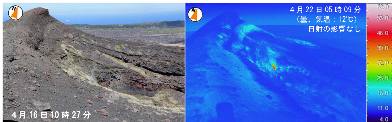
図7-1 伊豆大島 B2 火孔周辺の状況（撮影方向は図8参照）
