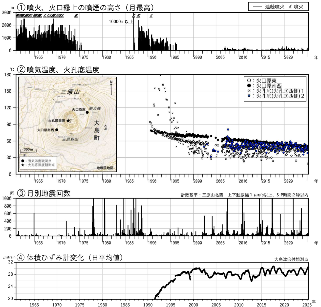
図1 伊豆大島 長期間の火山活動経過図（1961年1月～2025年4月30日）
