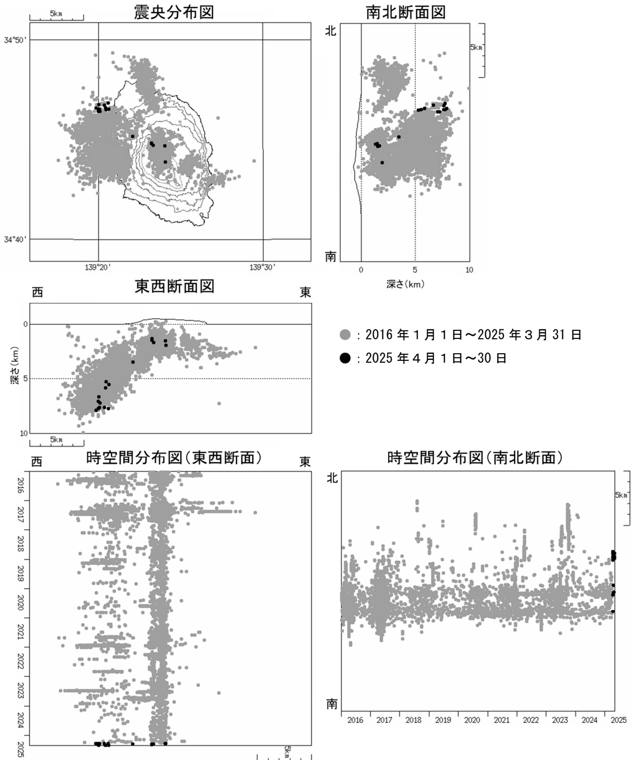
図 4 伊豆大島 震源分布図（2016 年 1 月 1 日～2025 年 4 月 30 日）
