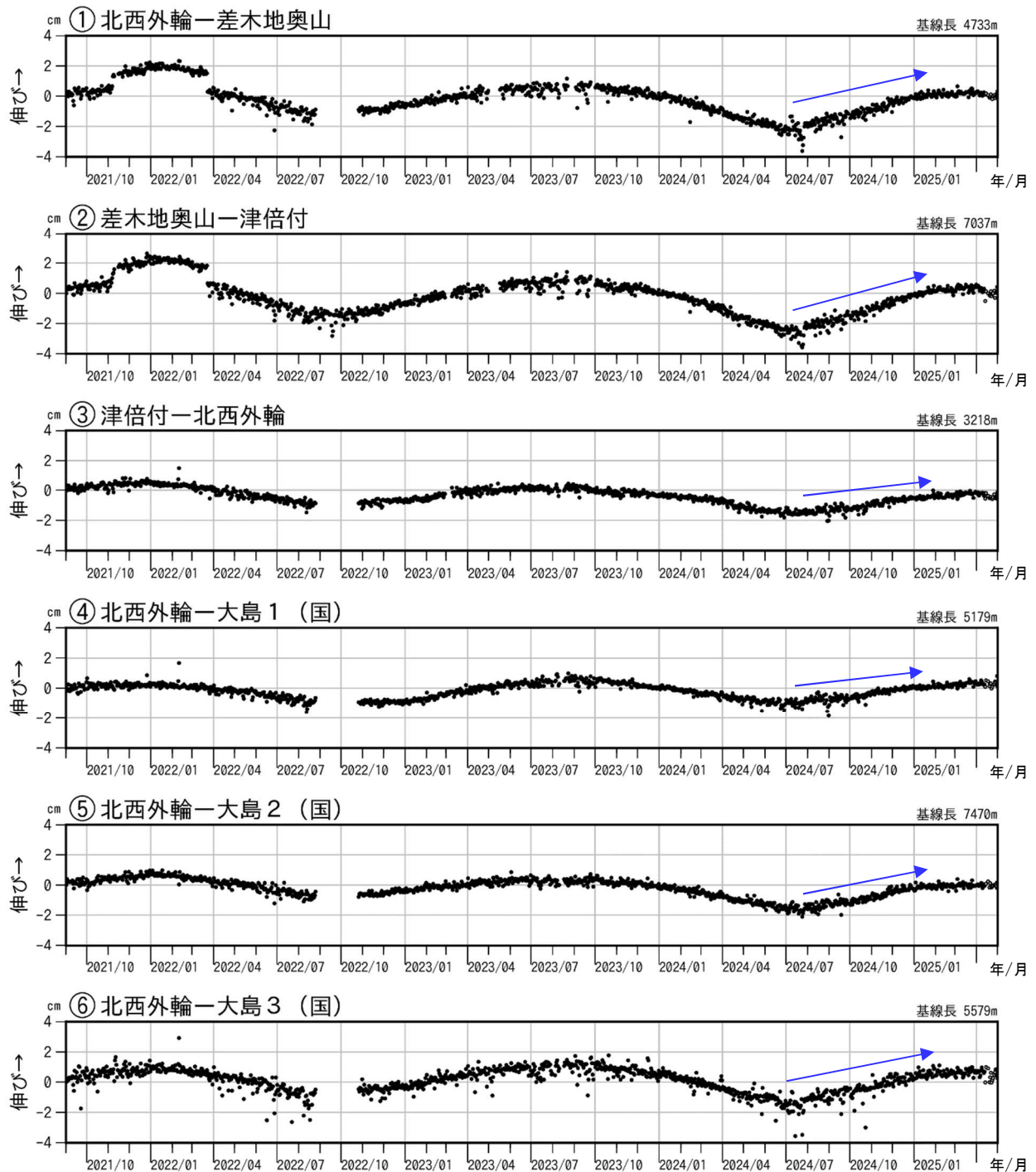
図 3-2 伊豆大島 GNSS 連続観測による基線長変化(2021 年 9 月～2025 年 4 月 30 日)
