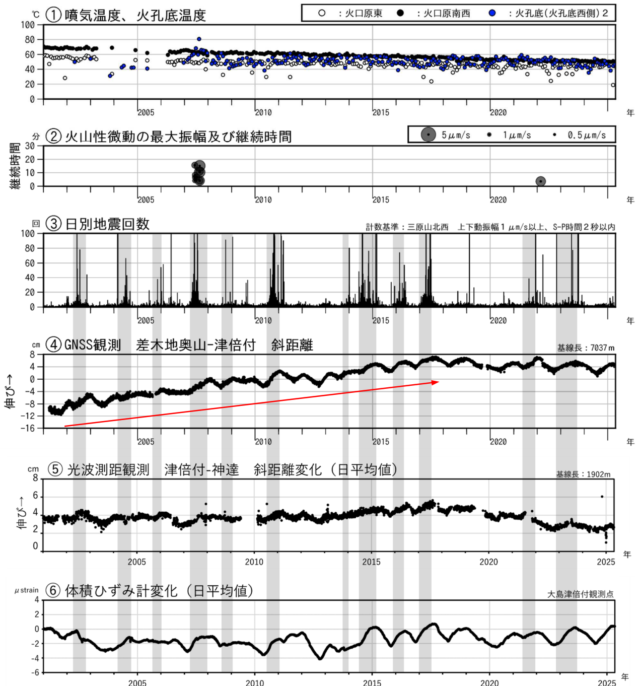
図2 伊豆大島 最近の火山活動経過図（2001年1月～2025年4月30日）
