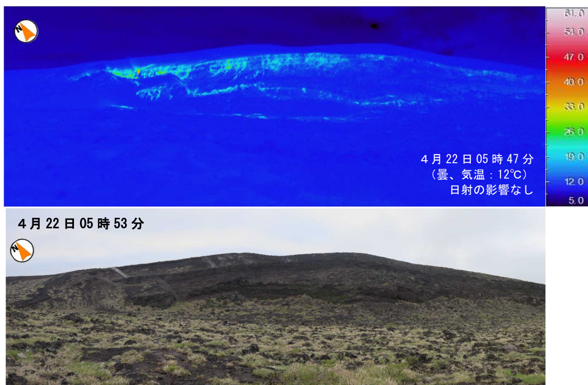
図7-2 伊豆大島 剣ガ峰の状況（撮影方向は図8参照）
