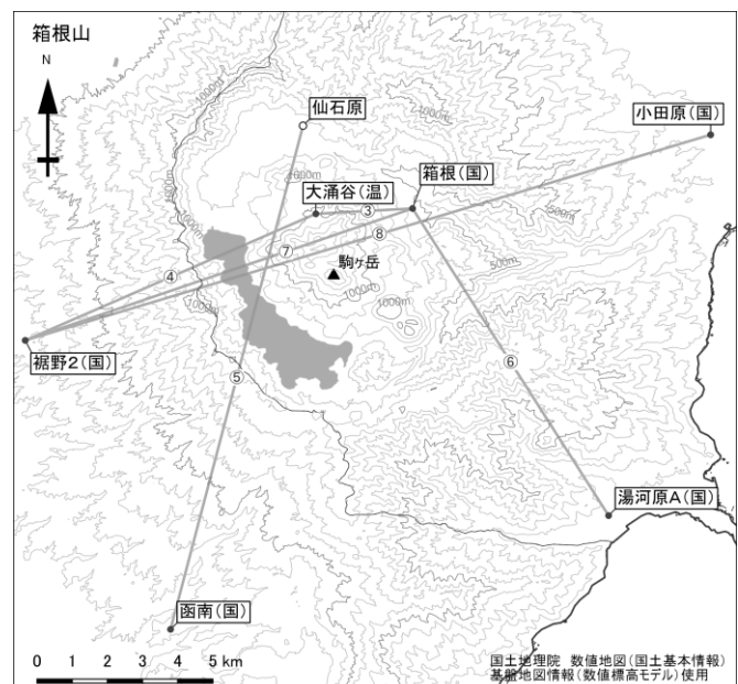
図3-2 箱根山 GNSS連続観測による 基線長変化及び観測点配置図 (2012年1月1日～2025年4月30日)
