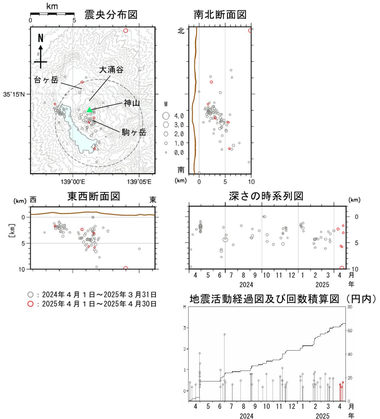
図4 箱根山 広域地震観測網による山体周辺の震源分布図（2024年4月1日～2025年4月30日）
