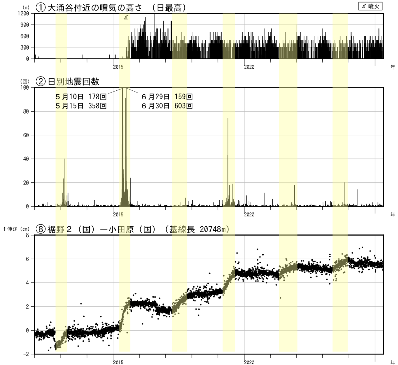
図3-1 箱根山 火山活動経過図（2012年1月1日～2025年4月30日）
