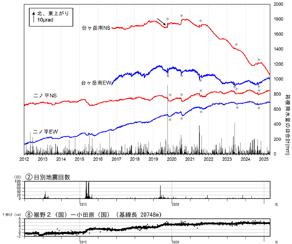
図5 箱根山 傾斜観測及び地震回数・GNSS観測（2012年1月1日～2025年4月30日）
