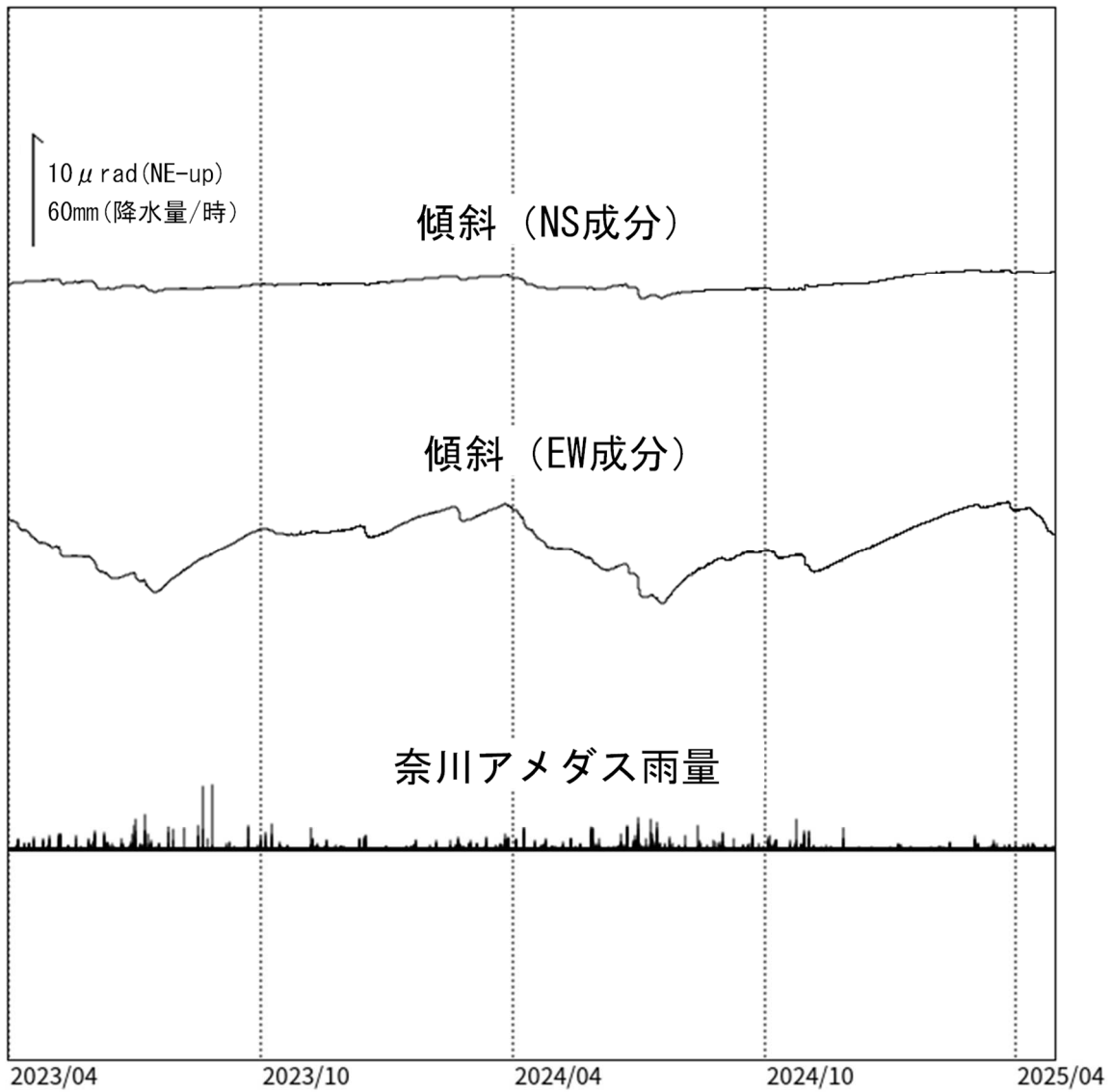
図4 乗鞍岳 三本滝観測点における傾斜データ（2023年4月1日～2025年4月30日） ・傾斜計による観測では、火山活動によるとみられる変動は認められません。
