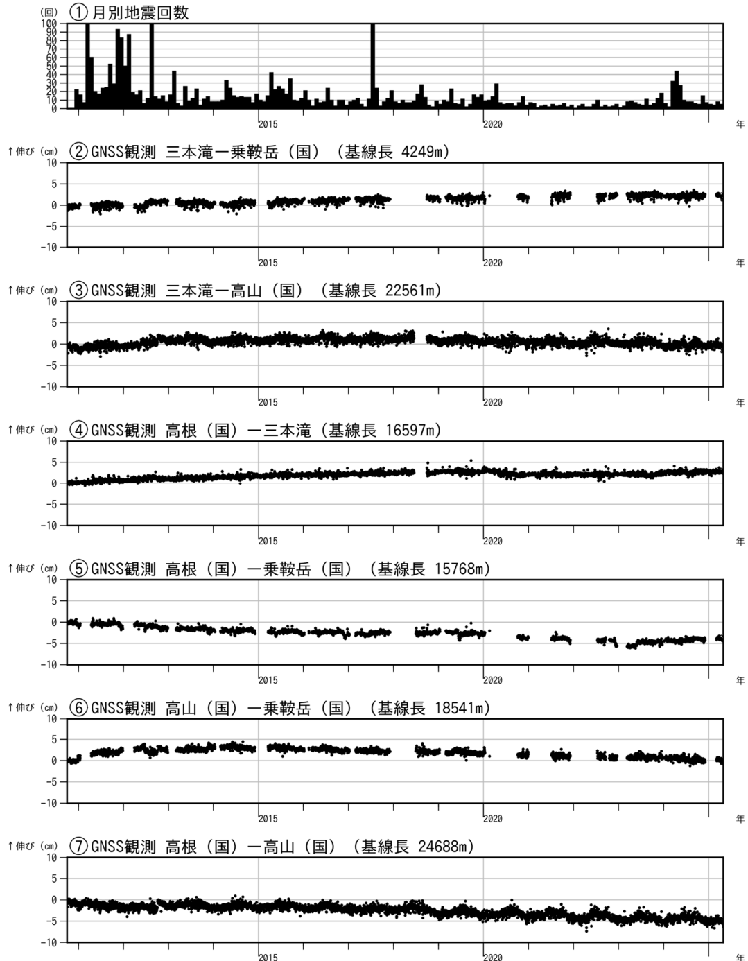
図2 乗鞍岳 火山活動経過図（2010年10月1日～2025年4月30日）
