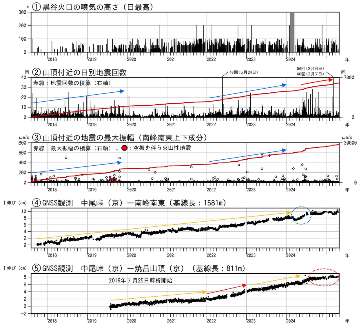
図1 焼岳 火山活動経過図（2017年8月1日～2025年4月30日）
