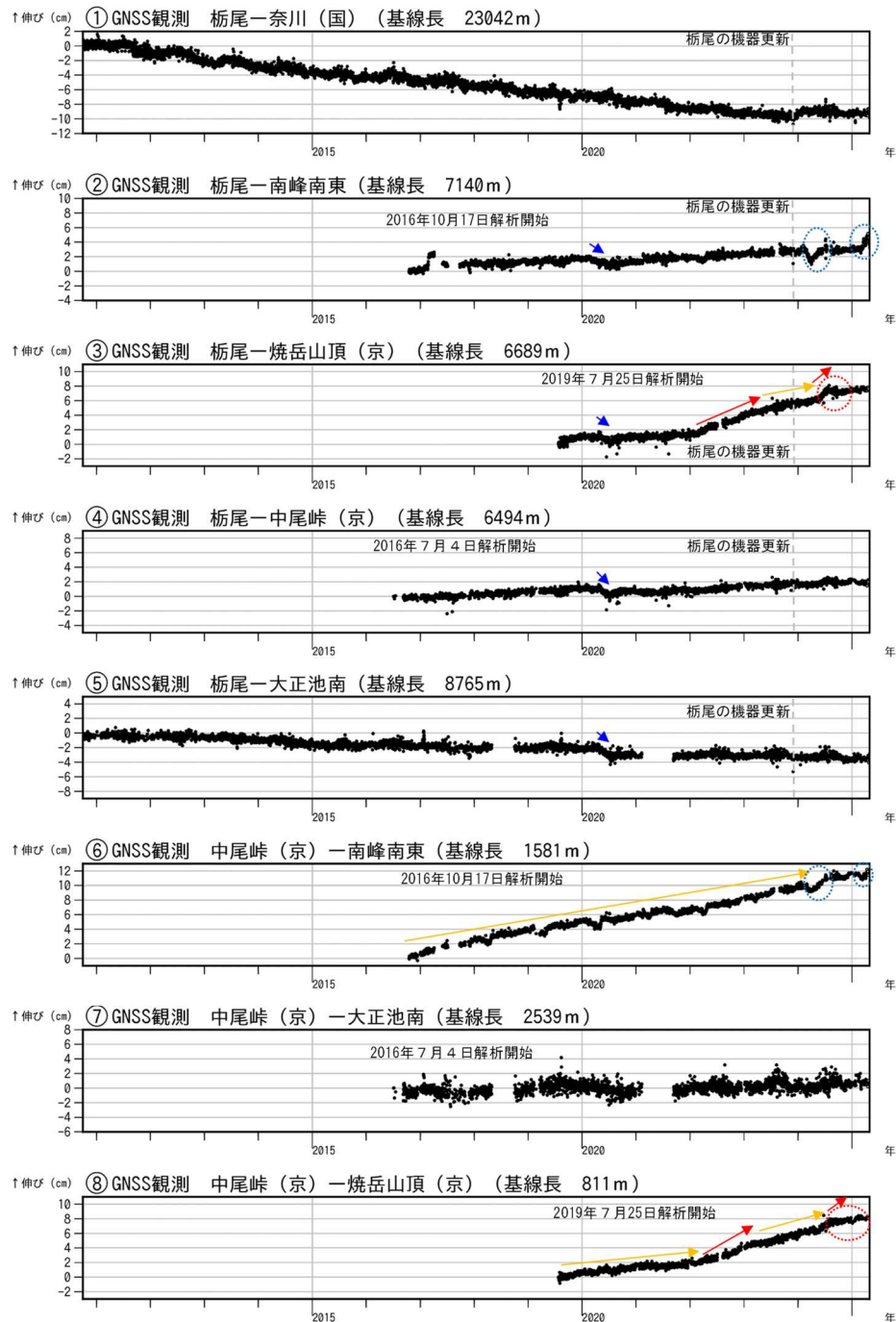
図6 焼岳 GNSS 連続観測による基線長変化（2010年10月1日～2025年4月30日）
