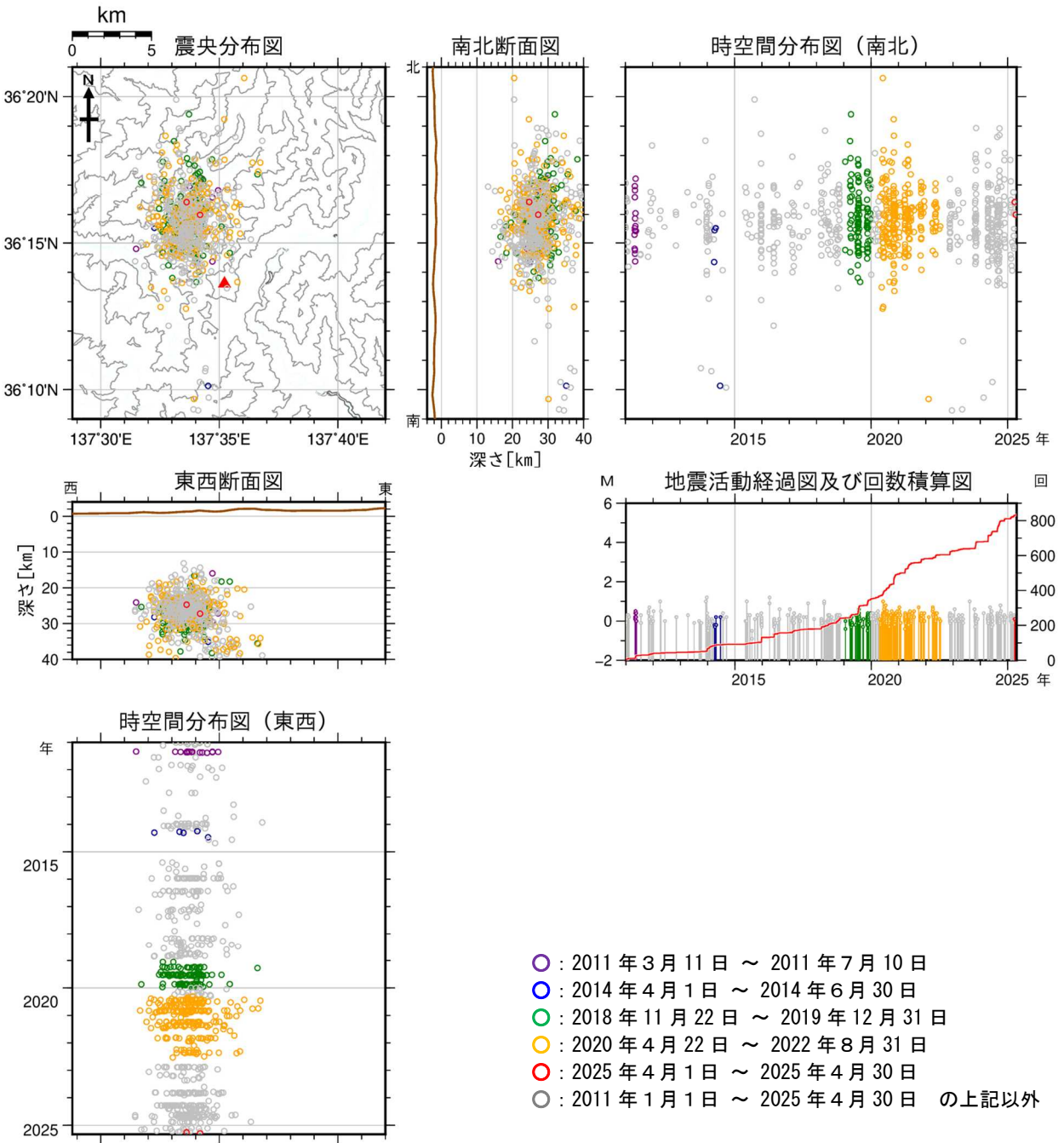
図10 焼岳 広域地震観測網による深部低周波地震の震源分布図（2011年1月1日～2025年4月30日）
