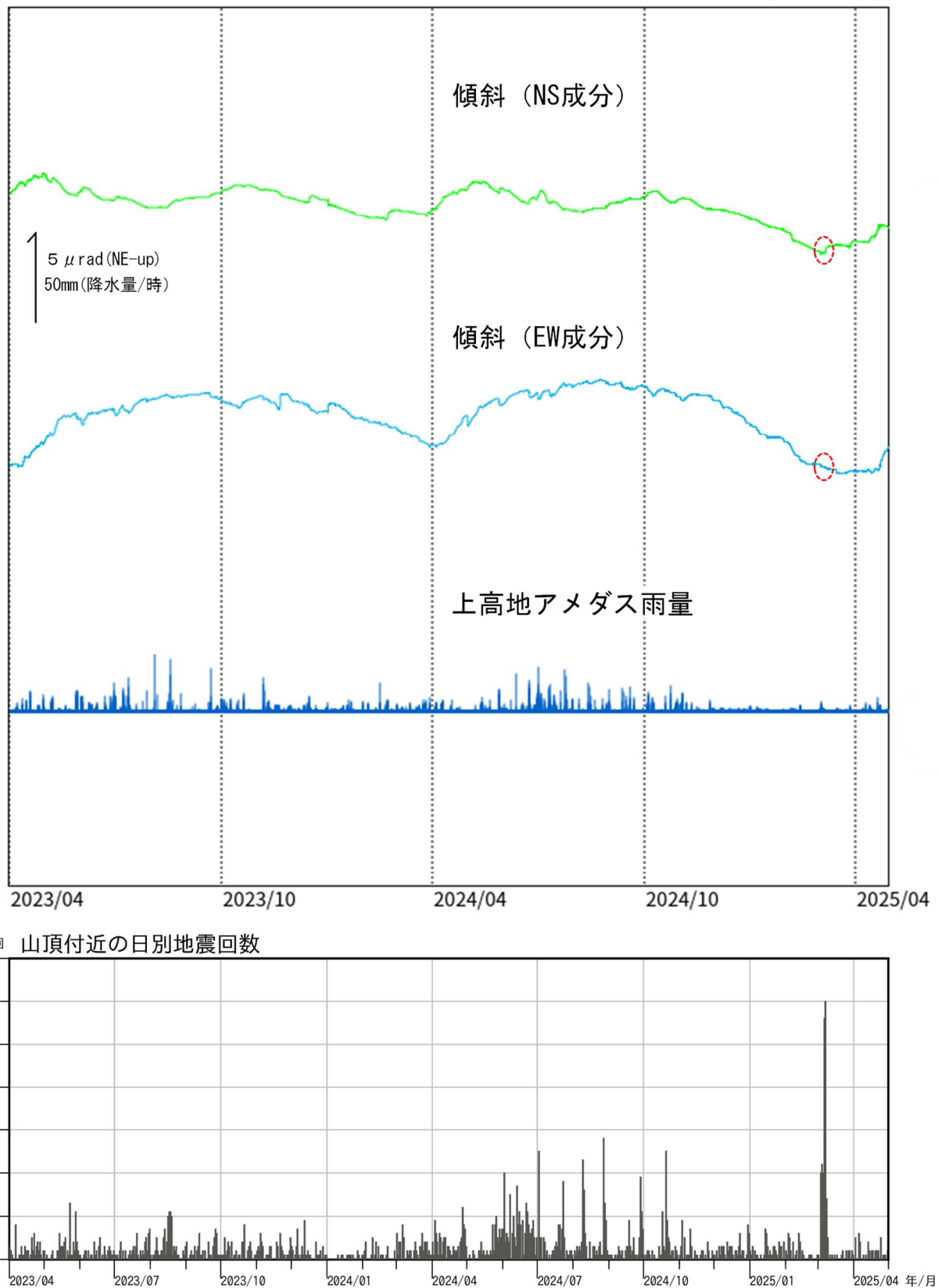
図8 焼岳 南峰南東観測点における傾斜データ（2023年4月1日～2025年4月30日） ・傾斜計による観測では、3月8日に発生した山頂方向の隆起を示すわずかな傾斜変動（赤破線）以外は、火山活動によるとみられる変動は認められません。
