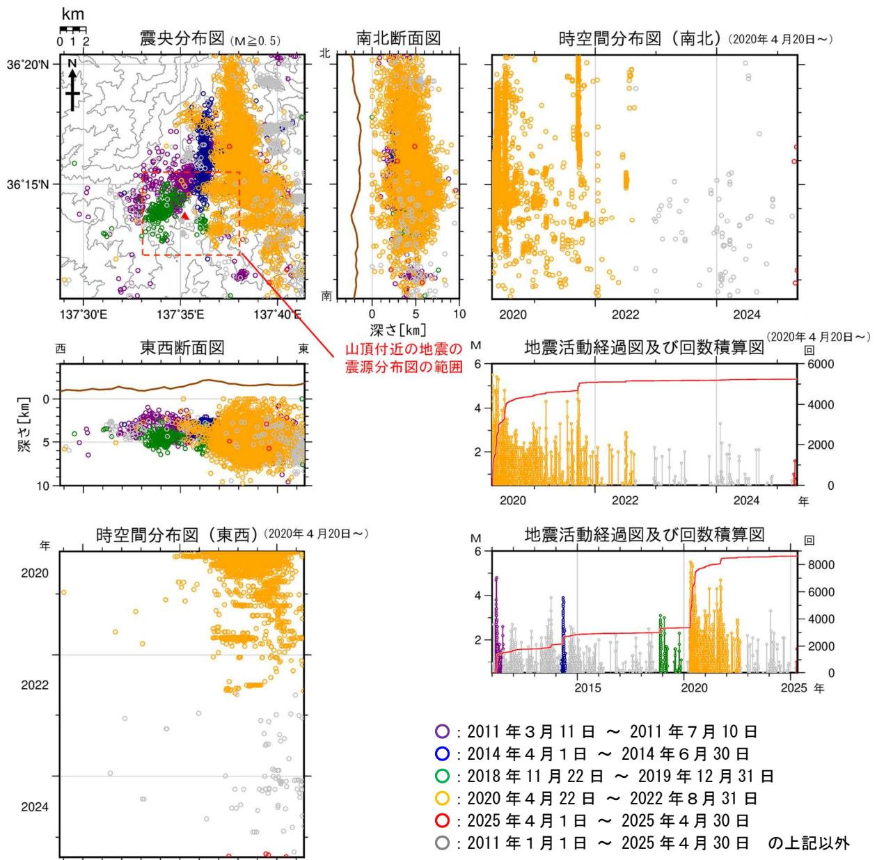
図9 焼岳 広域地震観測網による山体及び周辺の地震活動(2011年1月1日～2025年4月30日)
