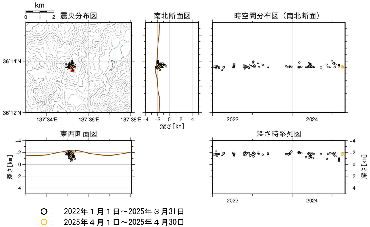
図2 焼岳 山頂付近の地震の震源分布図（2022年1月1日～2025年4月30日）
