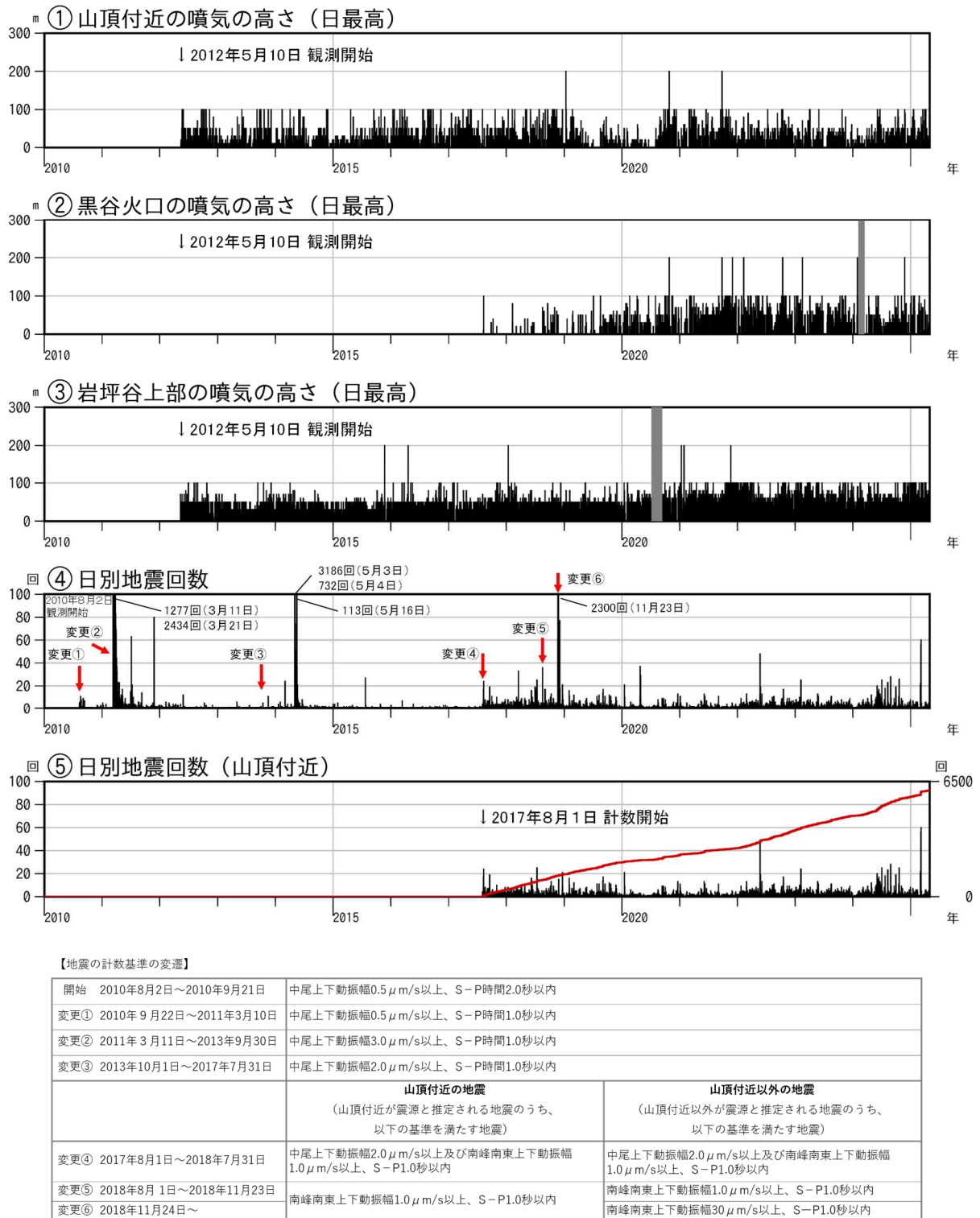
図5 焼岳 噴気の高さと地震回数の推移(2010年8月2日～2025年4月30日)
