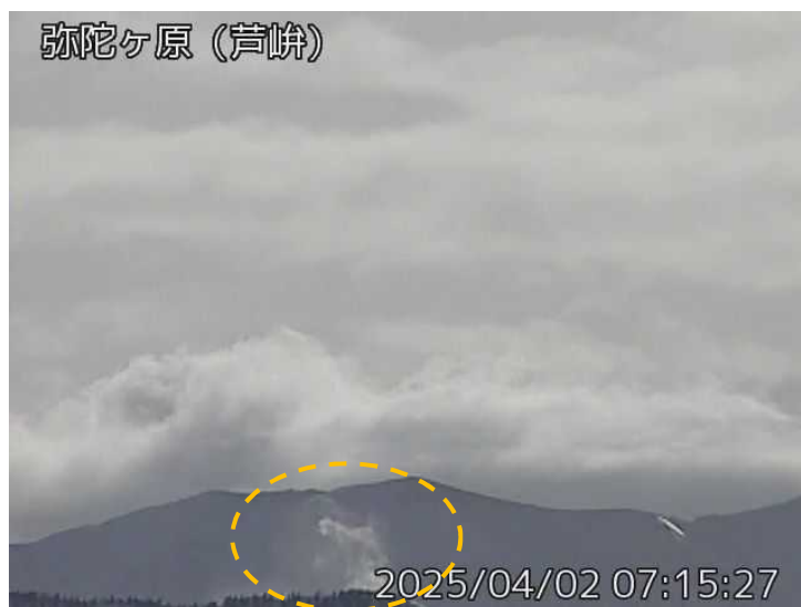
図1 弥陀ヶ原 地獄谷からの噴気の状況（橙丸）（4月2日、芦峠監視カメラによる）
