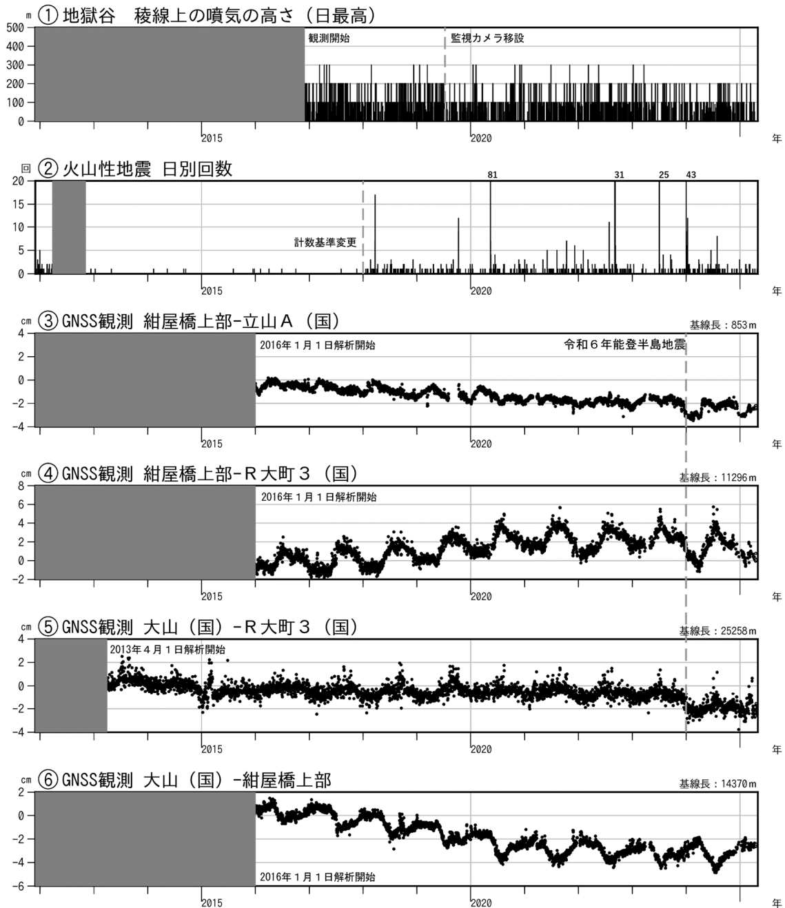
図3 弥陀ヶ原 火山活動経過図（2011年12月1日～2025年4月30日）
