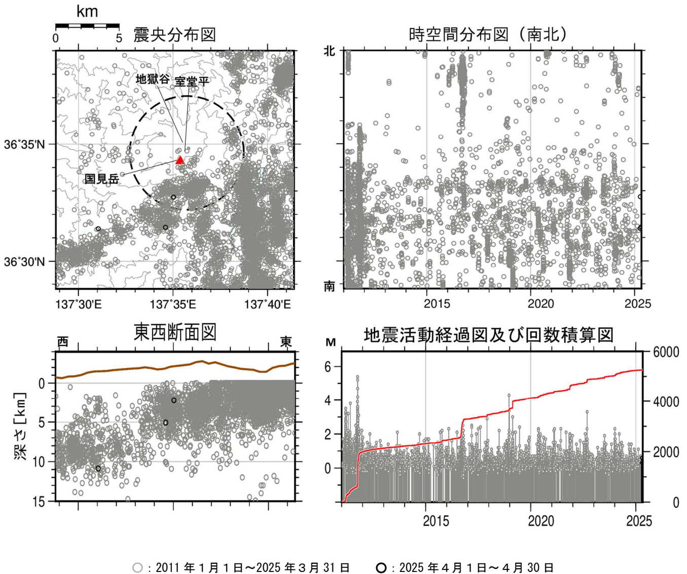
図 2 弥陀ヶ原 広域地震観測網による山体・周辺の地震活動（2011 年 1 月 1 日～2025 年 4 月 30 日） 震央分布図中の円は弥陀ヶ原の計数対象地震（室堂平で S-P 時間 1 秒以内）のおよその範囲を示しています。 広域地震観測網により震源決定したもので、深さは全て海面以下として決定しています。なお、2020 年 9 月以降については、地震観測点の標高を考慮する等、震源決定の手法を変更しています。 図中の震源要素は一部暫定値が含まれており、後日変更することがあります。
