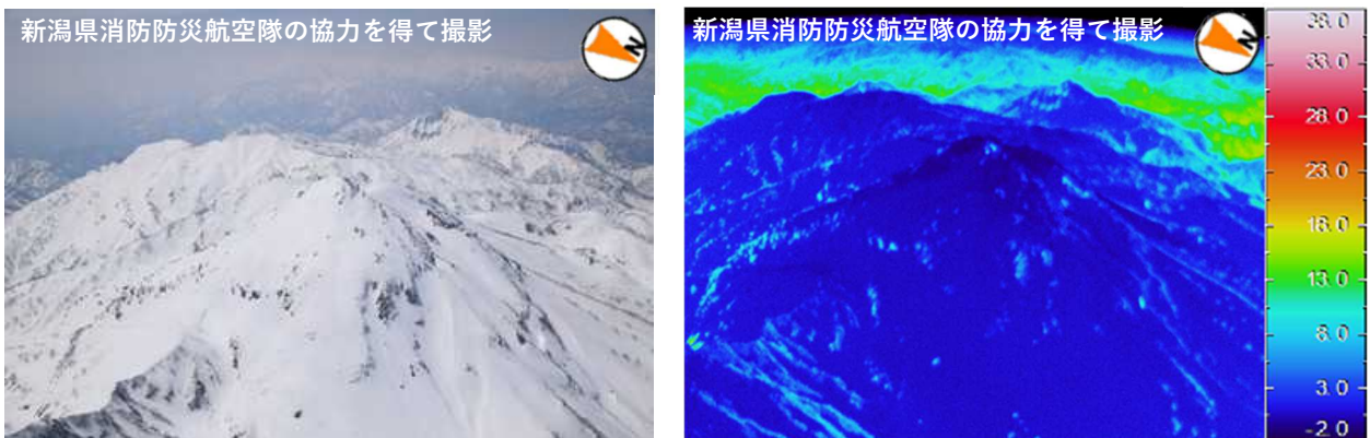
④東斜面 2025年4月17日 11:27（可視） 11:27（赤外） 高度約2,900m
