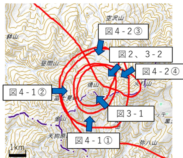
図5 新潟焼山 図2、図3及び図4の撮影位置と撮影方向
