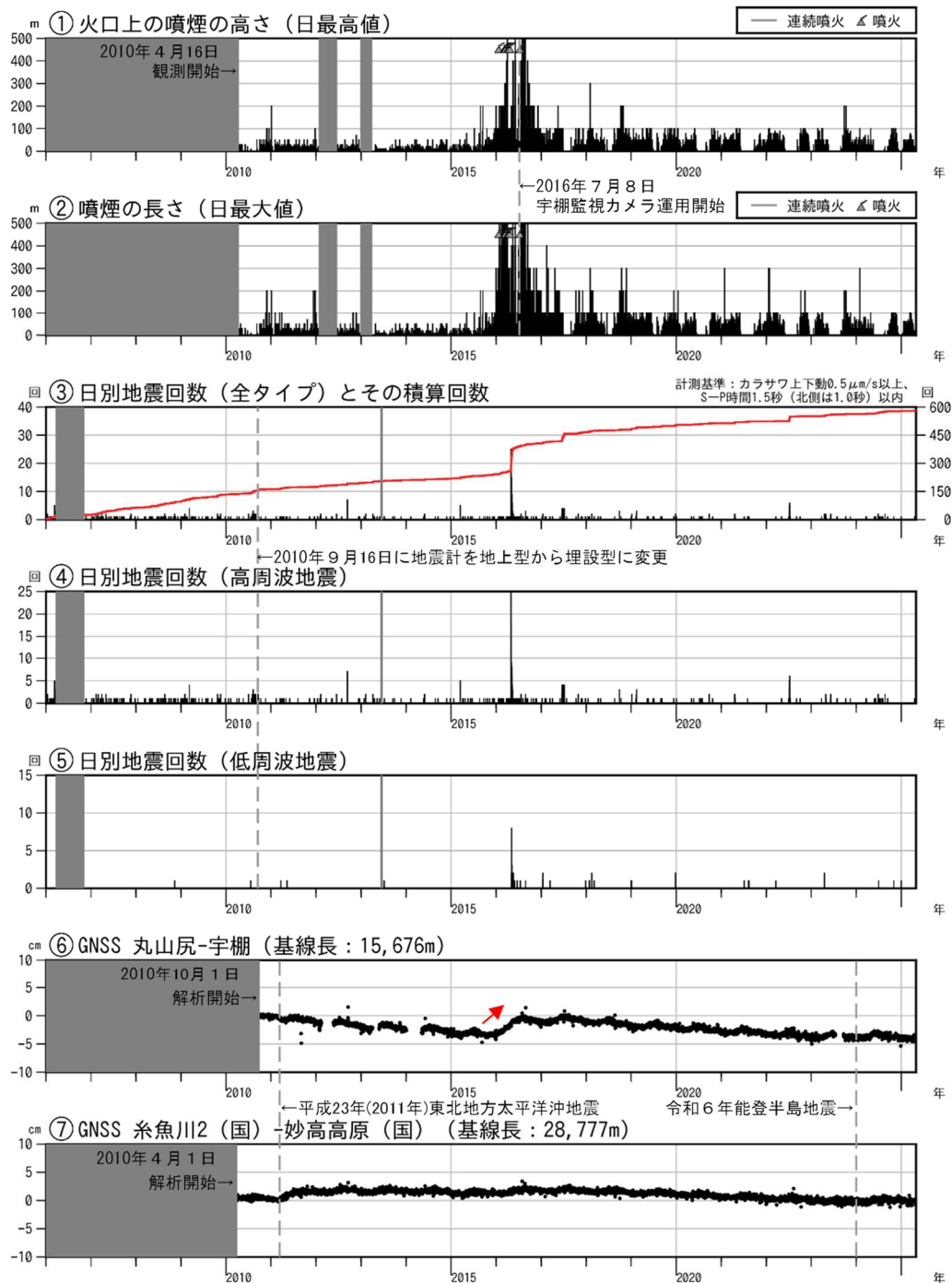
図6 新潟焼山 火山活動経過図（2006年1月1日～2025年4月30日）
