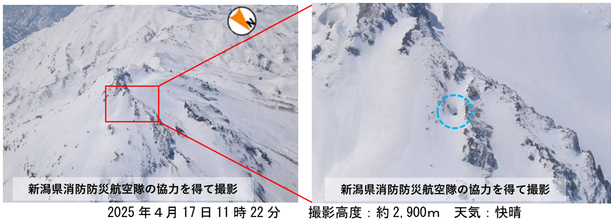
図 3－2 新潟焼山 北東斜面（北北東側噴気孔群）の状況
