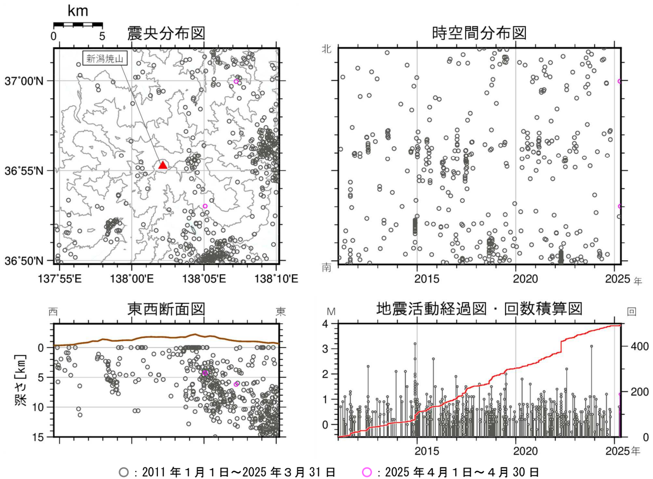
図 8 新潟焼山 広域地震観測網による山体・周辺の地震活動（2011 年 1 月 1 日～2025 年 4 月 30 日）
