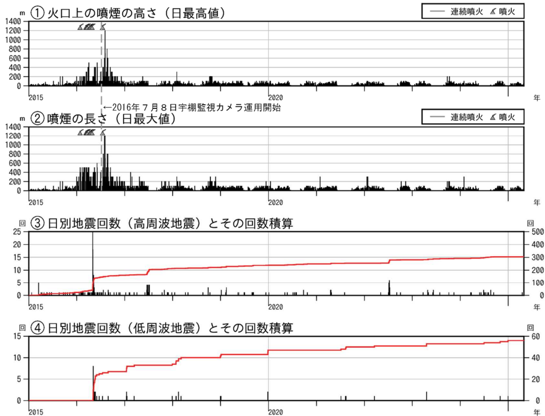
図 7 新潟焼山 火山活動経過図（短期）（2015 年 1 月 1 日～2025 年 4 月 30 日）
