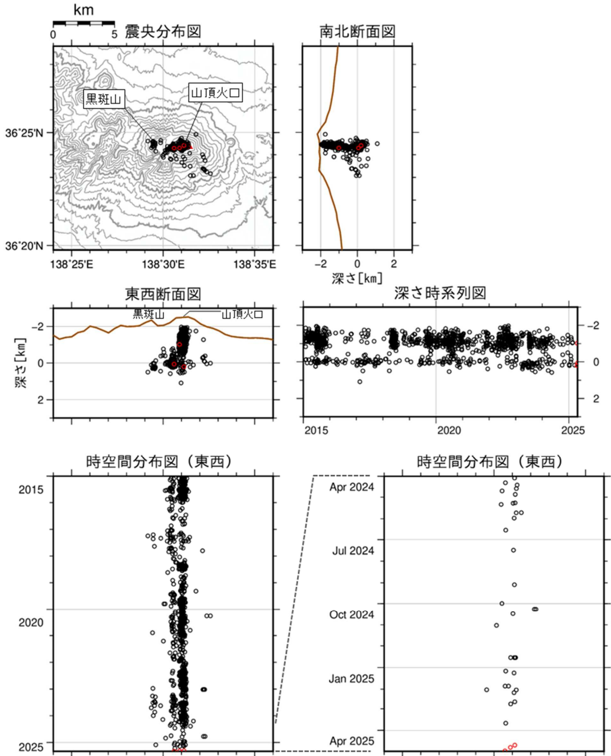
図5 浅間山 震源分布図（2015年1月1日～2025年4月30日）
