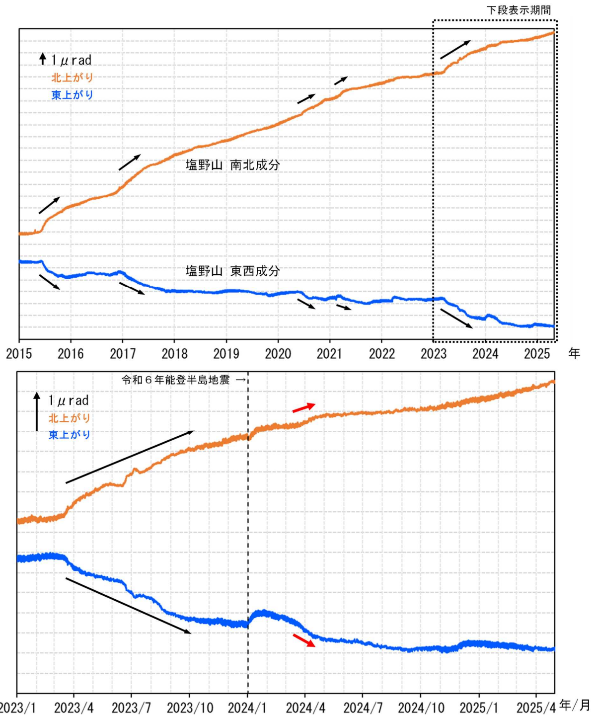
図6 浅間山 塩野山観測点における傾斜データ（2015年1月1日～2025年4月30日）
