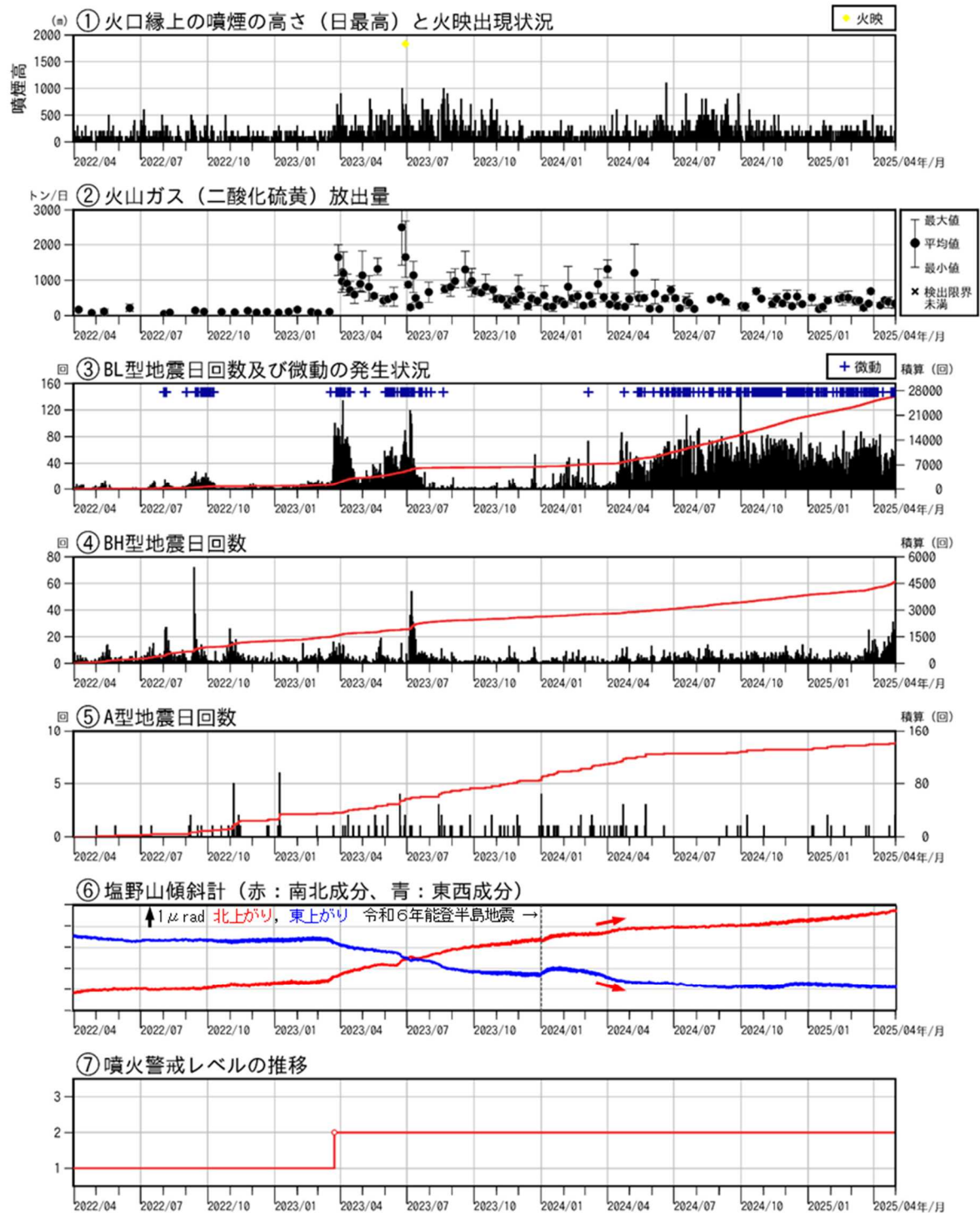
図2 浅間山 短期火山活動経過図（2022年4月1日～2025年4月30日）
