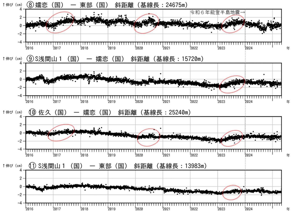
図7-2 浅間山 GNSS 連続観測結果（2016年1月1日～2025年4月30日）
