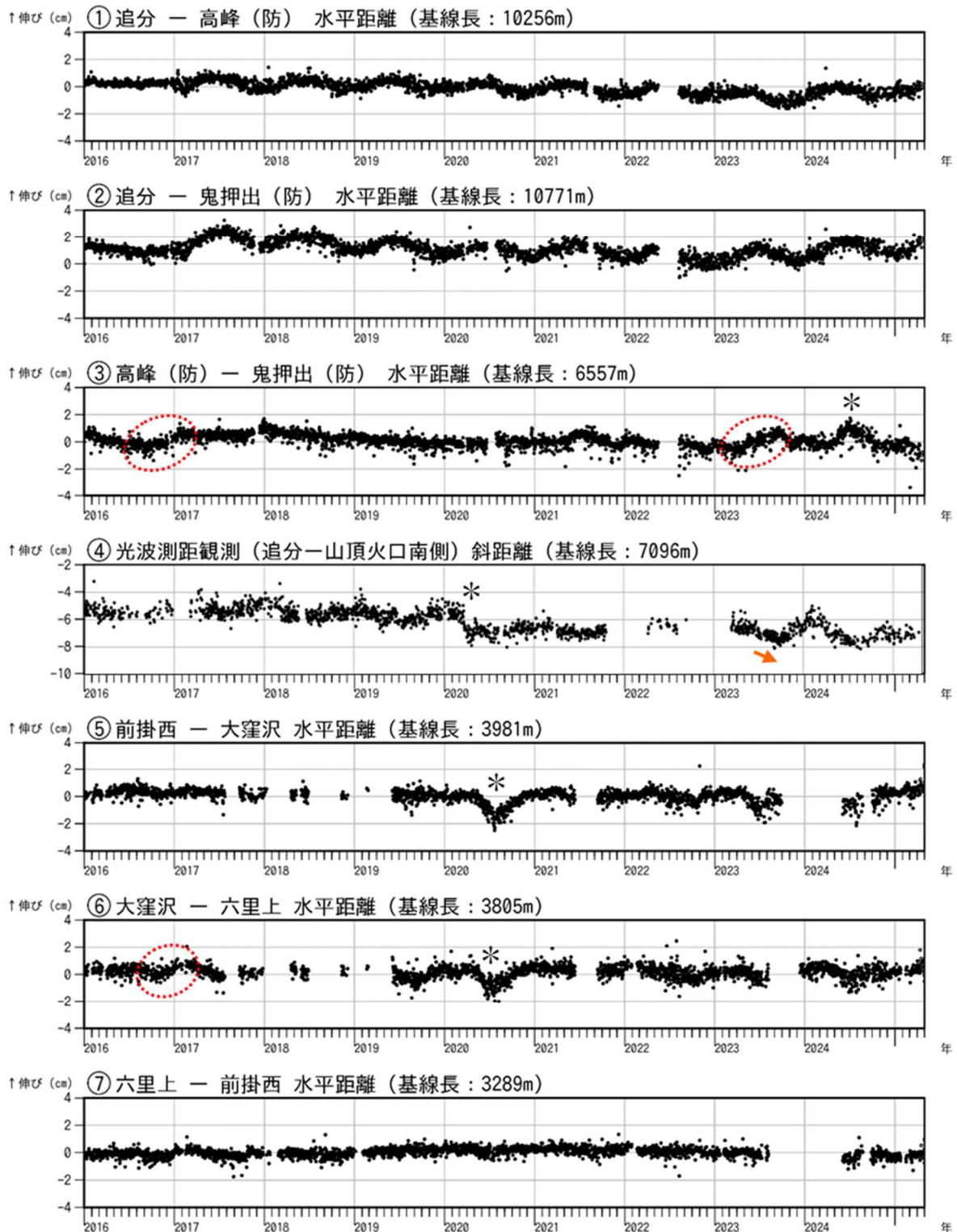
図7-1 浅間山 GNSS 連続観測及び光波測距観測結果(2016年1月1日~2025年4月30日)
