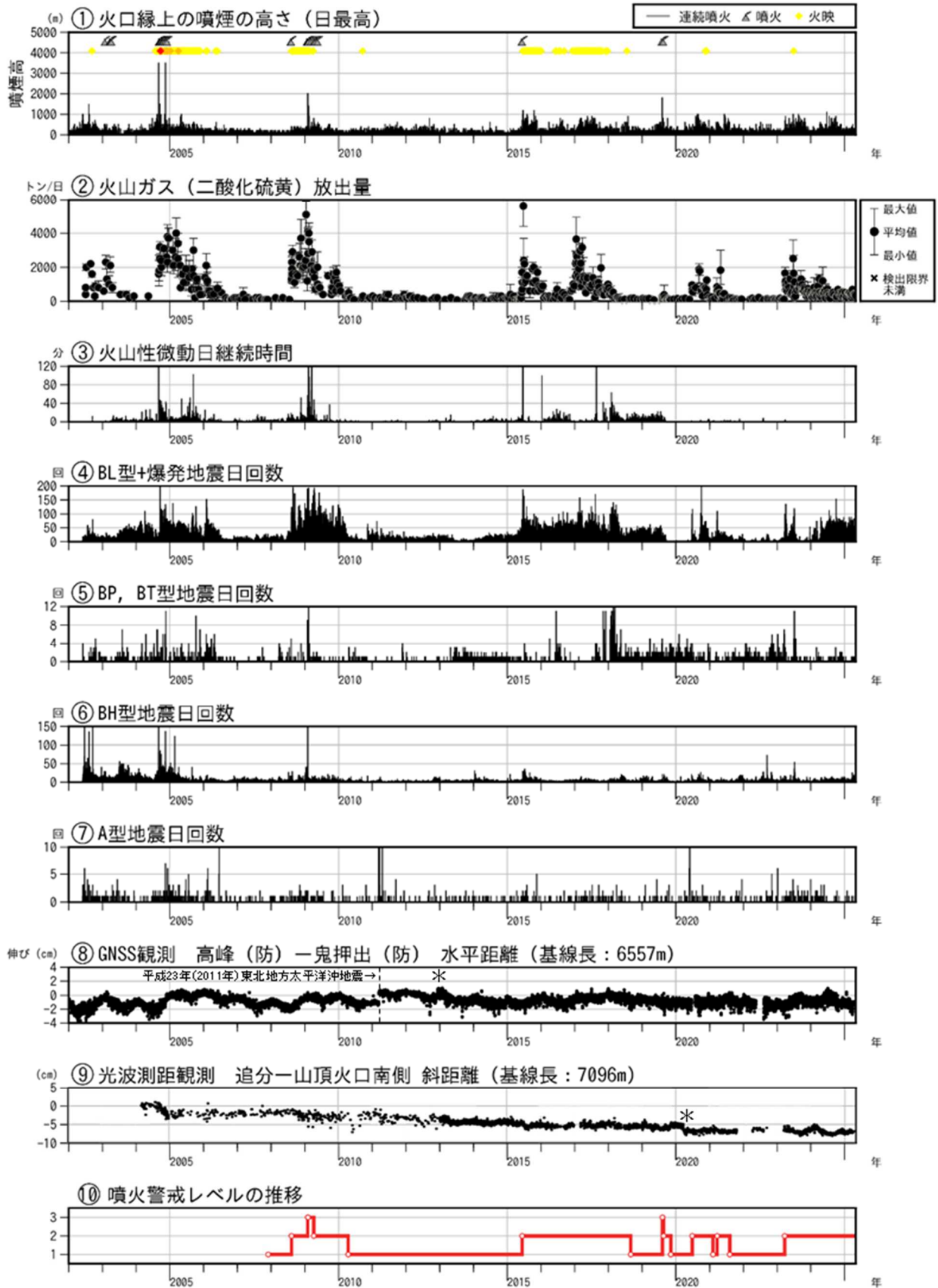
図3 浅間山 長期火山活動経過図（2002年1月1日～2025年4月30日）
