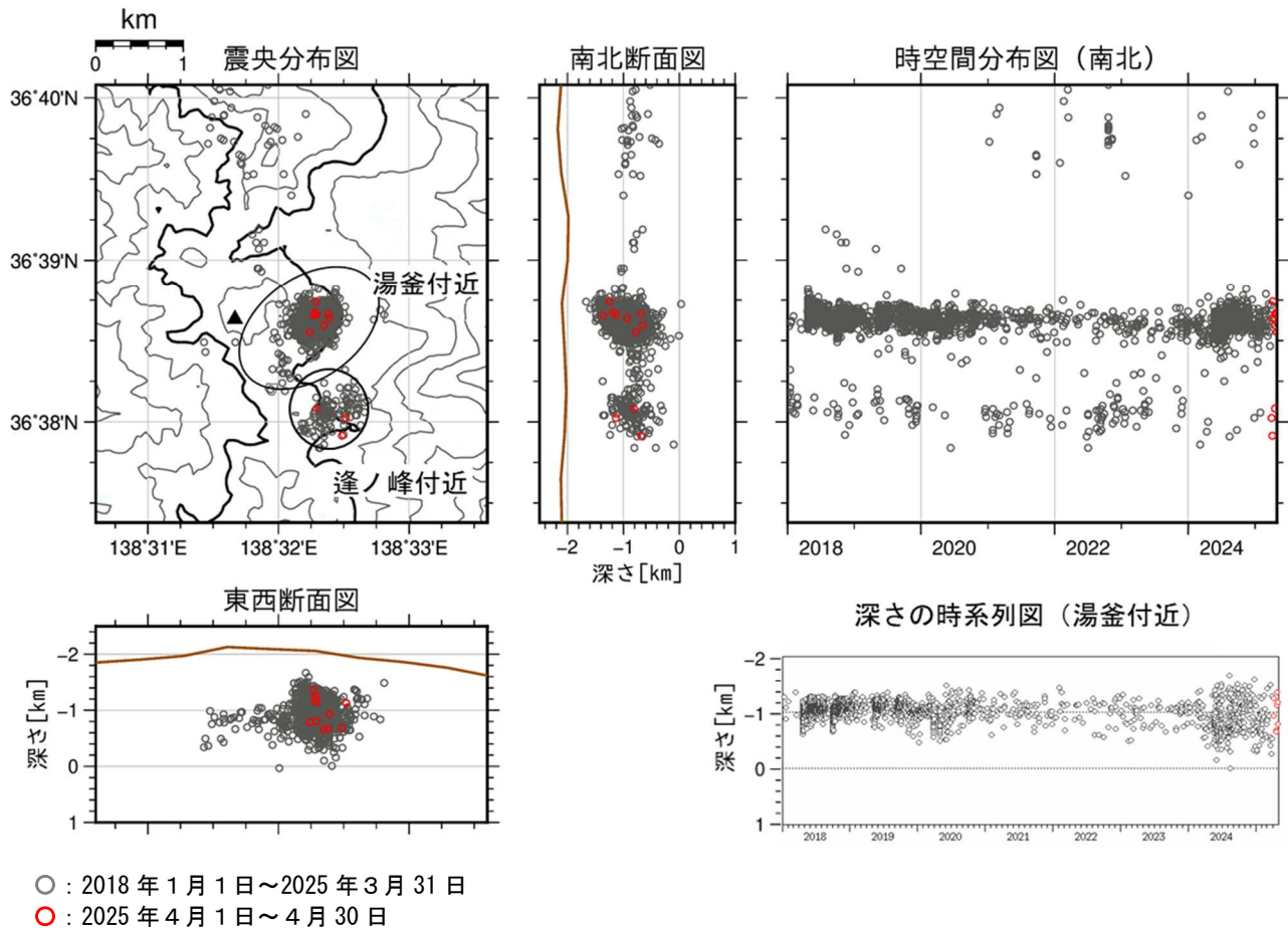
図4 草津白根山 震源分布図（2018 年 1 月 1 日～2025 年 4 月 30 日）
