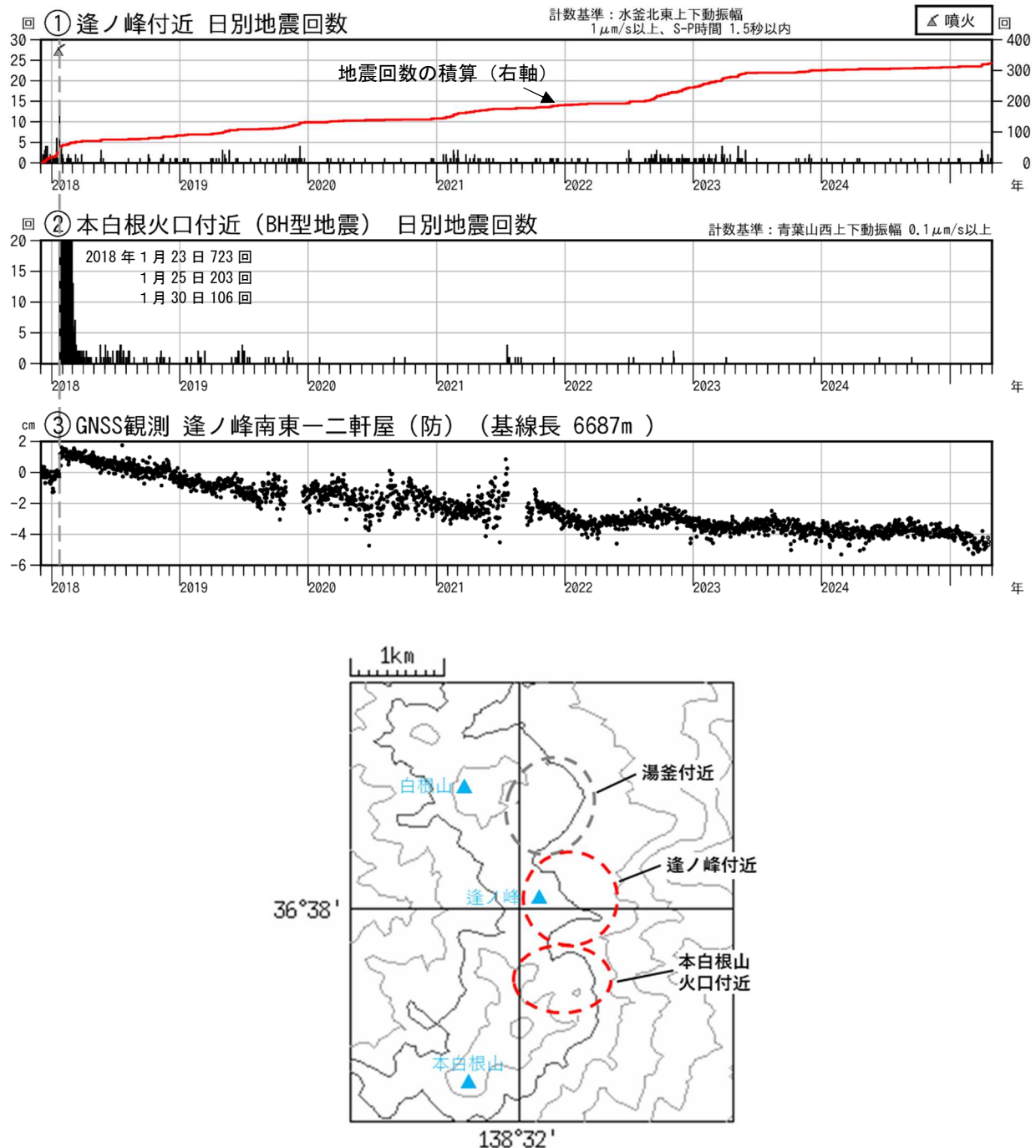
図12 草津白根山（本白根山） 火山活動経過図（2017年12月1日～2025年4月30日）
