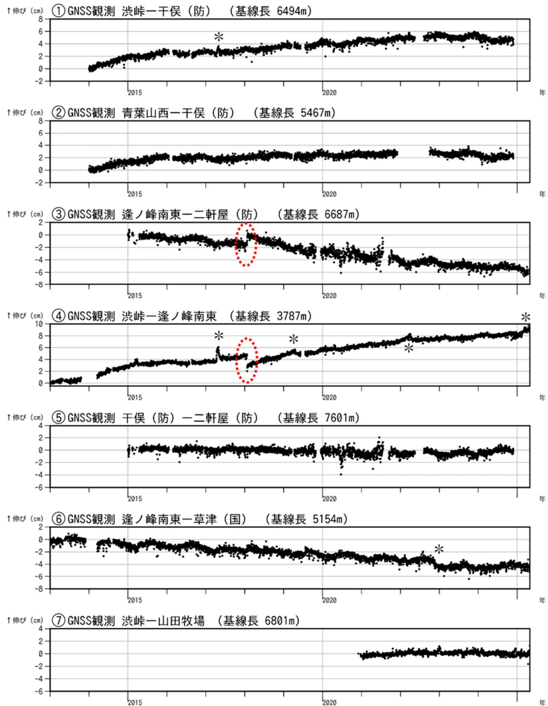
図6 草津白根山 GNSS 連続観測の結果（2013 年 1 月 1 日～2025 年 4 月 30 日）
