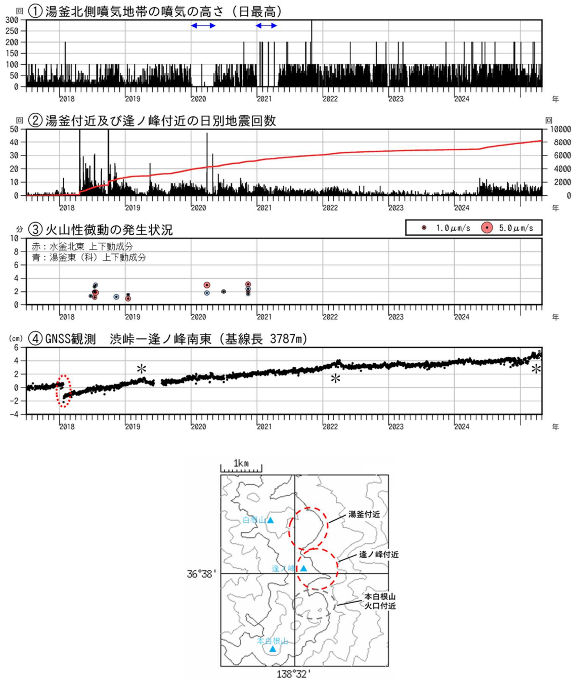
図3 草津白根山（白根山（湯釜付近）） 火山活動経過図（2017年7月1日～2025年4月30日）
