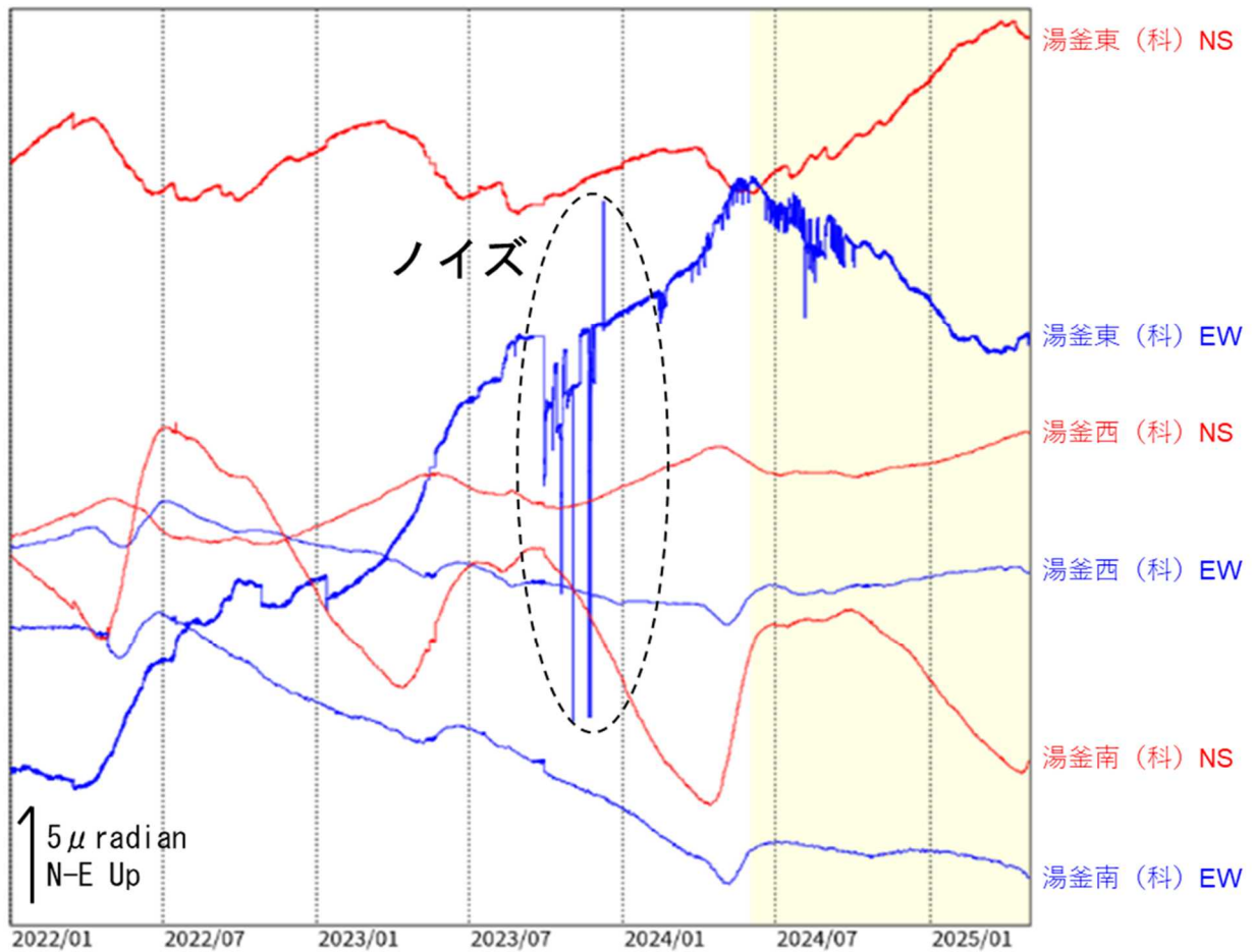
図5 草津白根山（白根山（湯釜付近）） 傾斜変動（2022年1月1日～2025年4月30日） （科）：東京科学大学
