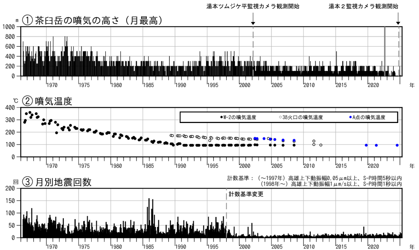
図3-1 那須岳 火山活動経過図（1966年6月～2025年4月）
