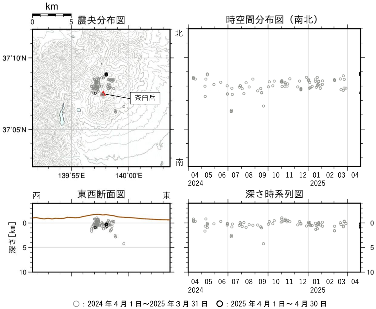
図5 那須岳 震源分布図（2024 年 4 月 1 日～2025 年 4 月 30 日）
