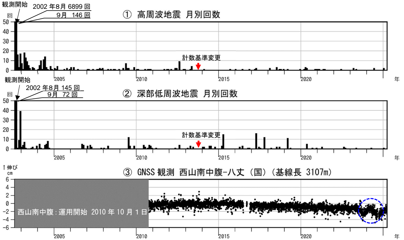
図2 八丈島 火山活動経過図（2002年8月13日～2025年3月31日）
