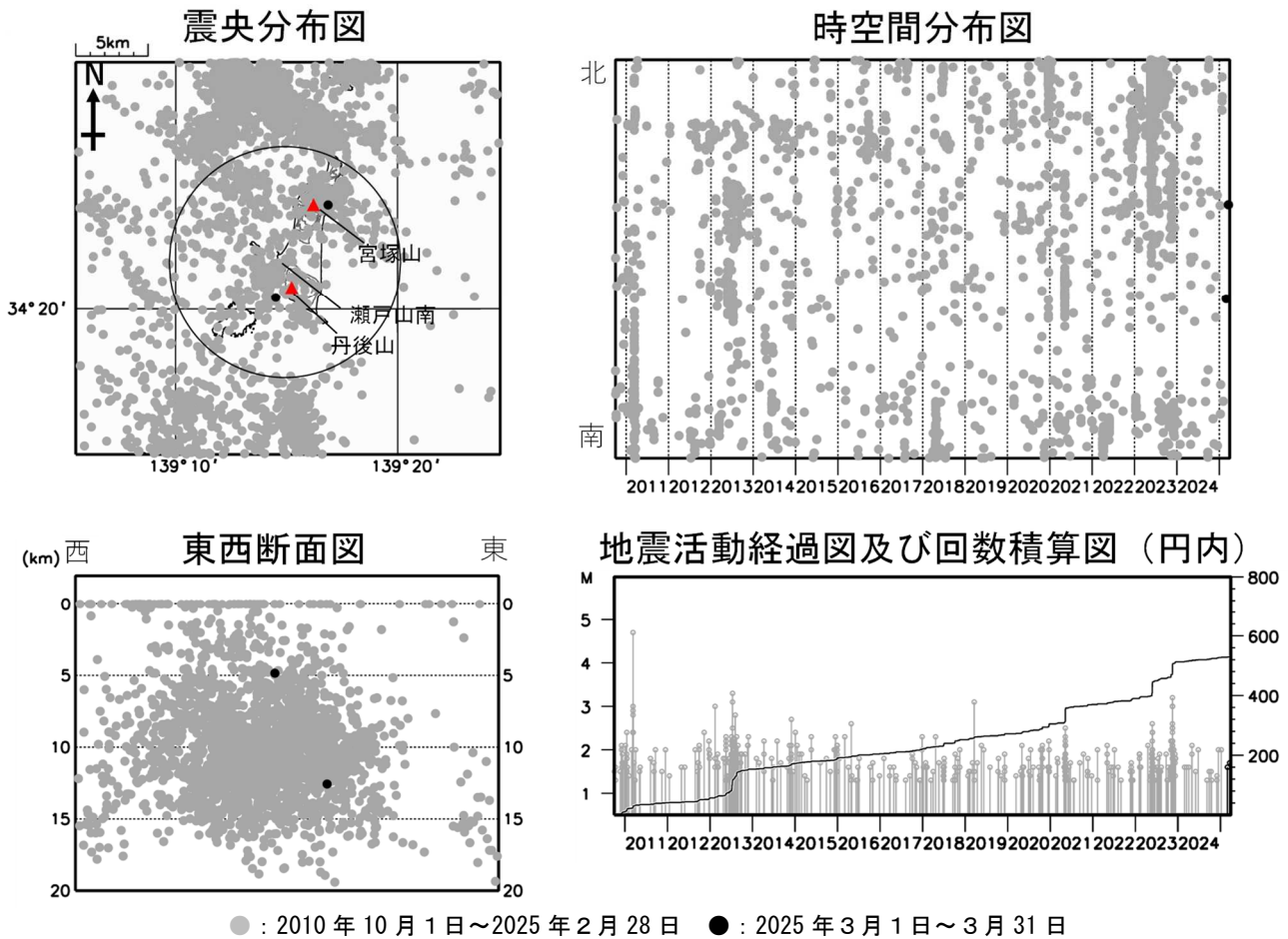
図 3 新島 広域地震観測網による山体・周辺の地震活動（2010 年 10 月 1 日～2025 年 3 月 31 日） 広域地震観測網により震源決定したもので、深さは全て海面以下として決定しています。なお、2020 年 9 月以降については、地震観測点の標高を考慮する等、震源決定の手法を変更しております。 M（マグニチュード）は地震の規模を表し、M1.3 以上の地震を示しています。 図中の震源要素は一部暫定値が含まれており、後日変更することがあります。 計数対象（瀬戸山南から半径約 8 km、深さ約 20km 以内）以外の地震が含まれるため、図 2－①の日別 A 型地震回数とは異なります。 震央分布図中の円は火山性地震の回数の計数対象（瀬戸山南から半径 8 km、深さ 20km 以内）の範囲を示しています。 ・地震活動は低調に経過しました。
