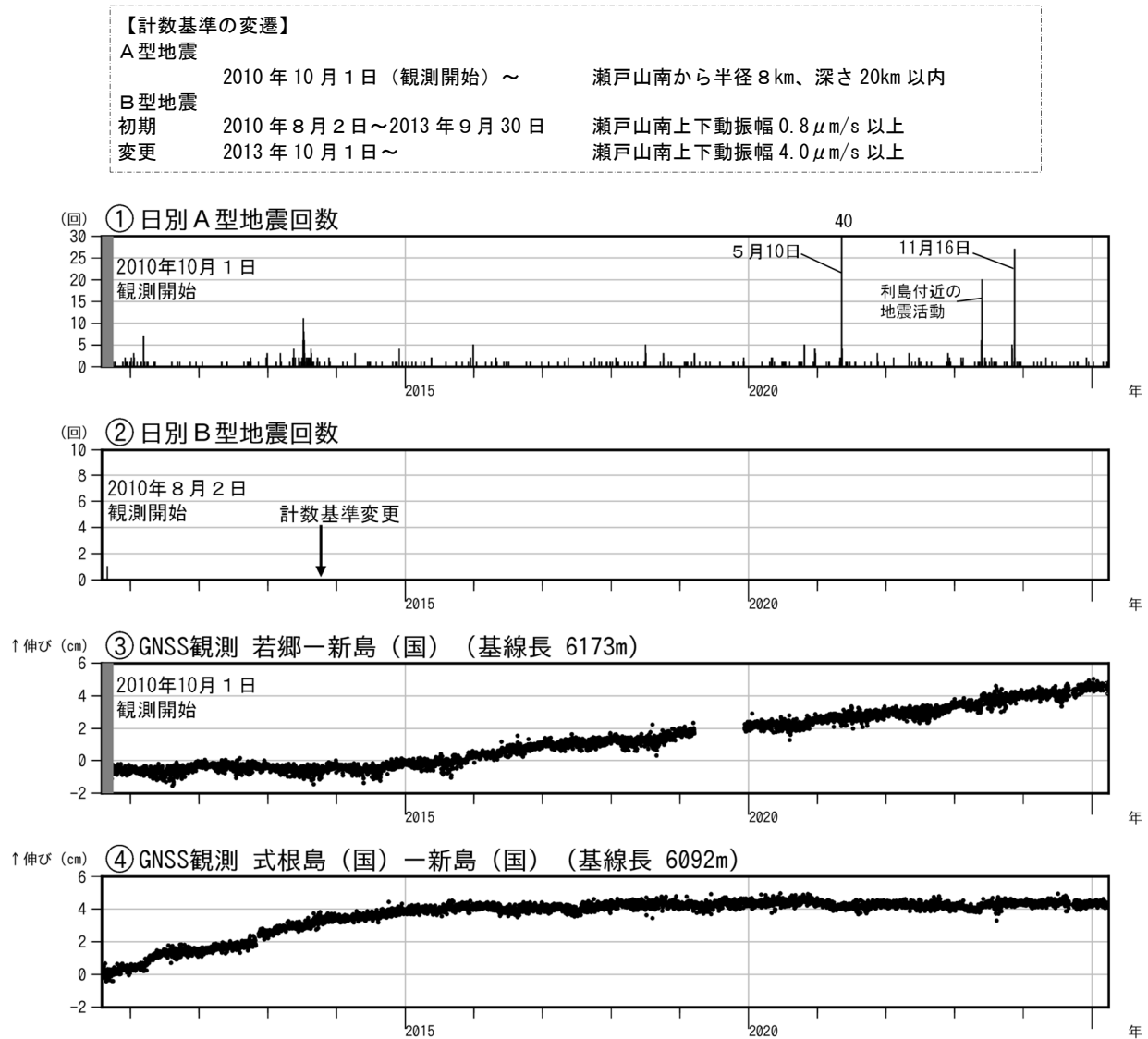
図2 新島 火山活動経過図(2010年8月2日～2025年3月31日)
