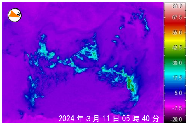
中央火孔東カメラ位置からの熱画像 （2024年3月11日 現地調査時に撮影）
