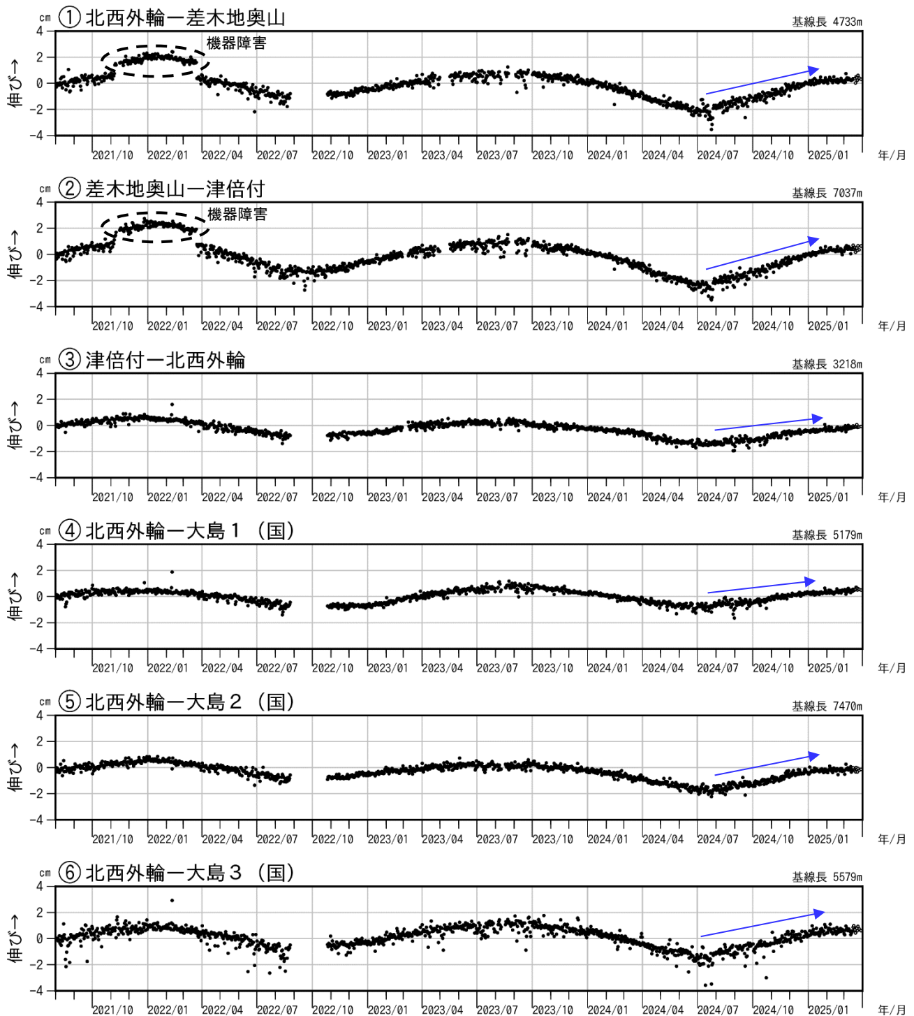
図3-2 伊豆大島 GNSS 連続観測による基線長変化(2021年8月～2025年3月31日)
