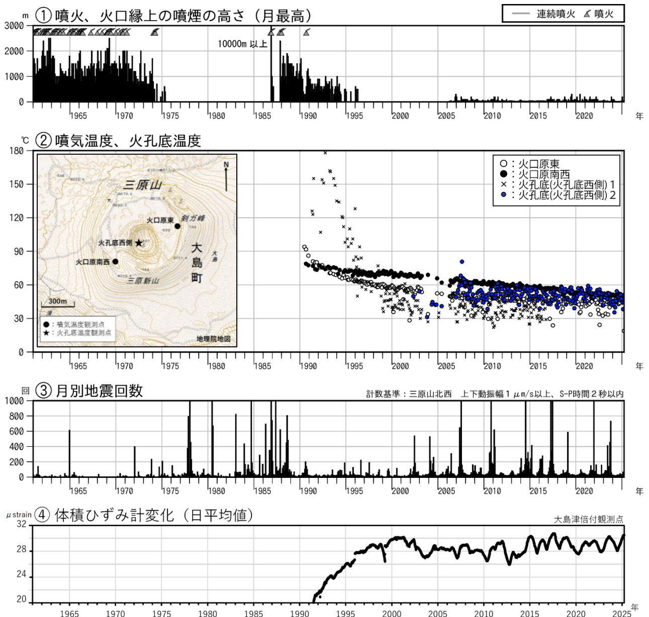
図1 伊豆大島 長期間の火山活動経過図（1961年1月～2025年3月31日）
