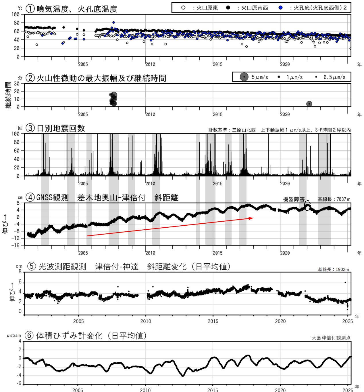
図2 伊豆大島 最近の火山活動経過図（2001年1月～2025年3月31日）
