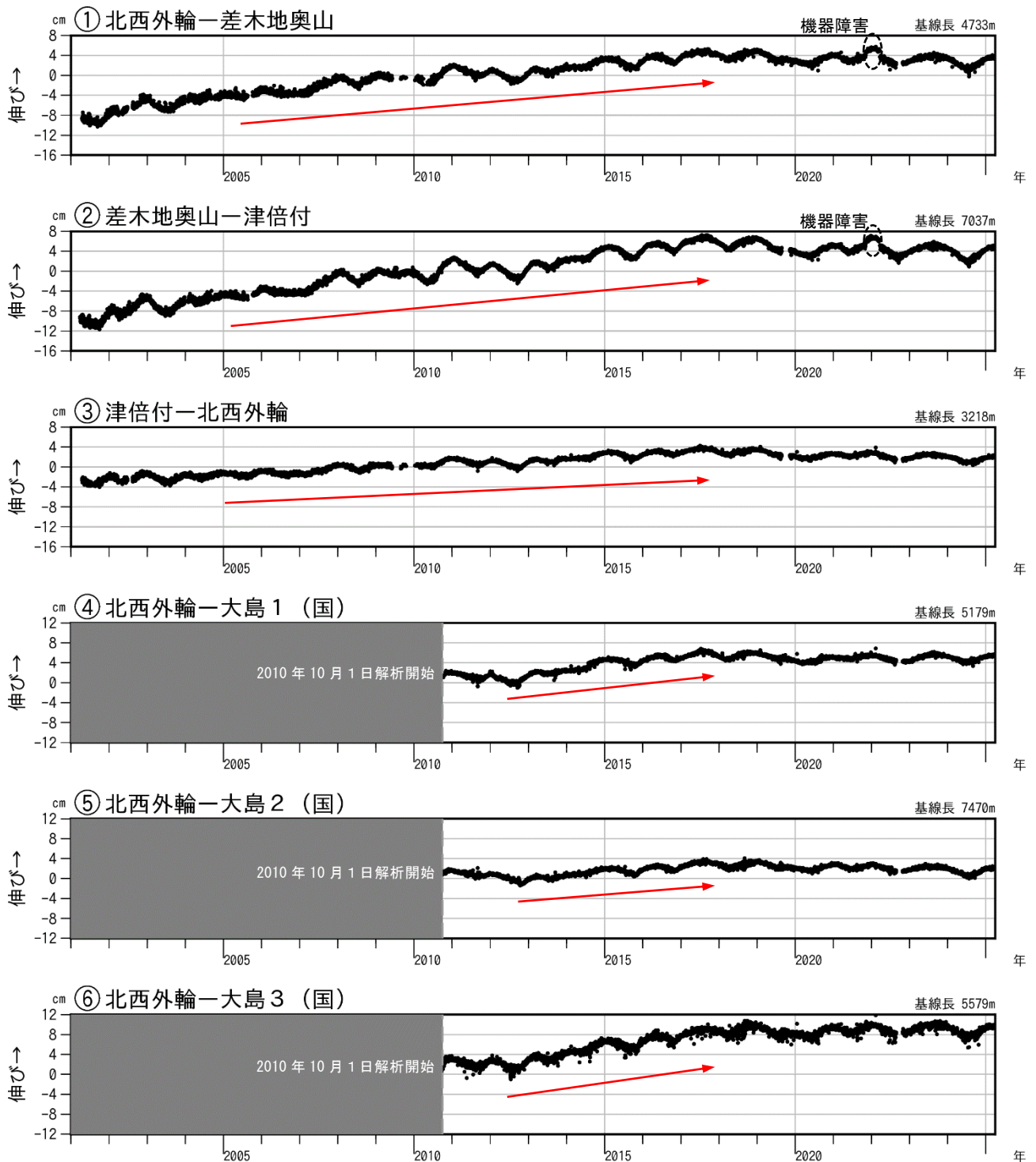
図 3-1 伊豆大島 GNSS 連続観測による基線長変化(2001 年 1 月～2025 年 3 月 31 日)
