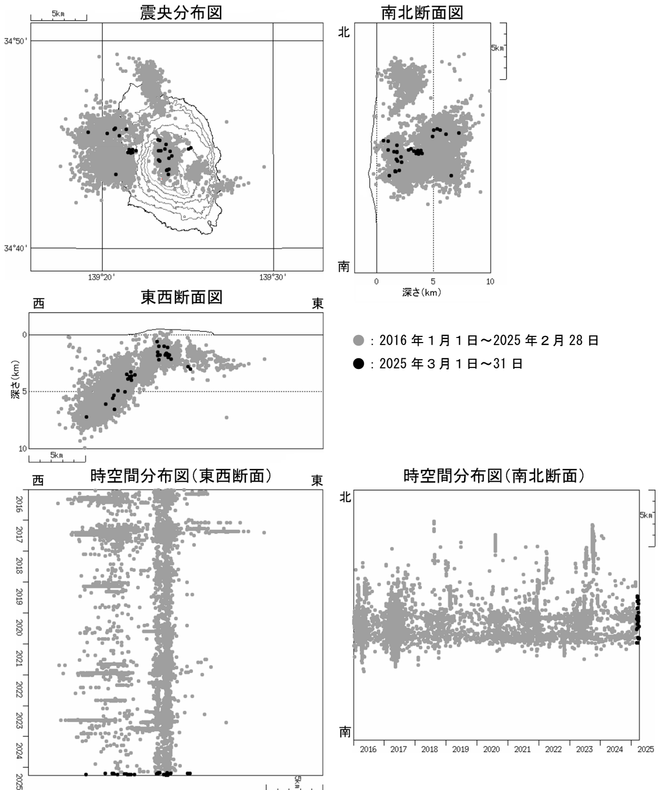
図4 伊豆大島 震源分布図（2016 年 1 月 1 日～2025 年 3 月 31 日）
