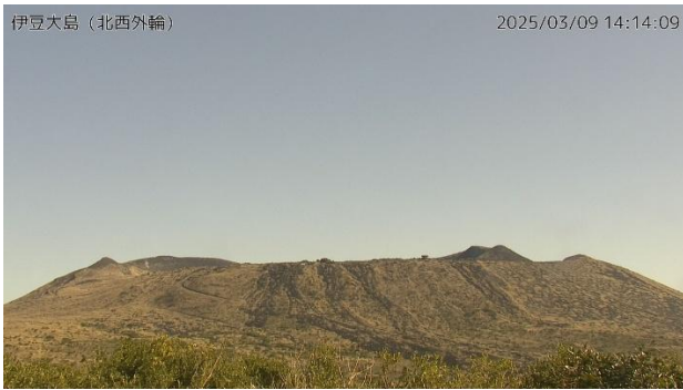
山頂部（3月9日、北西外輪監視カメラによる）
