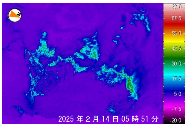
中央火孔東カメラ位置からの熱画像 （2月14日 現地調査時に撮影）
