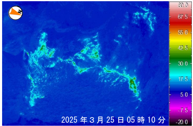
中央火孔東カメラ位置からの熱画像 （3月25日 現地調査時に撮影）
