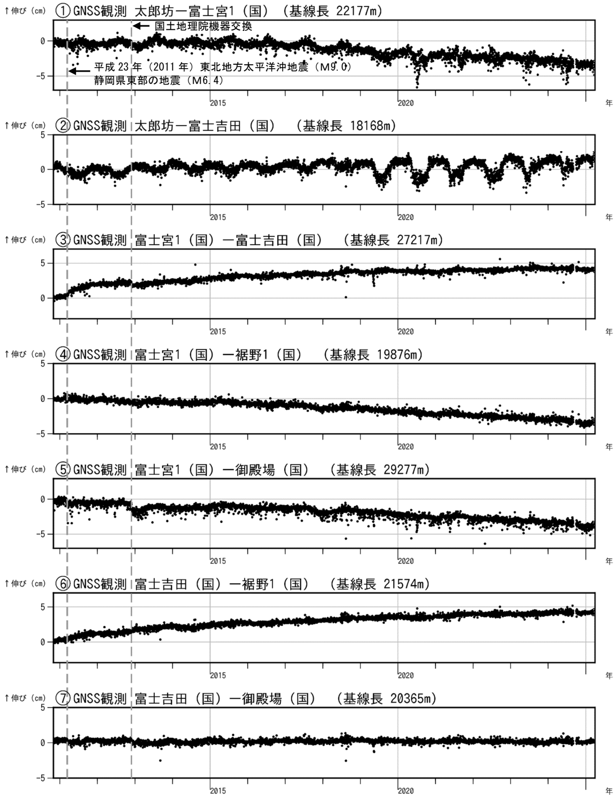
図4 富士山 GNSS 連続観測による基線長変化 (2010 年 10 月 1 日～2025 年 3 月 31 日)
