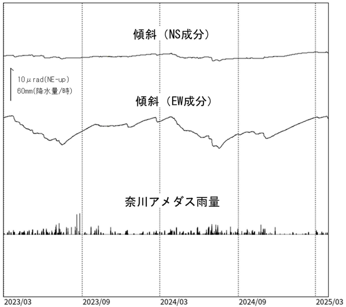
図4 乗鞍岳 三本滝観測点における傾斜データ（2023年3月1日～2025年3月31日）
