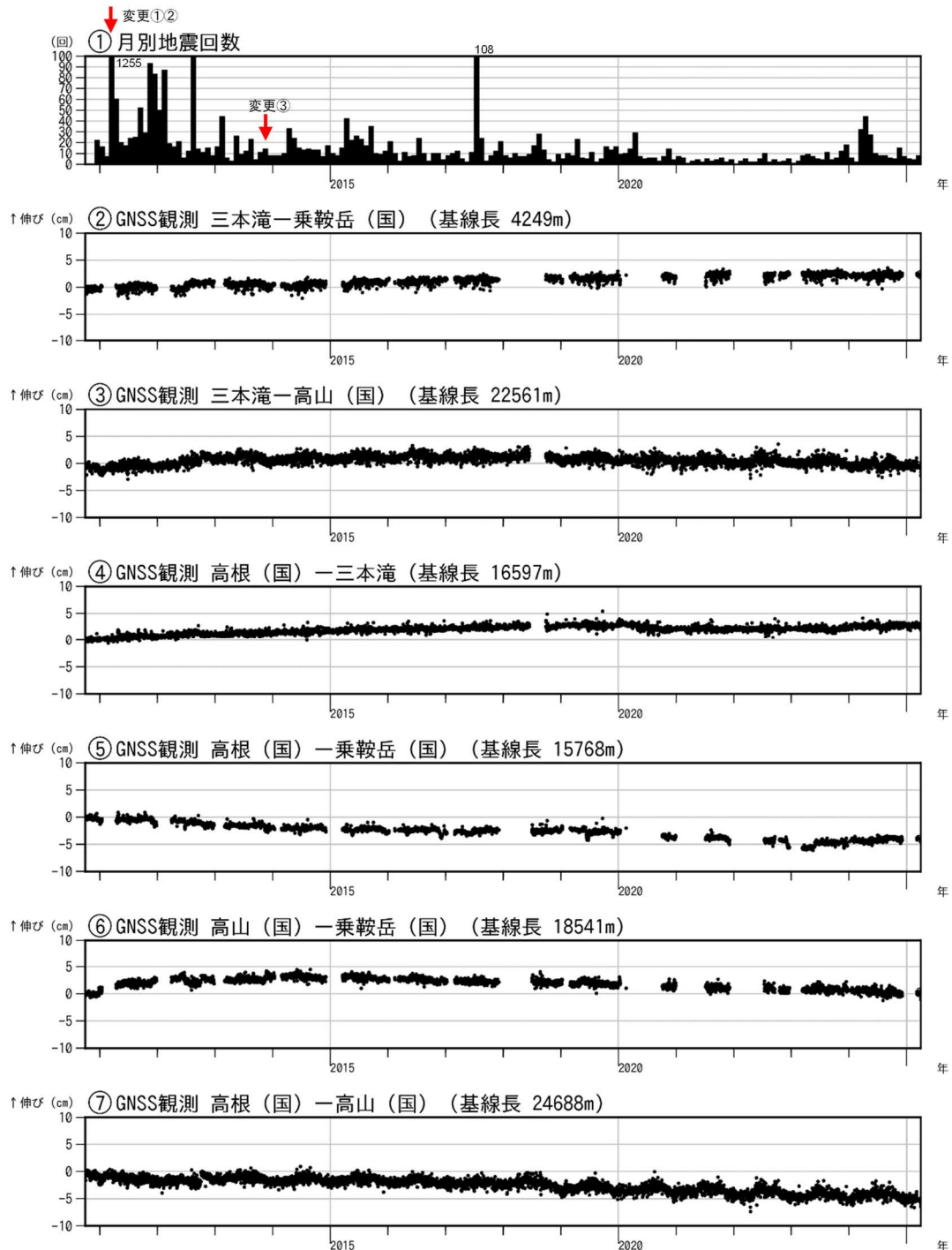
図2 乗鞍岳 火山活動経過図（2010年10月1日～2025年3月31日）
