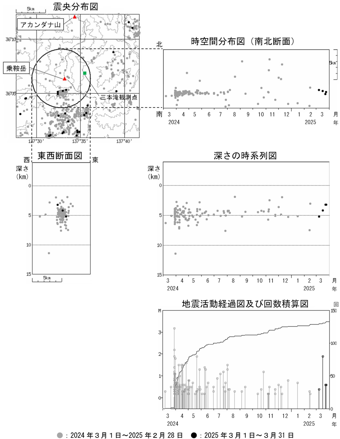
図 3 乗鞍岳 広域地震観測網による山体・周辺の地震活動(2024 年 3 月 1 日～2025 年 3 月 31 日)
