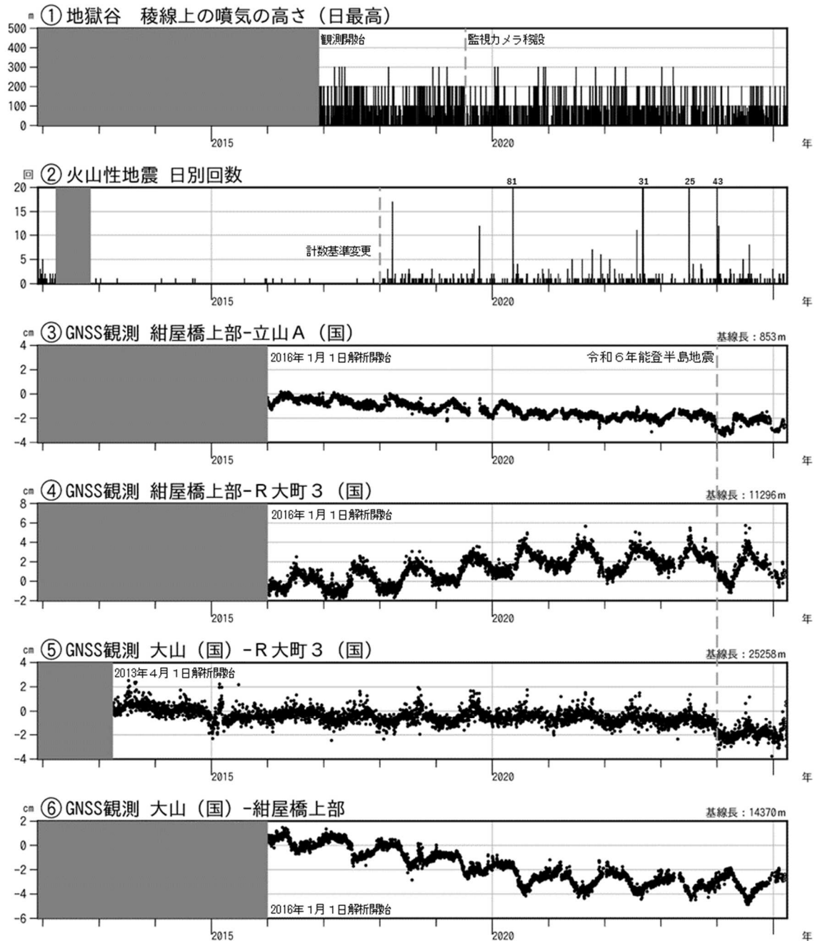
図3 弥陀ヶ原 火山活動経過図（2011年12月1日～2025年3月31日）
