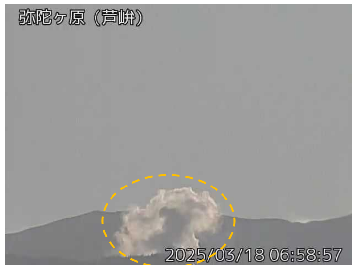
図1 弥陀ヶ原 地獄谷からの噴気の状況（橙丸）（3月18日、芦峯監視カメラによる）
