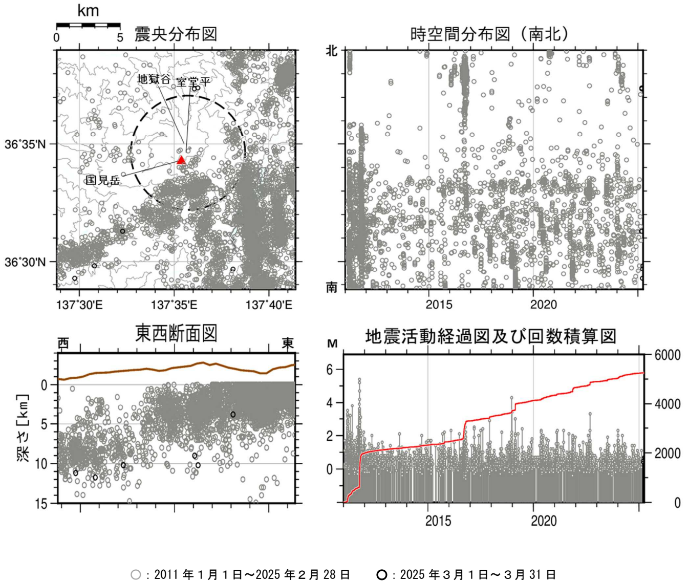
図 2 弥陀ヶ原 広域地震観測網による山体・周辺の地震活動（2011 年 1 月 1 日～2025 年 3 月 31 日） 震央分布図中の円は弥陀ヶ原の計数対象地震（室堂平で S-P 時間 1 秒以内）のおよその範囲を示しています。 広域地震観測網により震源決定したもので、深さは全て海面以下として決定しています。なお、2020 年 9 月以降については、地震観測点の標高を考慮する等、震源決定の手法を変更しております。 図中の震源要素は一部暫定値が含まれており、後日変更することがあります。
