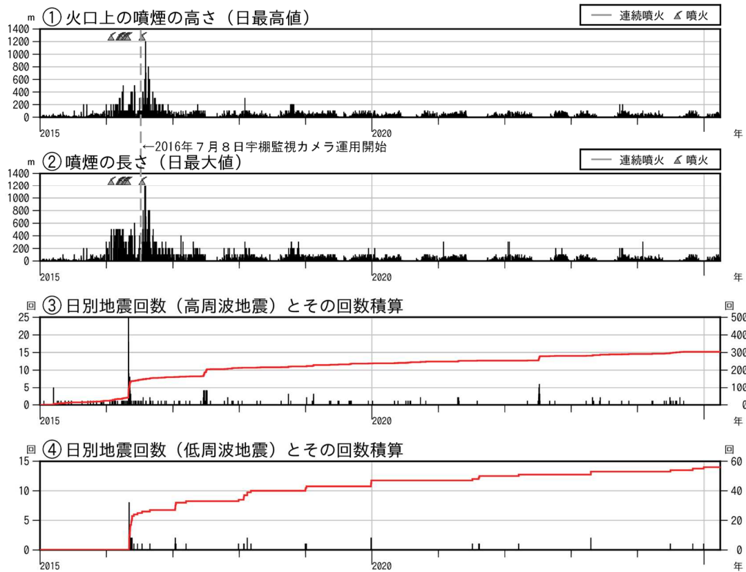
図 3 新潟焼山 火山活動経過図（短期）（2015 年 1 月 1 日～2025 年 3 月 31 日）
