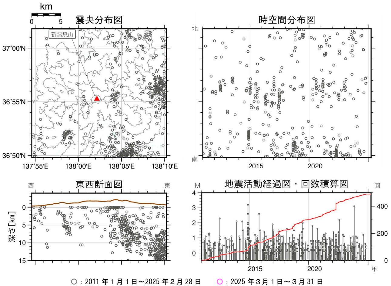
図4 新潟焼山 広域地震観測網による山体・周辺の地震活動（2011年1月1日～2025年3月31日）
