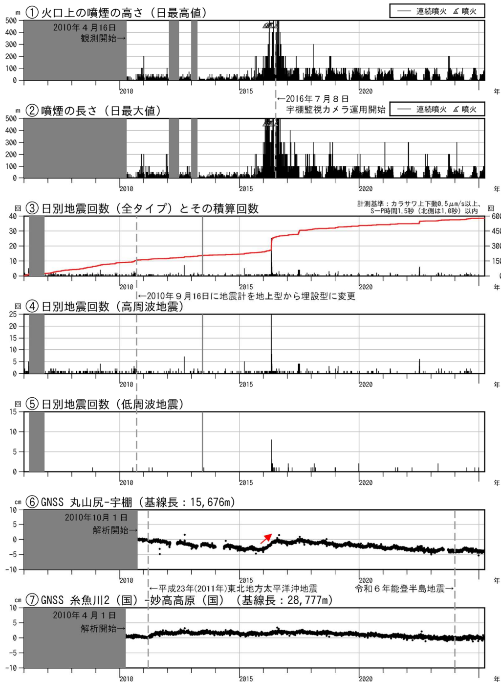
図2 新潟焼山 火山活動経過図（2006年1月1日～2025年3月31日）
