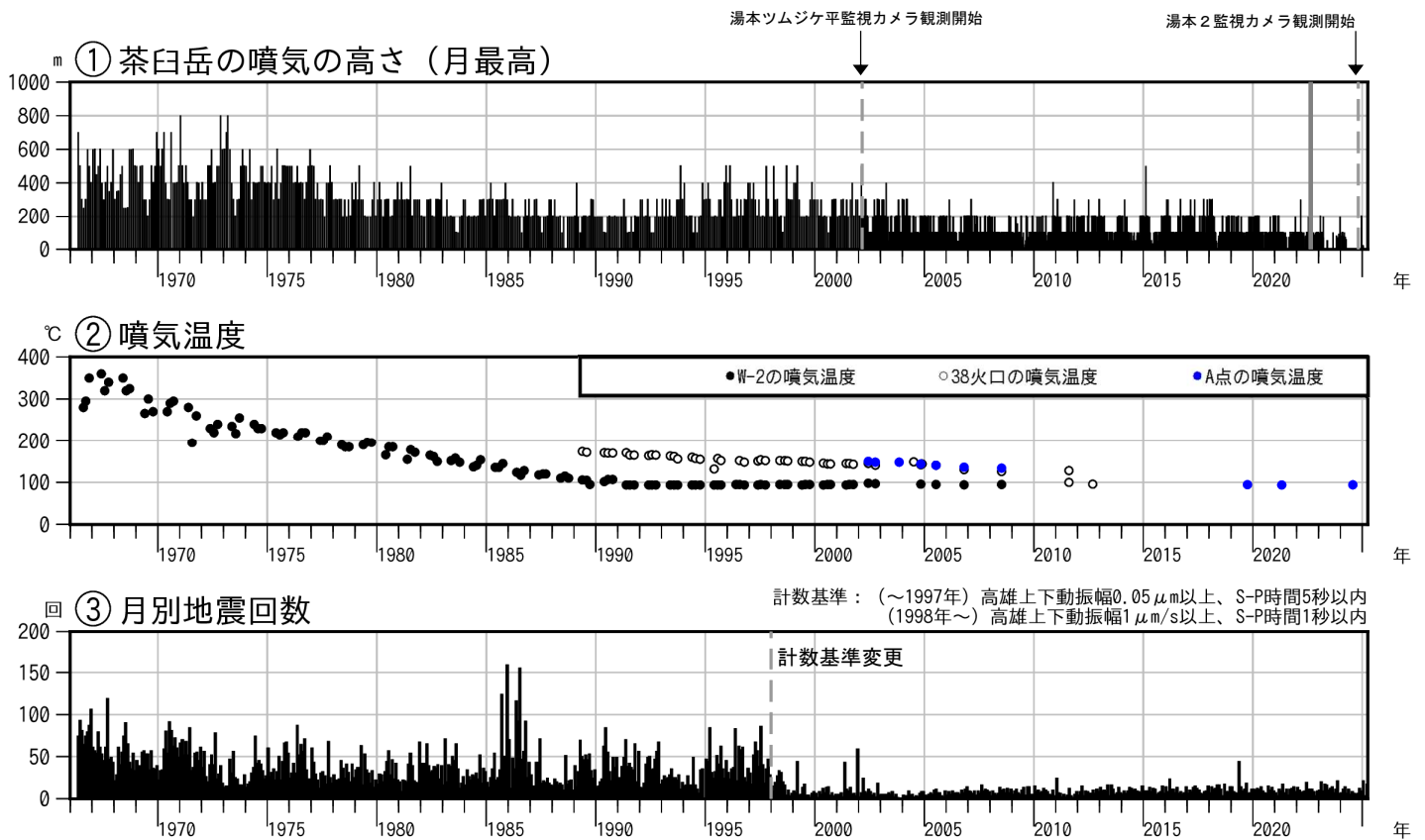
図3-1 那須岳 火山活動経過図（1966年6月～2025年3月）
