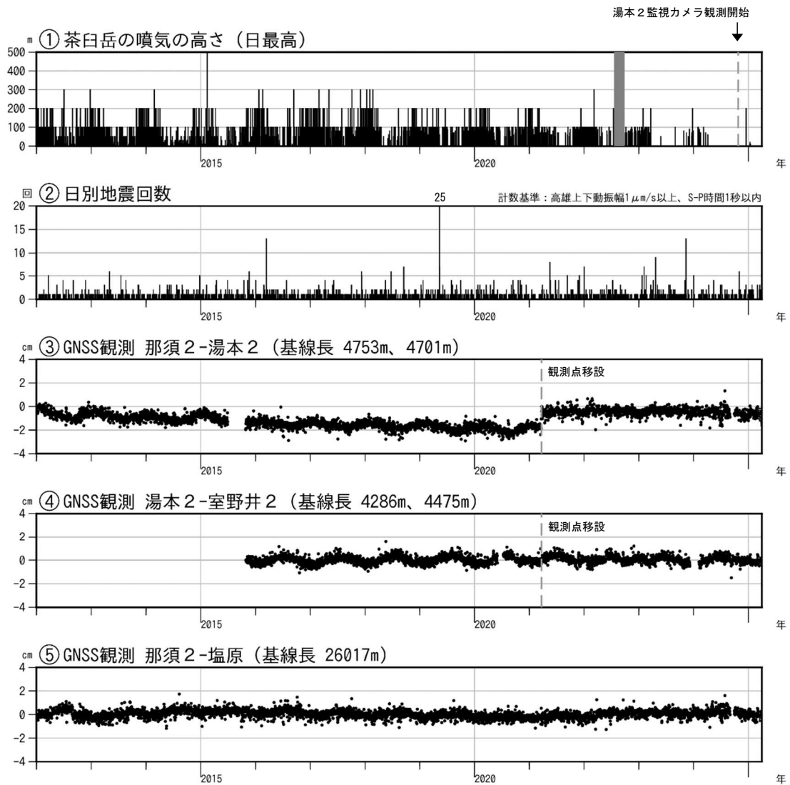
図4 那須岳 火山活動経過図（2012年1月1日～2025年3月31日）
