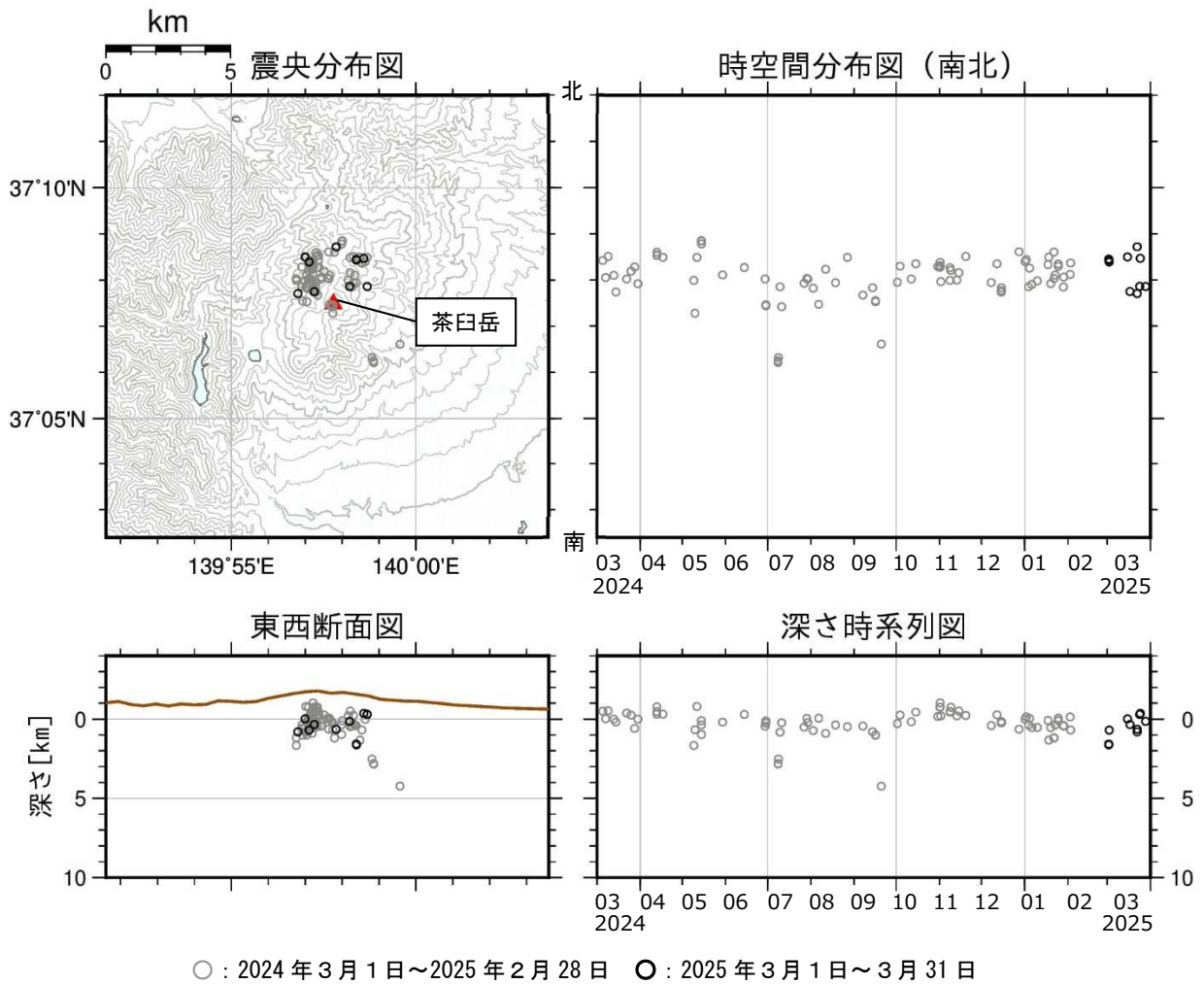
図5 那須岳 震源分布図（2024 年 3 月 1 日～2025 年 3 月 31 日）
