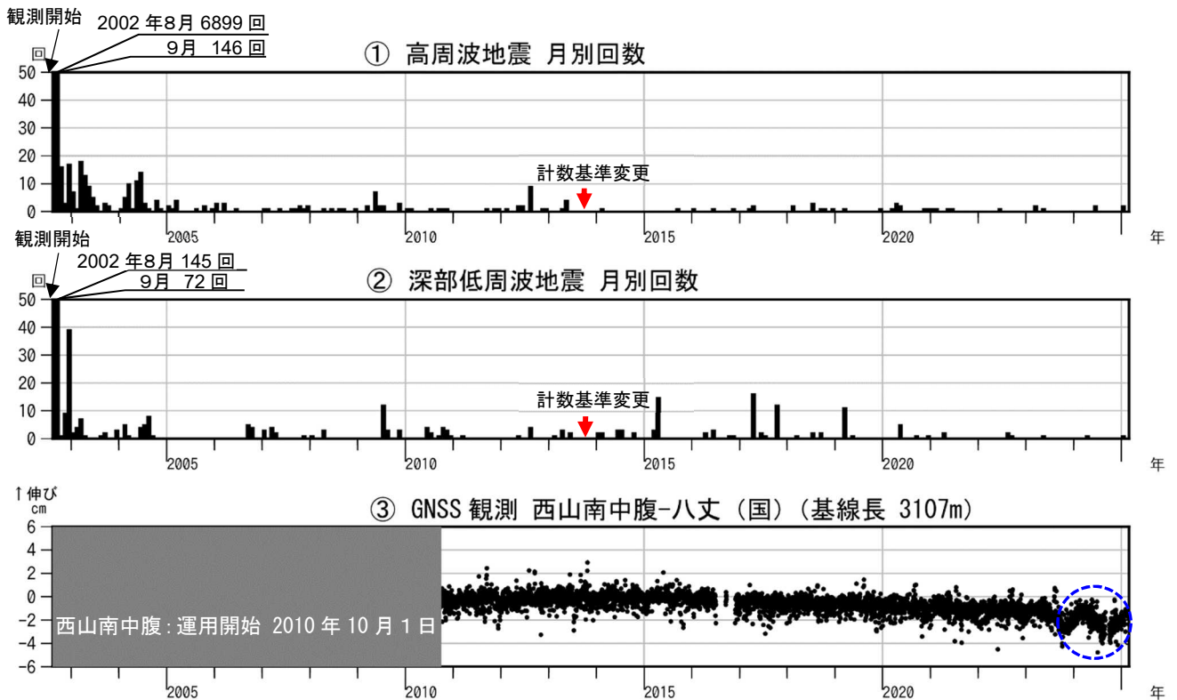
図2 八丈島 火山活動経過図（2002年8月13日～2025年2月28日）
