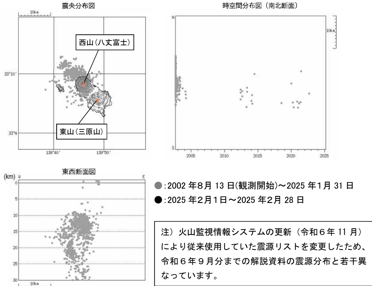
図3 八丈島 震源分布図（2002 年 8 月 13 日～2025 年 2 月 28 日）
