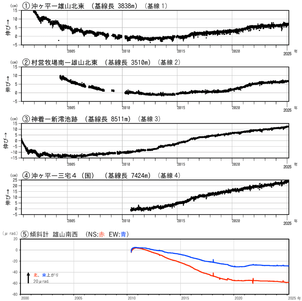
図8 三宅島 GNSS 連続観測及び傾斜計観測結果（2000 年 10 月 26 日～2025 年 2 月 28 日）
