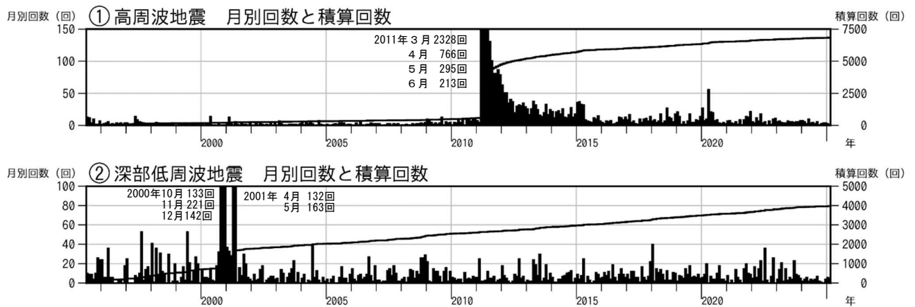
図2 富士山 月別地震回数（1995年6月1日～2025年2月28日）
