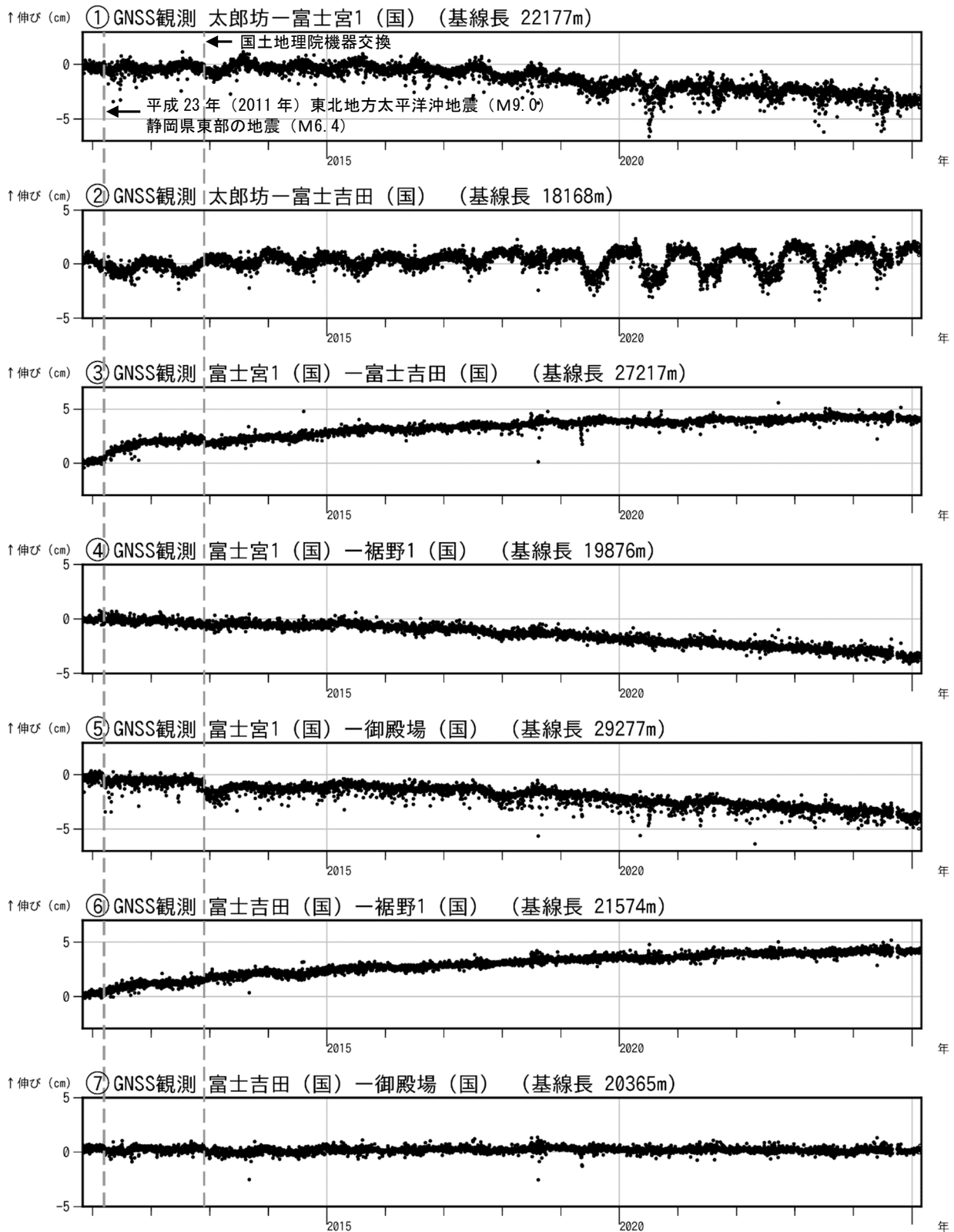
図4 富士山 GNSS連続観測による基線長変化(2010年10月1日～2025年2月28日)
