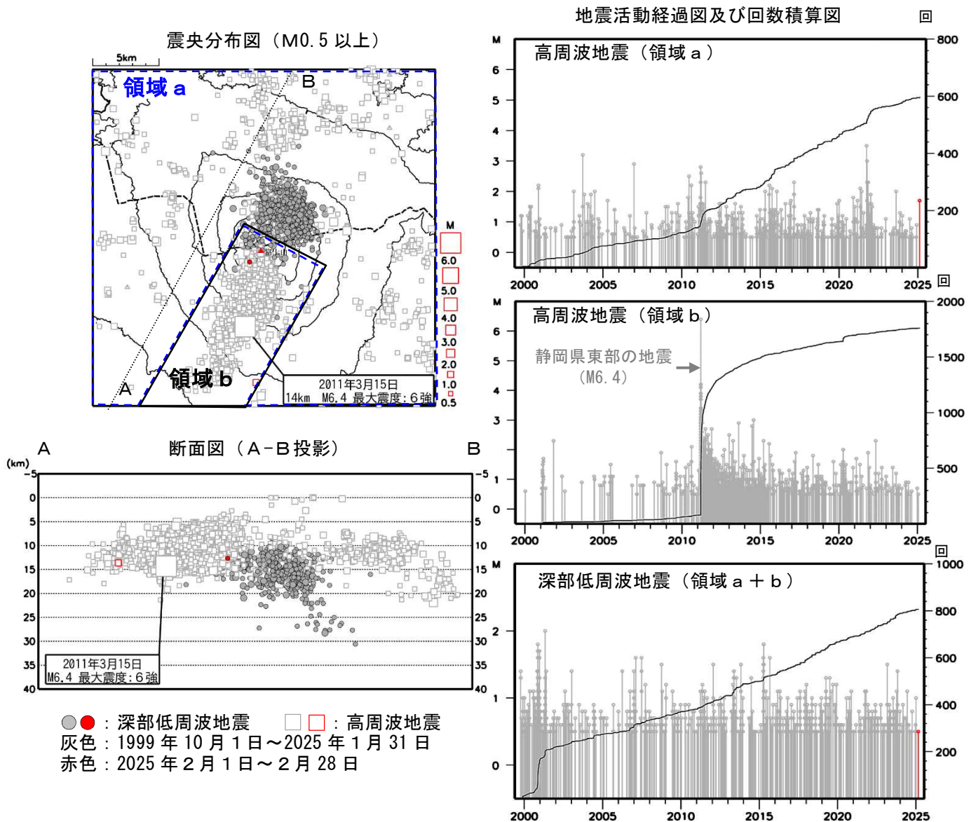
図3 富士山 広域地震観測網による山体及び周辺の地震活動(1999年10月1日～2025年2月28日)
