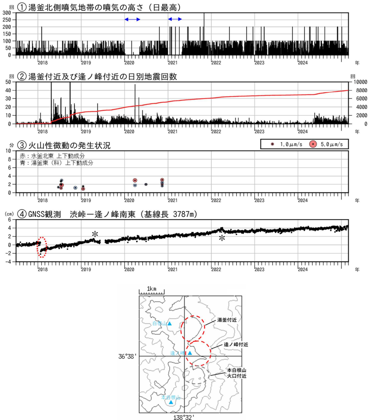
図3 草津白根山（白根山（湯釜付近）） 火山活動経過図（2017年7月1日～2025年2月28日）
