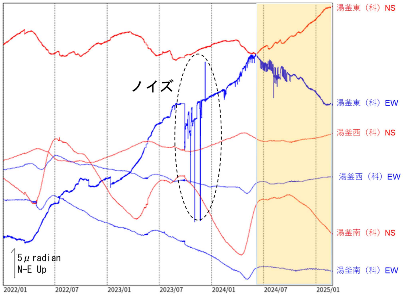
図 5 草津白根山（白根山（湯釜付近）） 傾斜変動（2022 年 1 月 1 日～2025 年 2 月 28 日） （科）：東京科学大学
