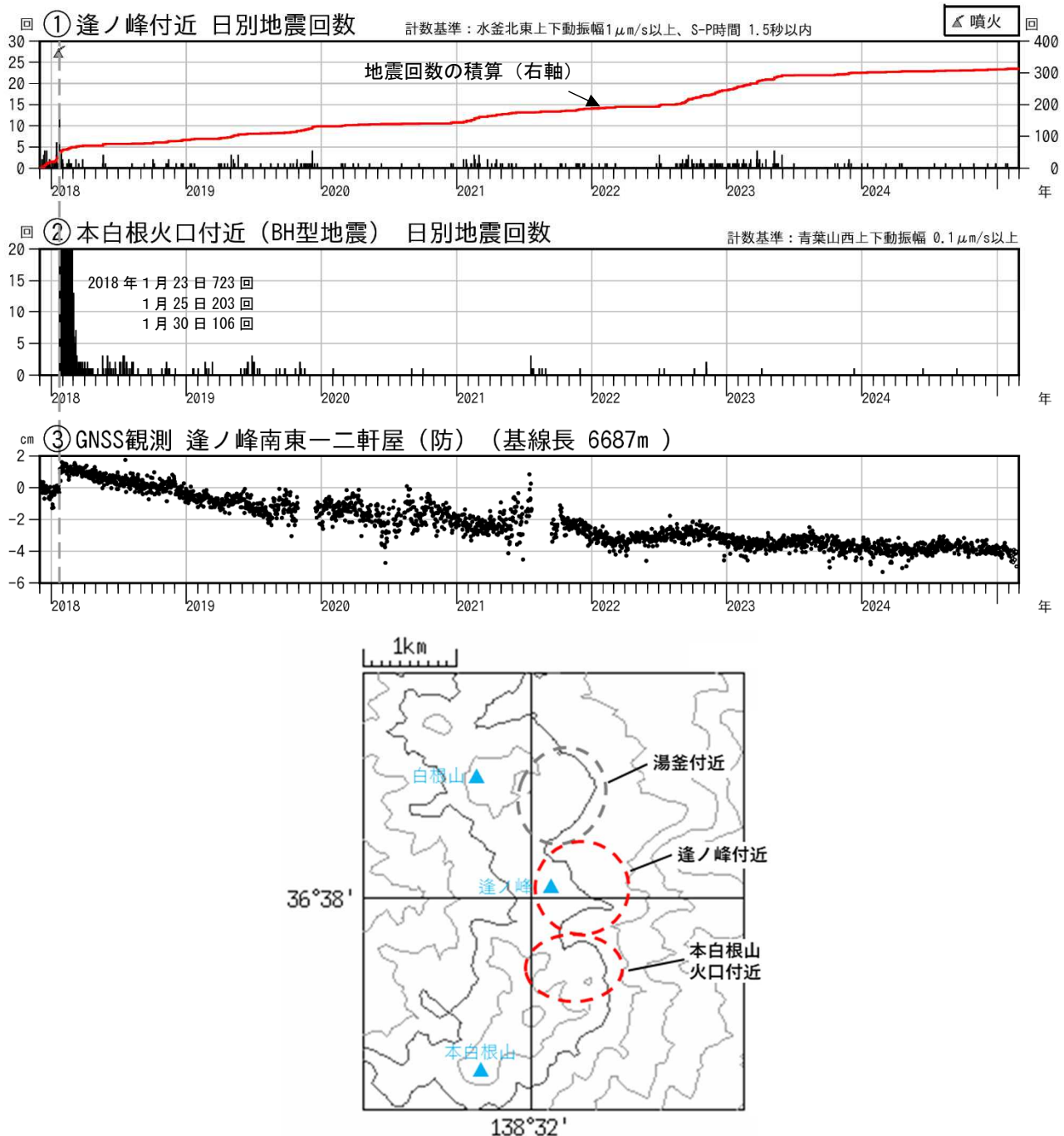
図12 草津白根山（本白根山） 火山活動経過図（2017年12月1日～2025年2月28日）
