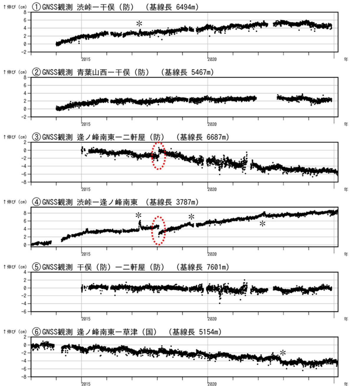
図6 草津白根山 GNSS 連続観測の結果（2013年1月1日～2025年2月28日）
