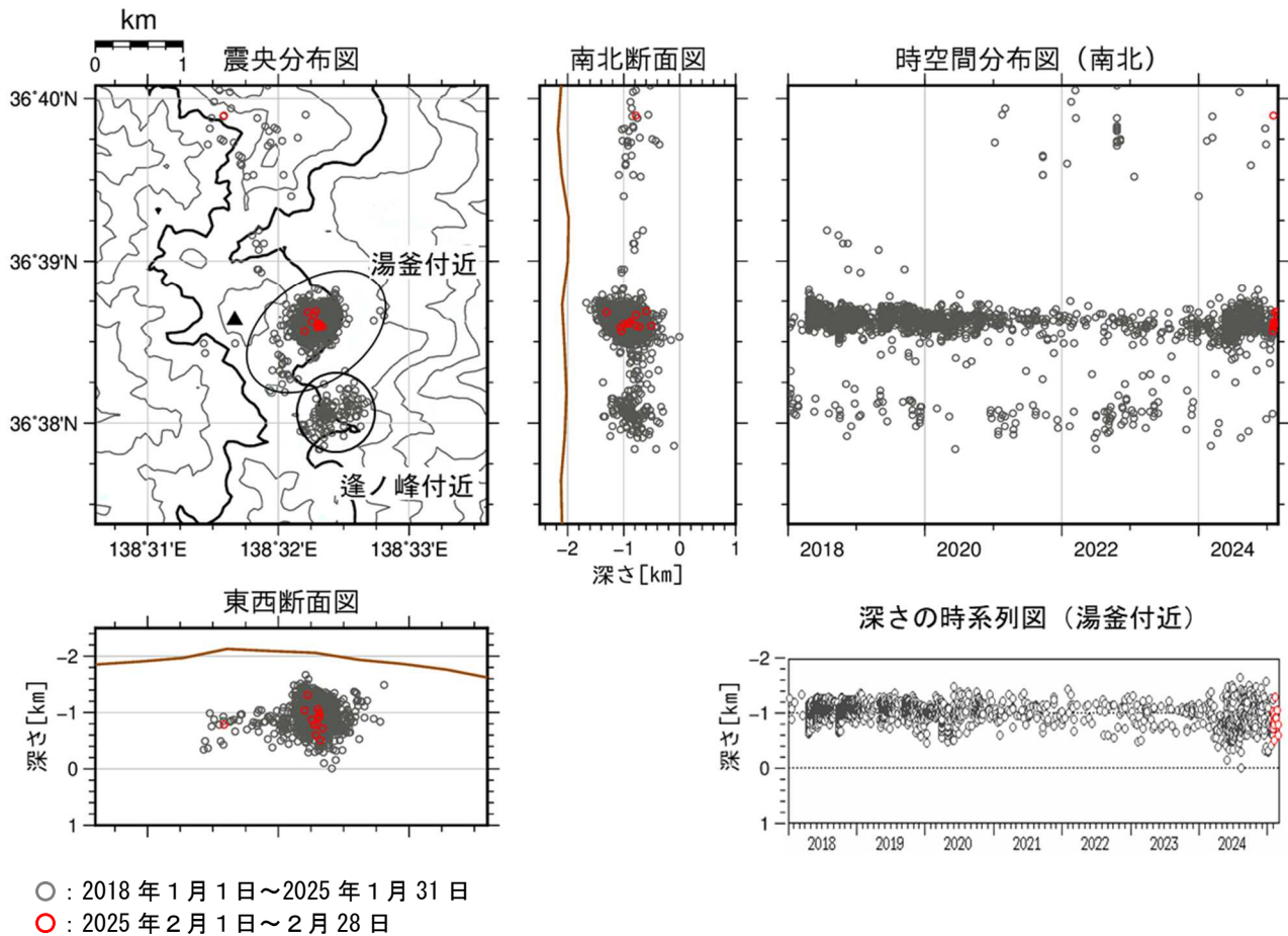
図4 草津白根山 震源分布図（2018 年 1 月 1 日～2025 年 2 月 28 日）
