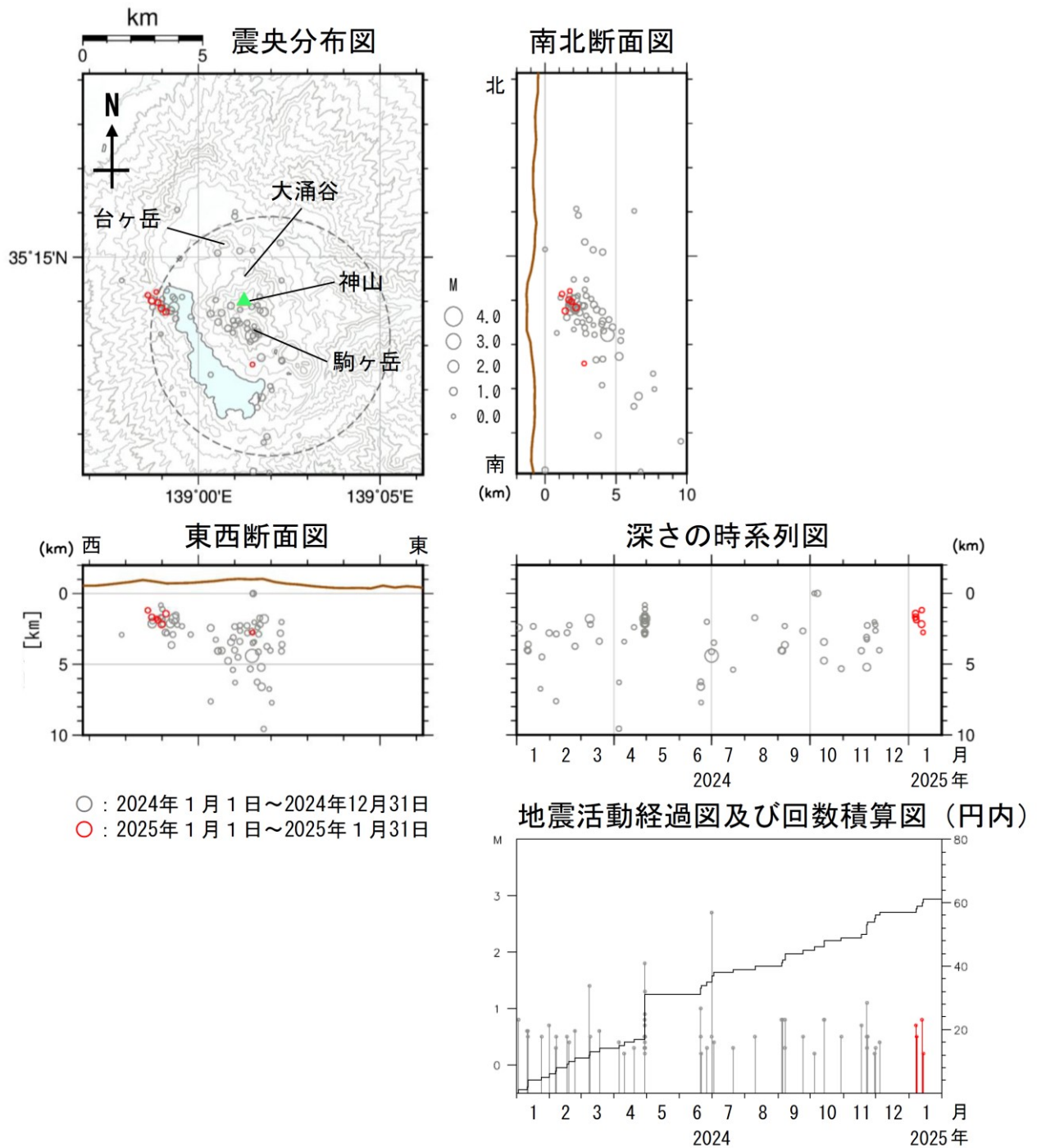
図4 箱根山 広域地震観測網による山体周辺の震源分布図（2024年1月1日～2025年1月31日）
