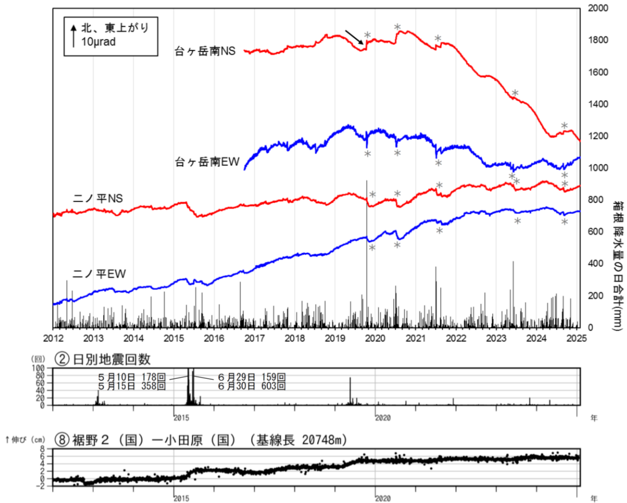
図5 箱根山 傾斜観測及び地震回数・GNSS 観測（2012年1月1日～2025年1月31日）
