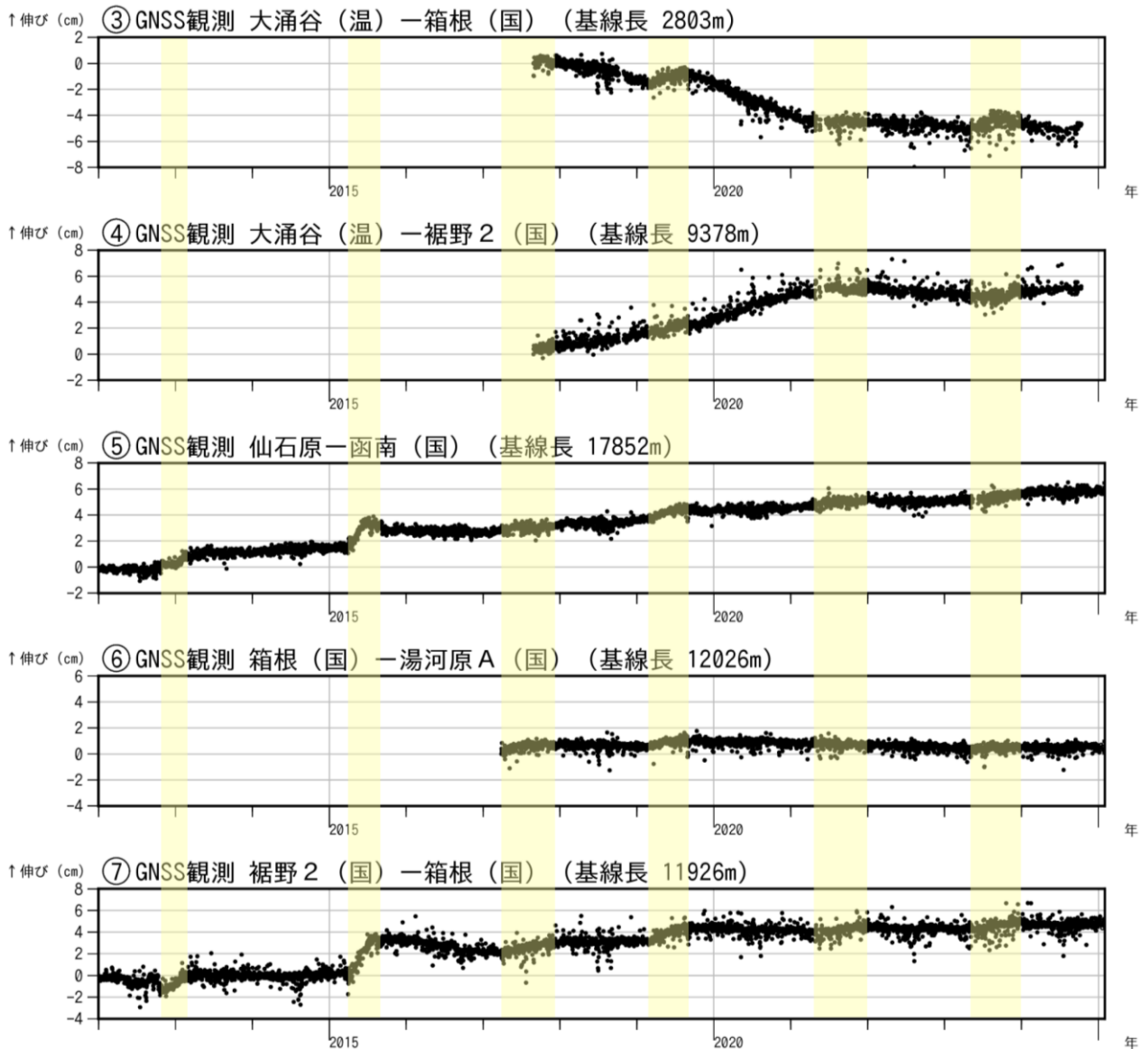
図3-2 箱根山 GNSS 連続観測による 基線長変化及び観測点配置図 (2012年1月1日～2025年1月31日)
