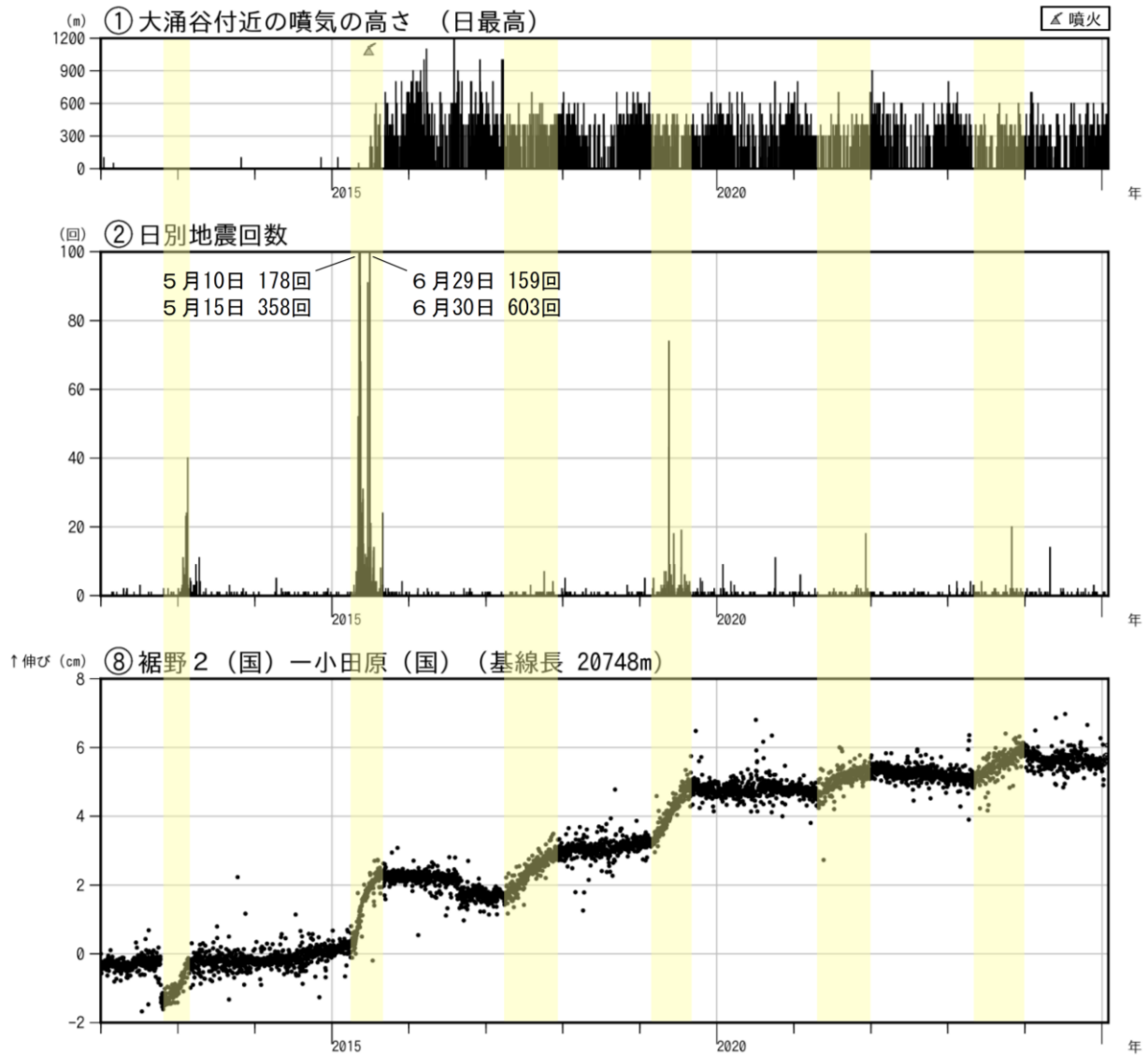
図 3 - 1 箱根山 火山活動経過図（2012 年 1 月 1 日～2025 年 1 月 31 日）
