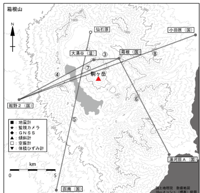
図3-2 箱根山 GNSS 連続観測による 基線長変化及び観測点配置図 (2012年1月1日～2025年1月31日)
