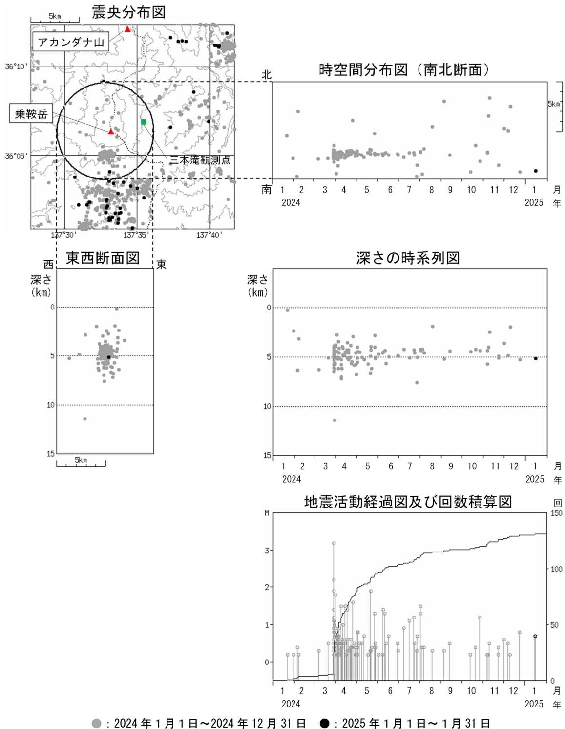
図3 乗鞍岳 広域地震観測網による山体・周辺の地震活動(2024年1月1日～2025年1月31日)
