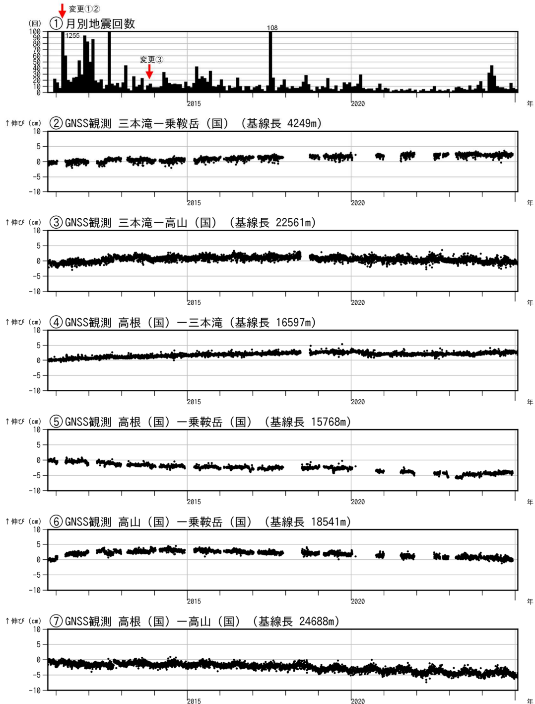
図2 乗鞍岳 火山活動経過図（2010年10月1日～2025年1月31日）
