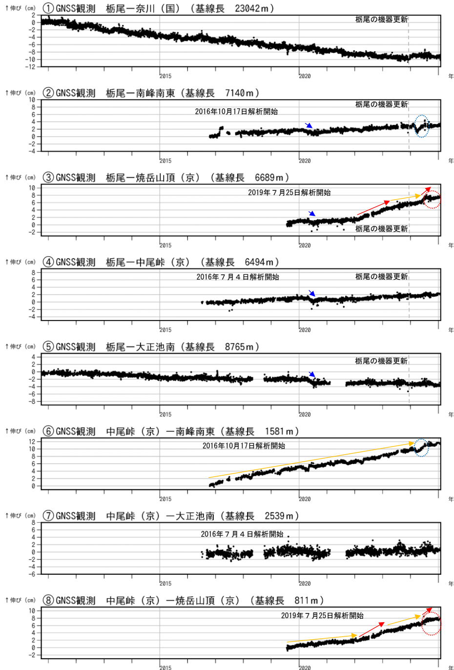
図6 焼岳 GNSS 連続観測による基線長変化（2010年10月1日～2025年1月31日）
