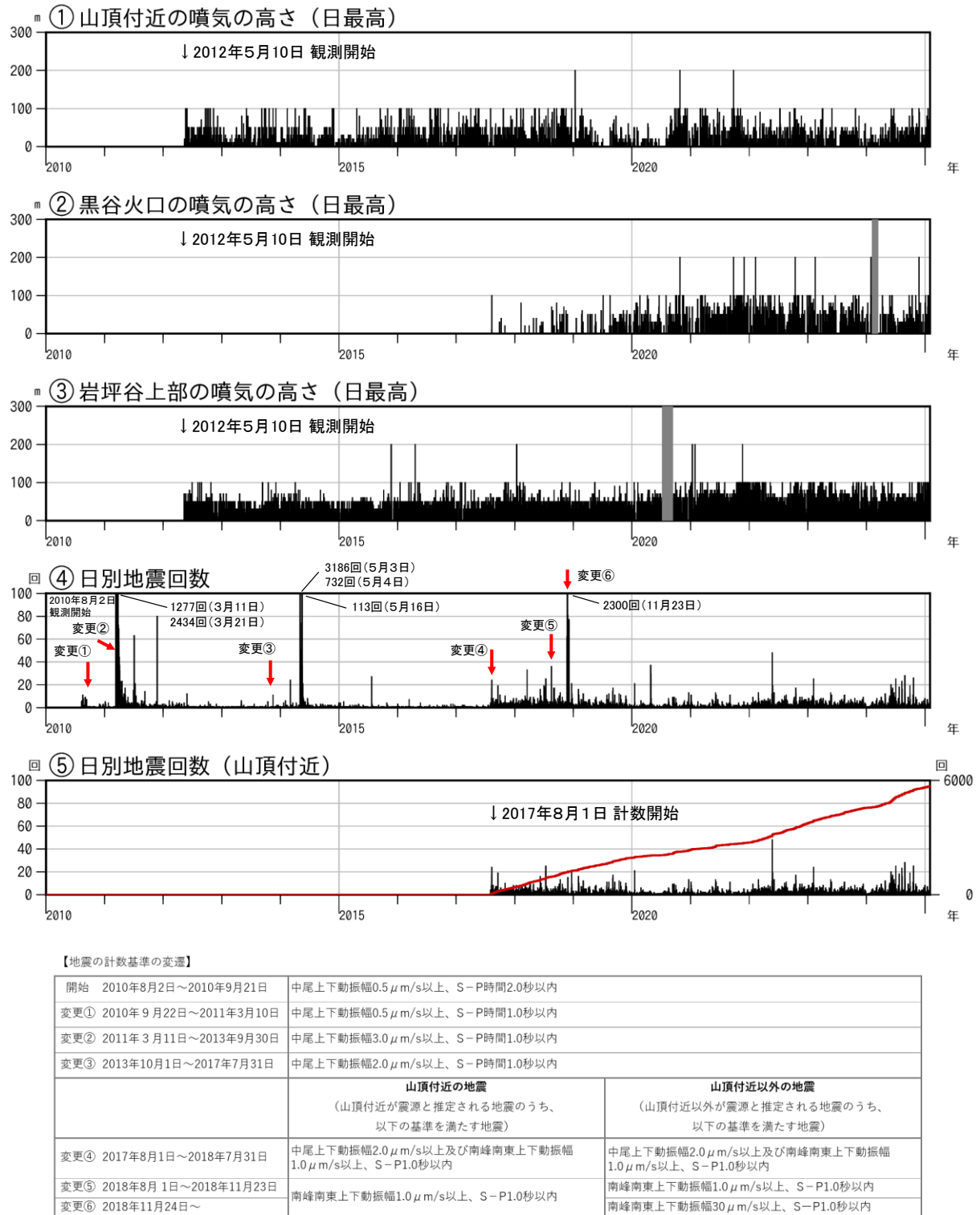
図5 焼岳 噴気の高さと地震回数の推移(2010年8月2日～2025年1月31日)
