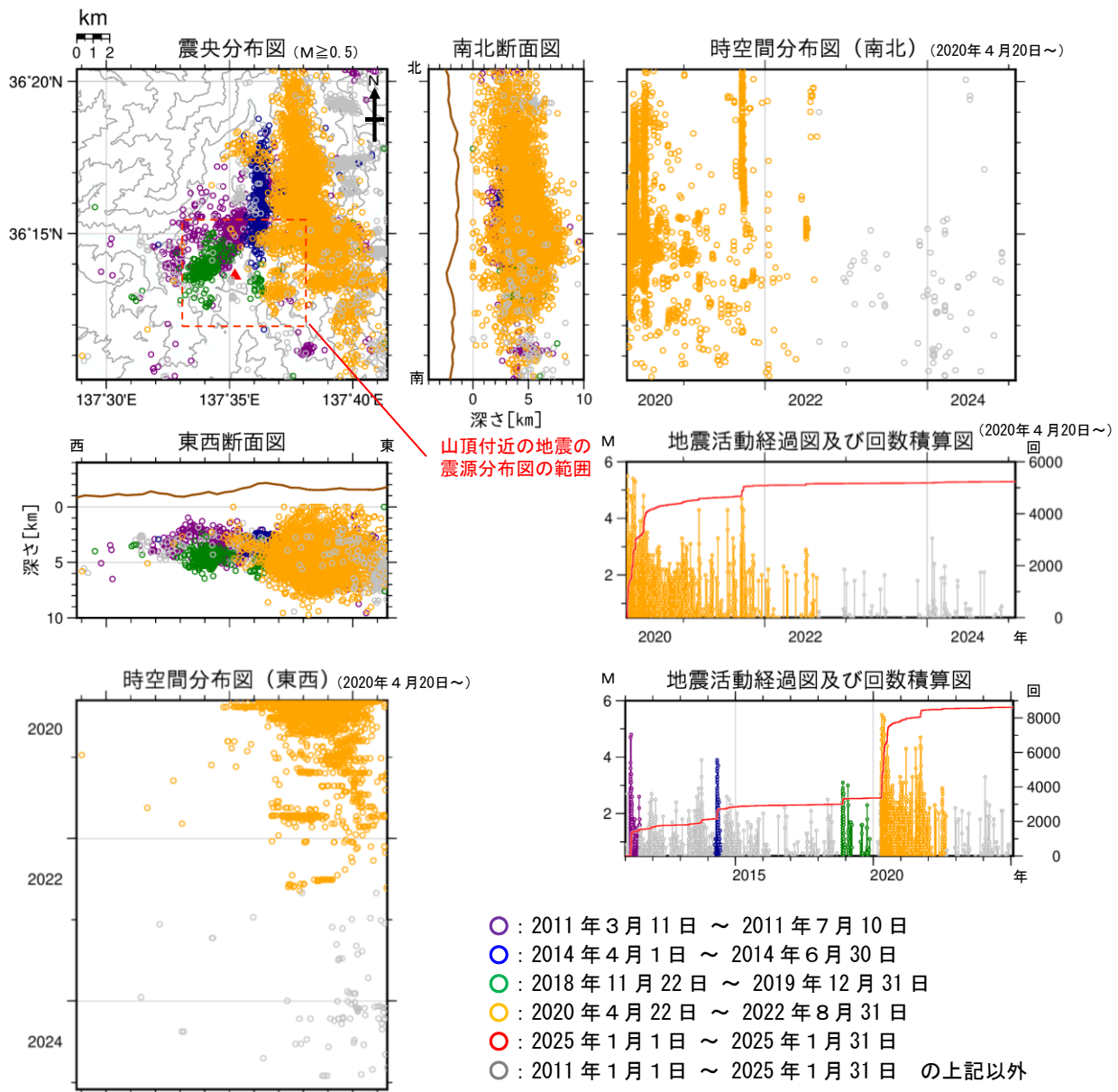
図9 焼岳 広域地震観測網による山体及び周辺の地震活動(2011年1月1日～2025年1月31日)
