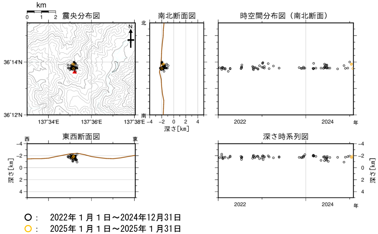
図2 焼岳 山頂付近の地震の震源分布図（2022年1月1日～2025年1月31日）
