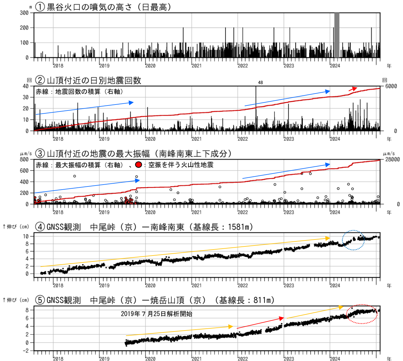
図1 焼岳 火山活動経過図（2017年8月1日～2025年1月31日）
