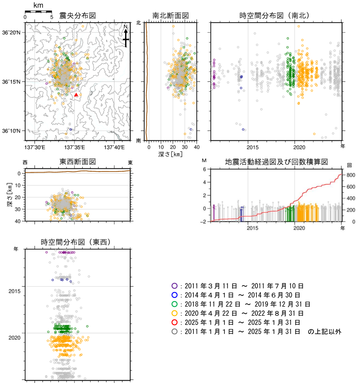
図10 焼岳 広域地震観測網による深部低周波地震の震源分布図（2011年1月1日～2025年1月31日）
