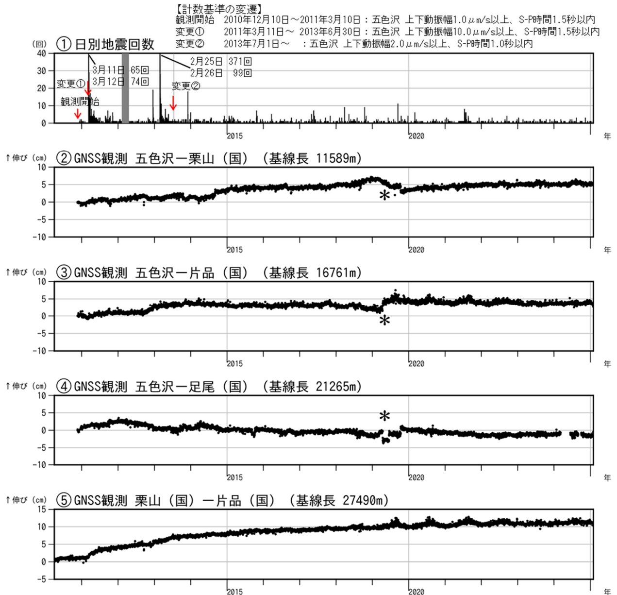
図2 日光白根山 火山活動経過図（2010年4月1日～2025年1月31日）
