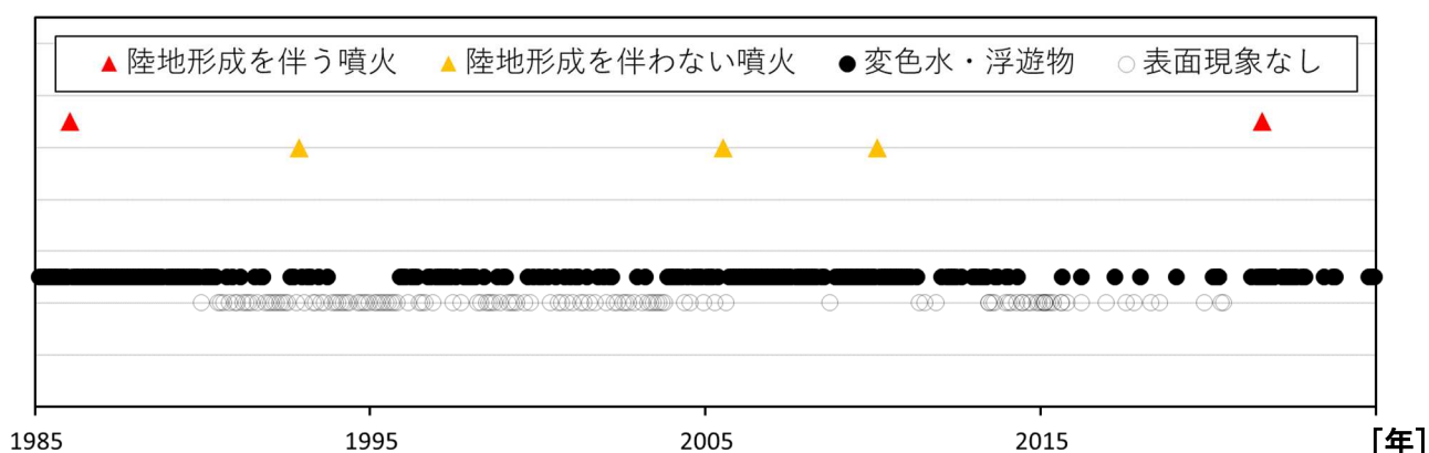
図2 福徳岡ノ場 1985年以降の活動状況
