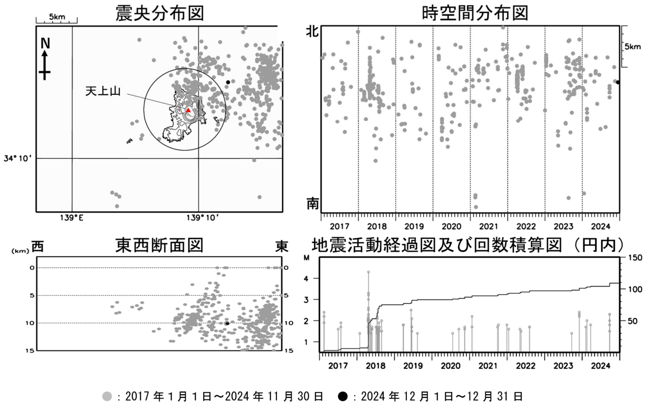
図3 神津島 広域地震観測網による山体・周辺の地震活動（2017年1月1日～2024年12月31日）
