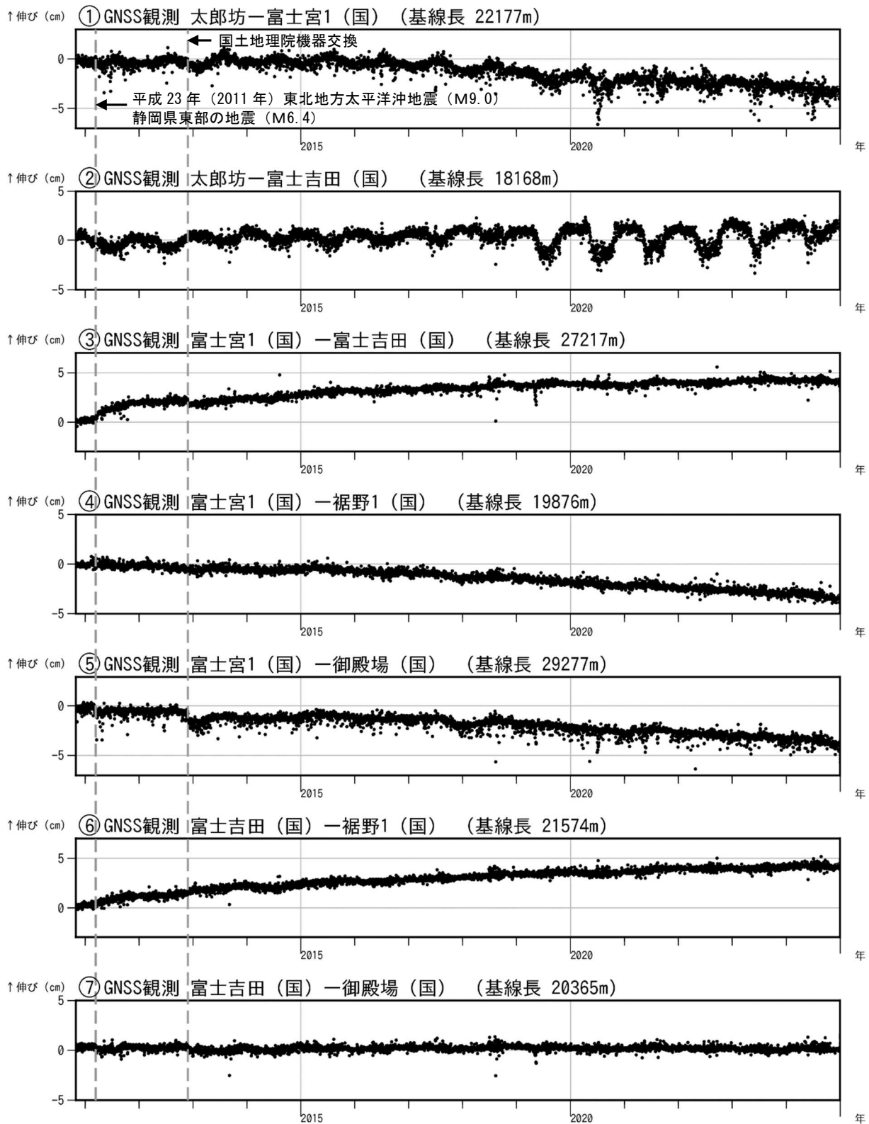
図4 富士山 GNSS 連続観測による基線長変化 (2010 年 10 月 1 日～2024 年 12 月 31 日)
