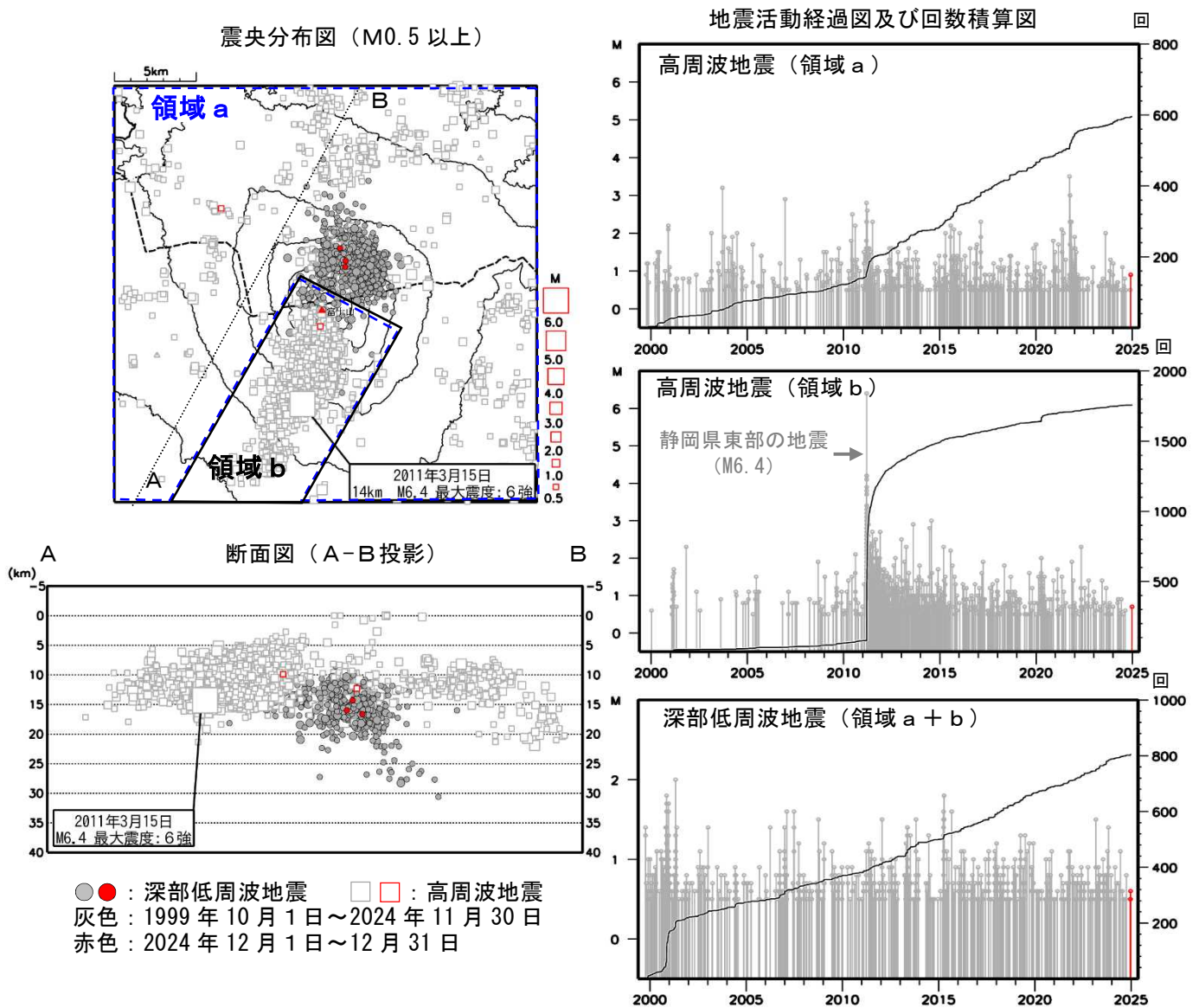
図3 富士山 広域地震観測網による山体及び周辺の地震活動（1999年10月1日～2024年12月31日）
