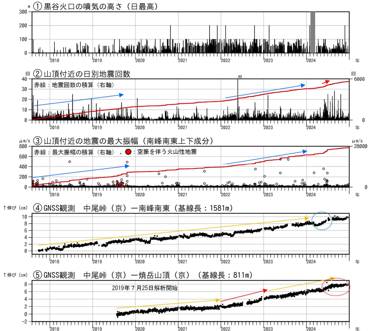
図1-1 焼岳 火山活動経過図（2017年8月1日～2024年12月31日）
