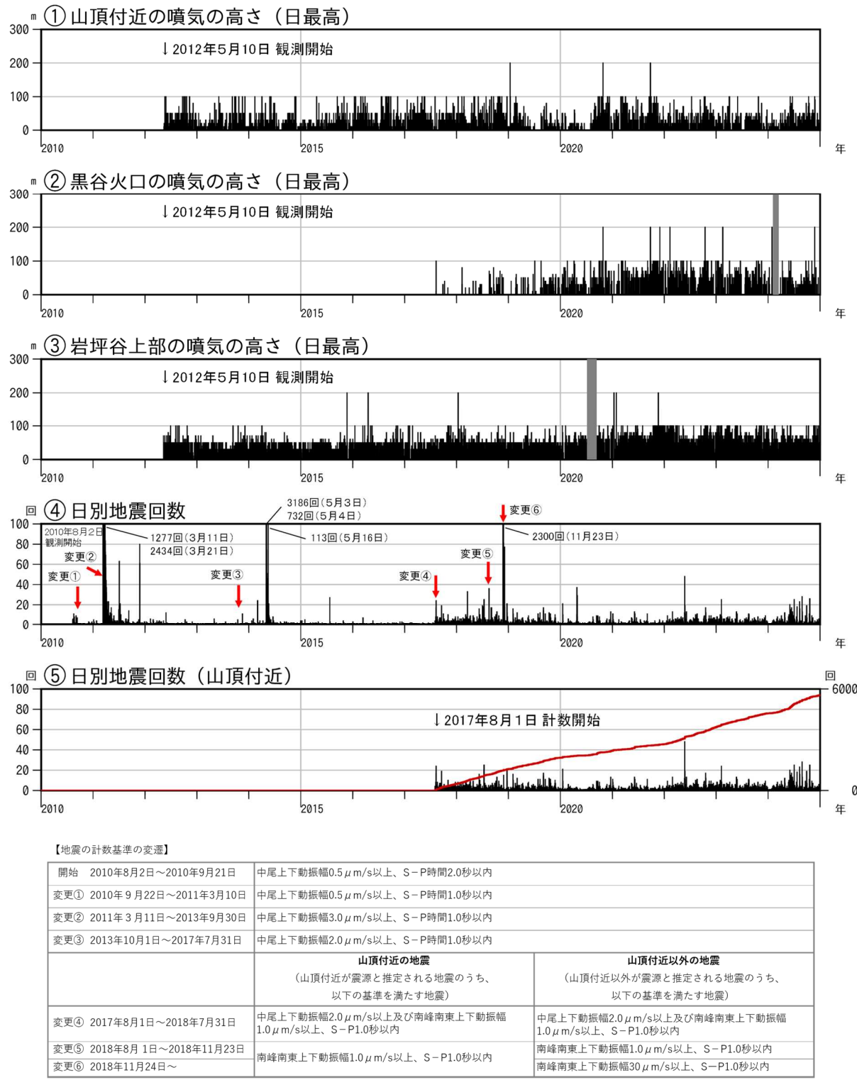
図5 焼岳 噴気の高さと地震回数の推移(2010年8月2日～2024年12月31日) ②黒谷火口の噴気の高さは、2024年2月5日から3月14日にかけて、障害のため欠測（灰色の期間）。 ③岩坪谷上部の噴気の高さは、2020年7月7日から9月10日にかけて、障害のため欠測（灰色の期間）。 ④2017年8月1日以降、山頂付近の地震と山頂付近以外の地震を分けて計数していますが、④ではこれらを合計した回数を示しています。図中の赤矢印は計数基準の変更を示しています。 ⑤山頂付近の日別地震回数（左軸）と日別地震回数の積算（右軸）を示しています。 ・黒谷火口では、2017年夏頃から噴気が時々観測されるようになり、2019年夏頃から噴気を観測する日が増えました。
