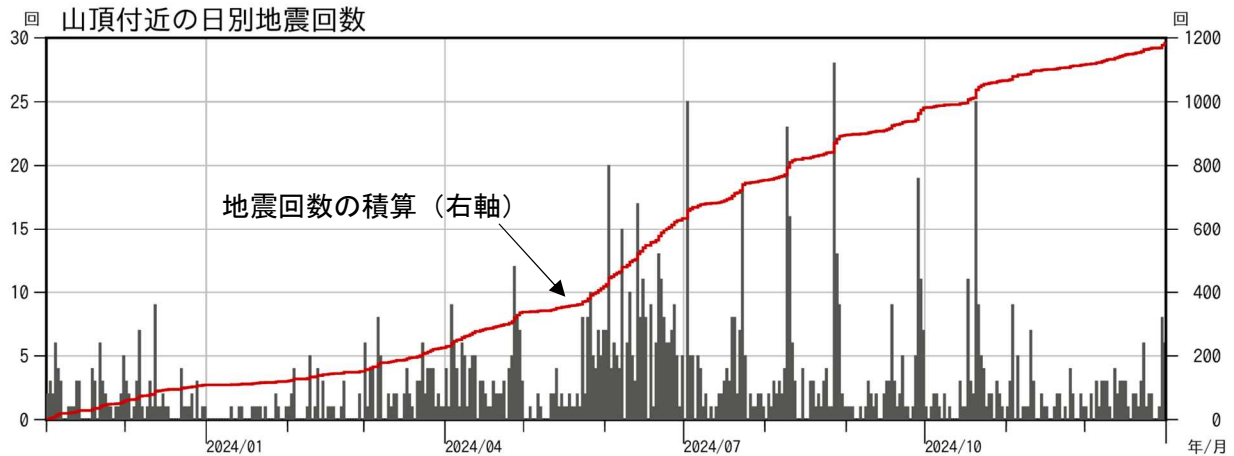
図1-2 焼岳 山頂付近の日別地震回数の推移（2023年11月1日～2024年12月31日）
