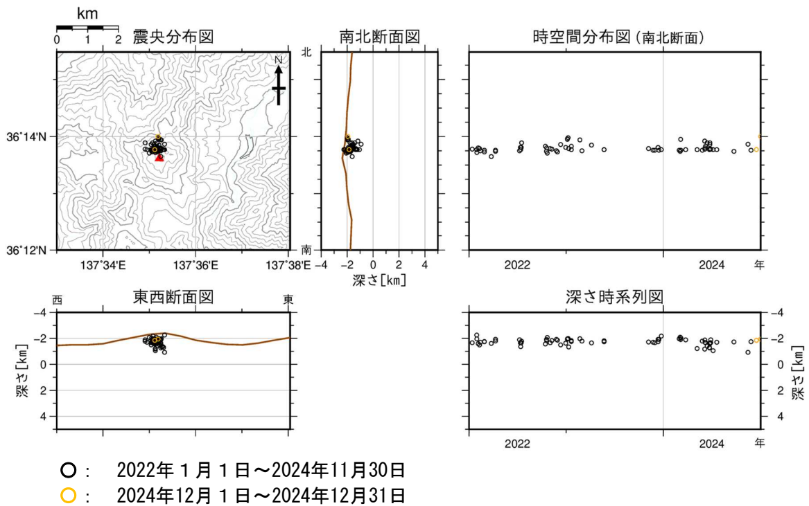
図2 焼岳 山頂付近の地震の震源分布図（2022年1月1日～2024年12月31日）
