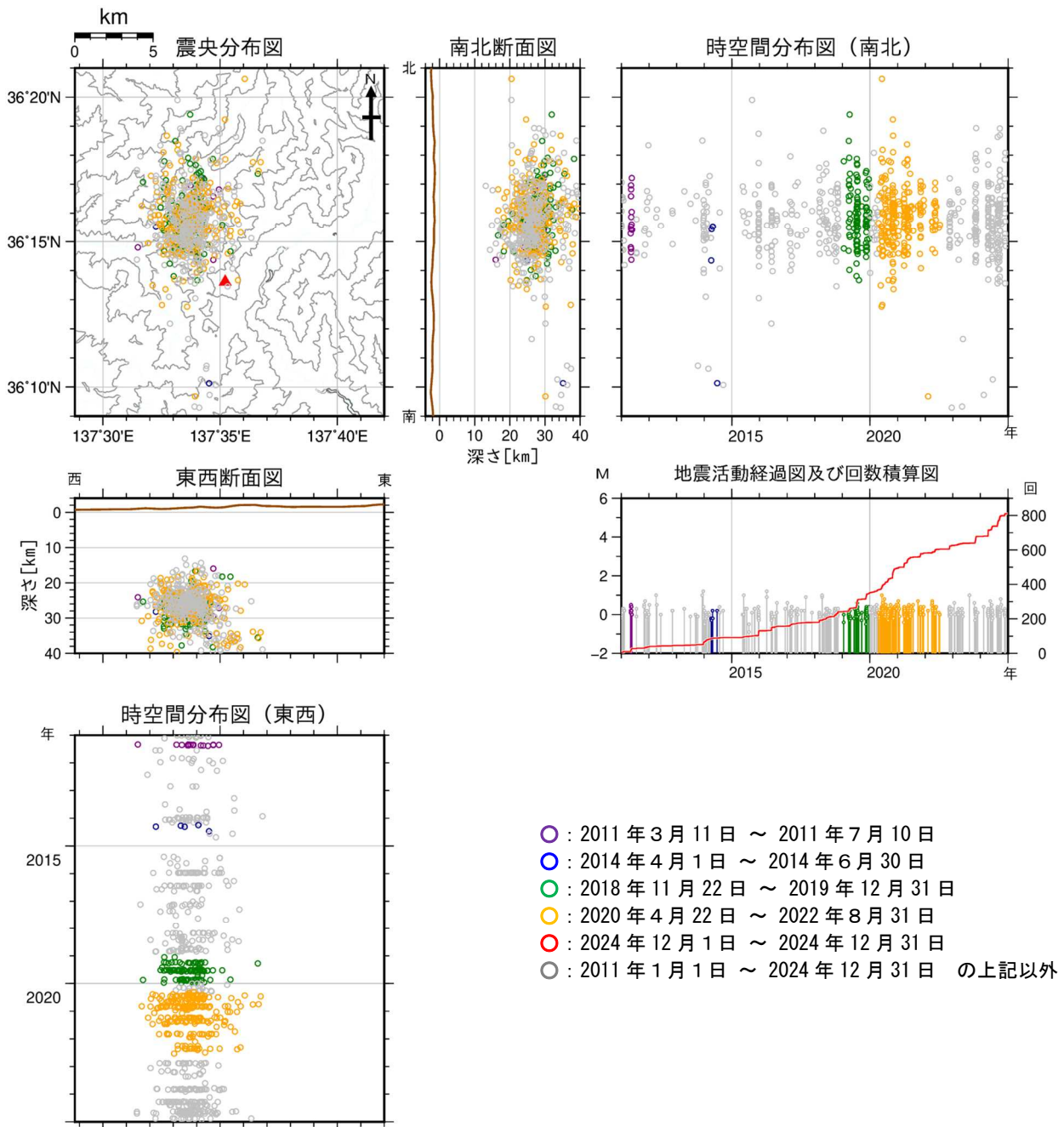
図10 焼岳 広域地震観測網による深部低周波地震の震源分布図（2011年1月1日～2024年12月31日） 広域地震観測網により震源決定したもので、深さは全て海面以下として決定しています。なお、2020年9月以降については、地震観測点の標高を考慮する等、震源決定の手法を変更しております。
