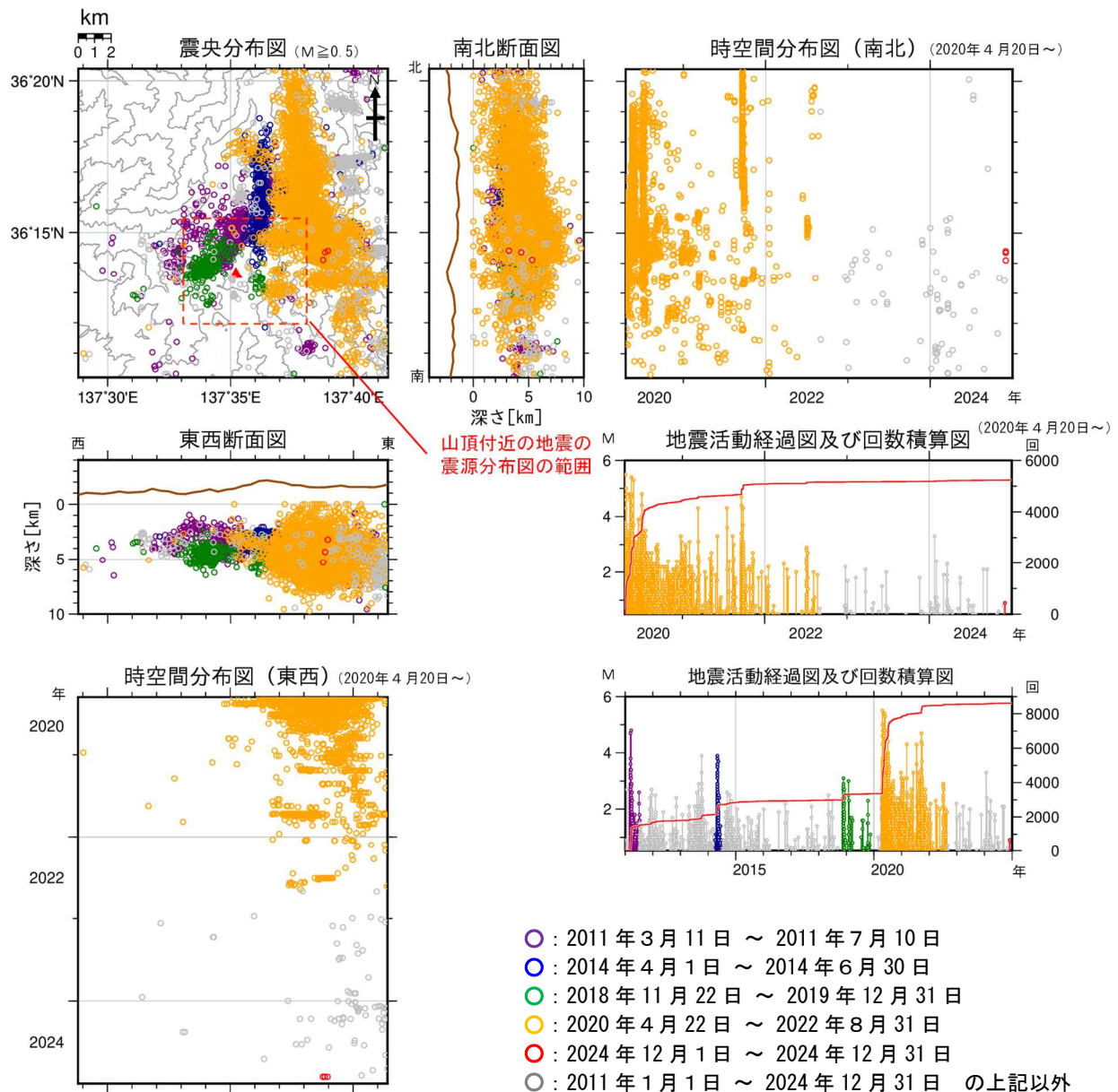
図9 焼岳 広域地震観測網による山体及び周辺の地震活動(2011年1月1日～2024年12月31日)
