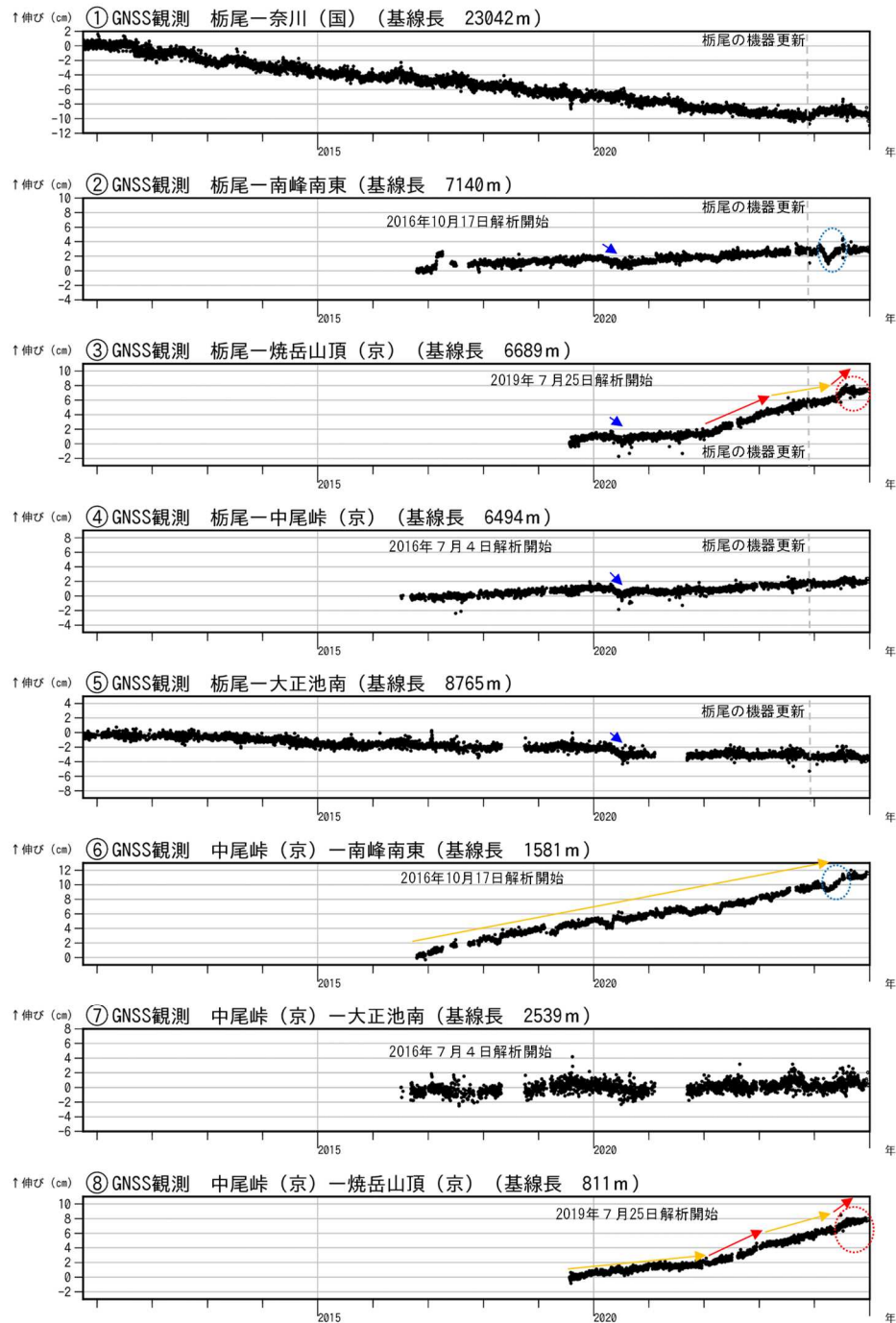
図6 焼岳 GNSS 連続観測による基線長変化（2010年10月1日～2024年12月31日）
