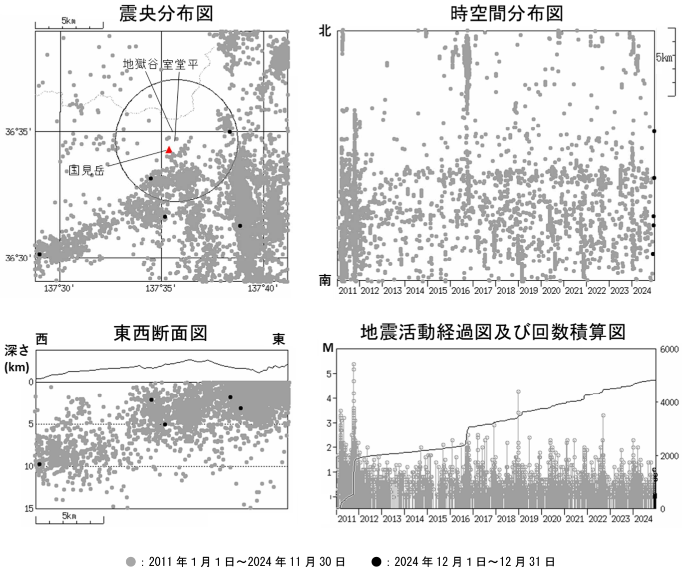
図2 弥陀ヶ原 広域地震観測網による山体・周辺の地震活動（2011 年 1 月 1 日～2024 年 12 月 31 日） 震央分布図中の円は弥陀ヶ原の計数対象地震（室堂平で S-P 時間 1 秒以内）のおよその範囲を示しています。 広域地震観測網により震源決定したもので、深さは全て海面以下として決定しています。なお、2020 年 9 月以降については、地震観測点の標高を考慮する等、震源決定の手法を変更しております。 図中の震源要素は一部暫定値が含まれており、後日変更することがあります。
