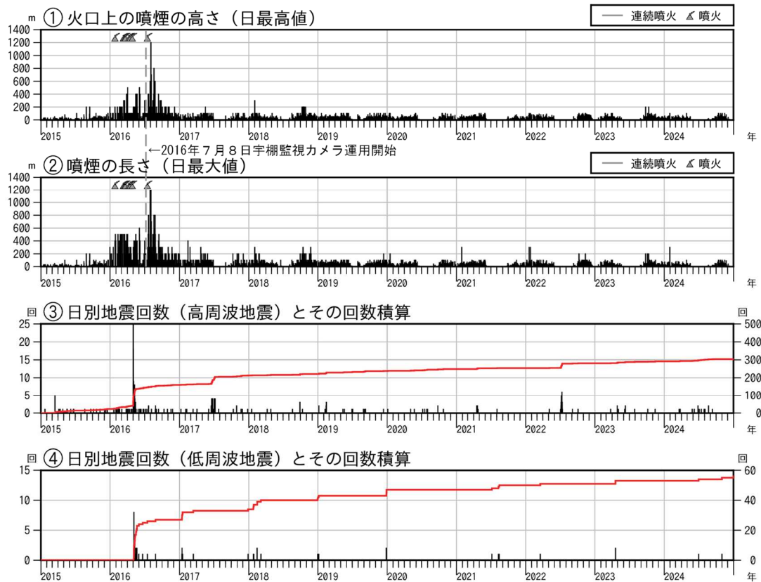
図3 新潟焼山 火山活動経過図（短期）（2015年1月1日～2024年12月31日）
