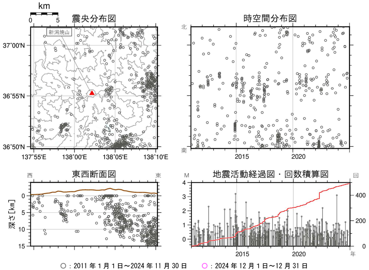
図4 新潟焼山 広域地震観測網による山体・周辺の地震活動（2011年1月1日～2024年12月31日） 広域地震観測網により震源決定したもので、深さは全て海面以下として決定しています。なお、2020年9月以降については、地震観測点の標高を考慮する等、震源決定の手法を変更しております。 図中の震源要素は一部暫定値が含まれており、後日変更することがあります。 ・新潟焼山周辺を震源とする地震活動は低調に経過しました。
