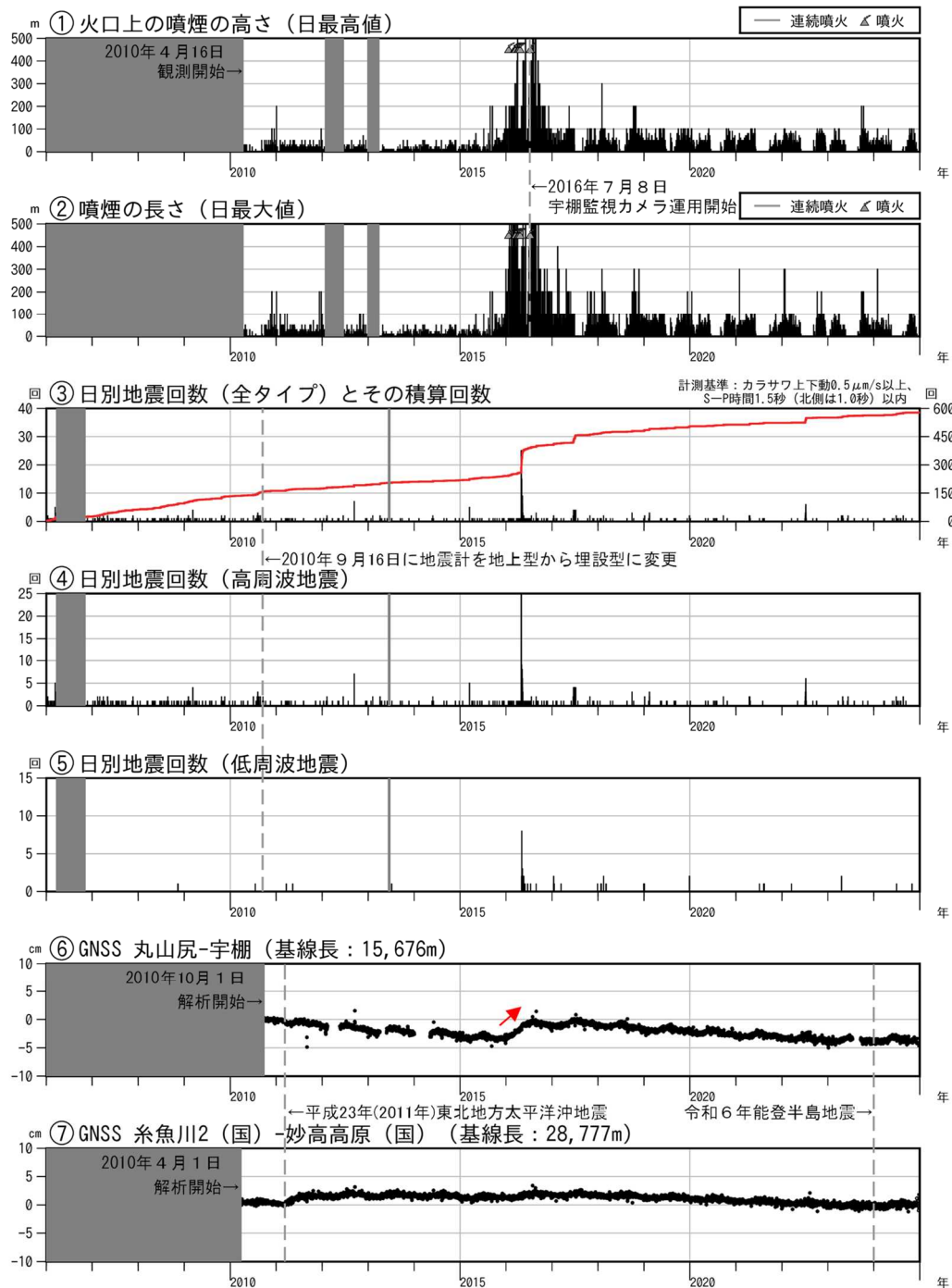
図2 新潟焼山 火山活動経過図（2006年1月1日～2024年12月31日）
