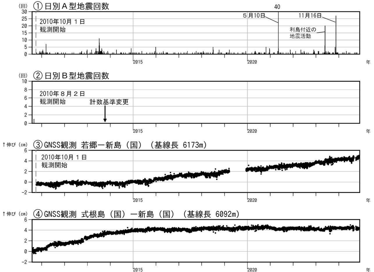
図2 新島 火山活動経過図(2010年8月2日～2024年11月30日)
