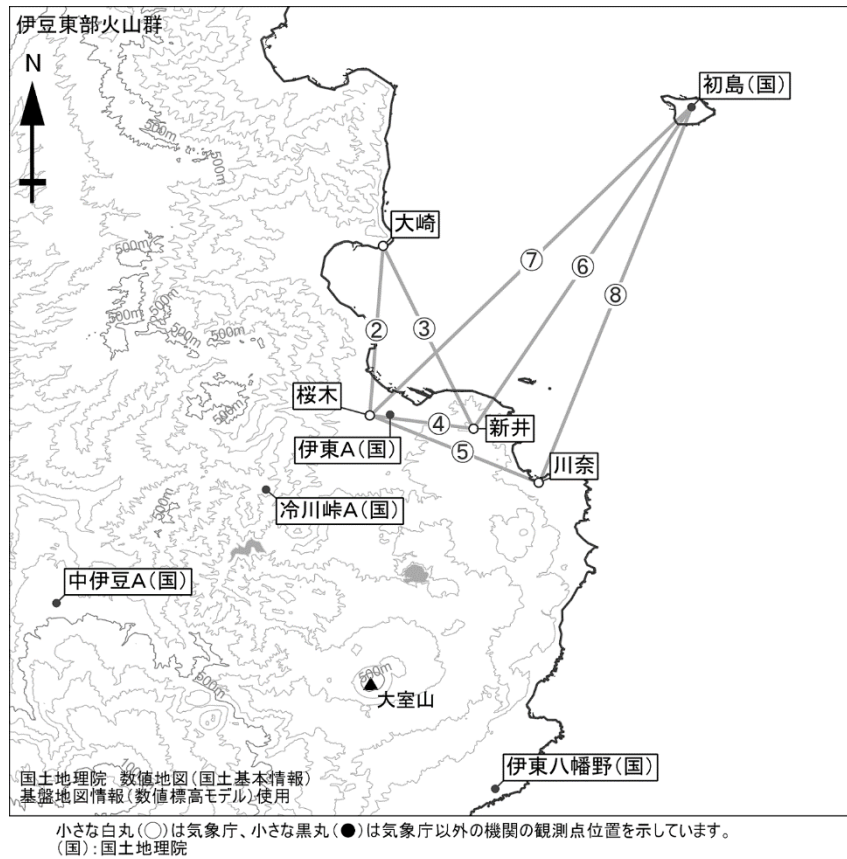
図4 伊豆東部火山群 GNSS 連続観測点配置図
