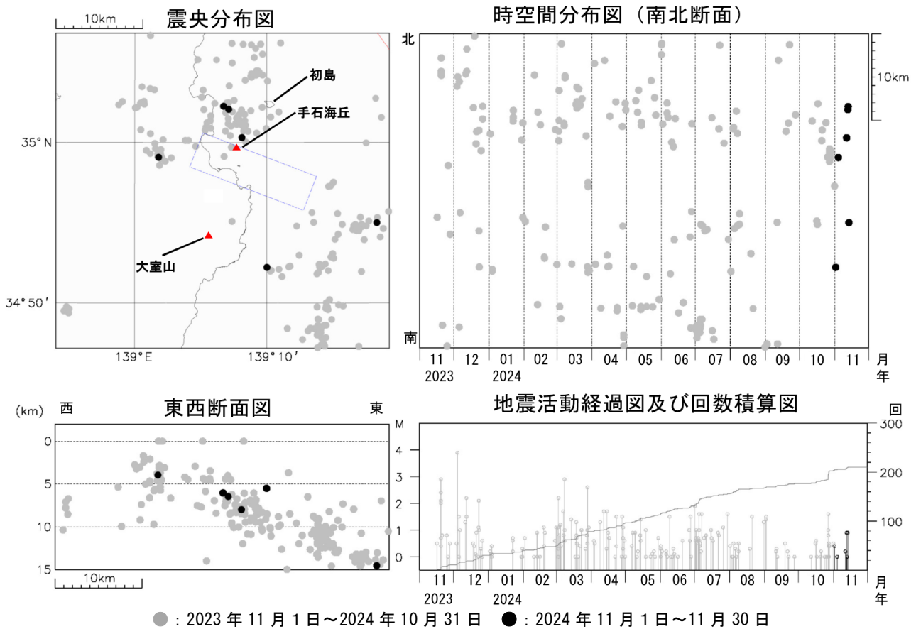
図2 伊豆東部火山群 広域地震観測網による震源分布図（2023 年 11 月 1 日～2024 年 11 月 30 日） □ の領域は群発地震活動の発生する可能性がある範囲（火口が出現する可能性のある範囲）を示しています。 https://www.data.jma.go.jp/vois/data/filing/level/PDF/level_316.pdf 広域地震観測網により震源決定したもので、深さは全て海面以下として決定しています。 M（マグニチュード）は地震の規模を表し、M0.0 以上を表示しています。 図中の震源要素は一部暫定値が含まれており、後日変更することがあります。 この図では、関係機関の地震波形を一元的に処理し、地震観測点の標高を考慮する等した手法で得られた震源を用いています。
