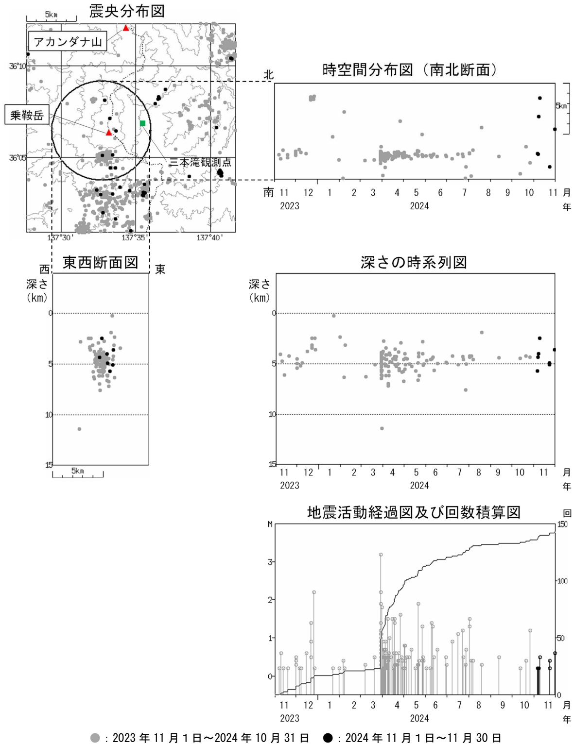
図3 乗鞍岳 広域地震観測網による山体・周辺の地震活動(2023 年 11 月 1 日～2024 年 11 月 30 日) M (マグニチュード) は地震の規模を表し、M0.2 以上の地震を表示しています。 広域地震観測網により震源決定したもので、深さは全て海面以下として決定しています。なお、2020 年 9 月以降については、地震観測点の標高を考慮する等、震源決定の手法を変更しております。図中の震源要素は一部暫定値が含まれており、後日変更することがあります。 東西断面図、時空間分布図、深さの時系列図、地震活動経過図及び回数積算図には、乗鞍岳付近（震央分布図中の黒線円の範囲）の地震を示しています。 ・ 3 月 29 日の乗鞍岳の南 2 km 付近を震源とする地震の発生以降、地震回数が増加していましたが、6 月以降はこの地震発生以前の地震回数と同程度となっています。
