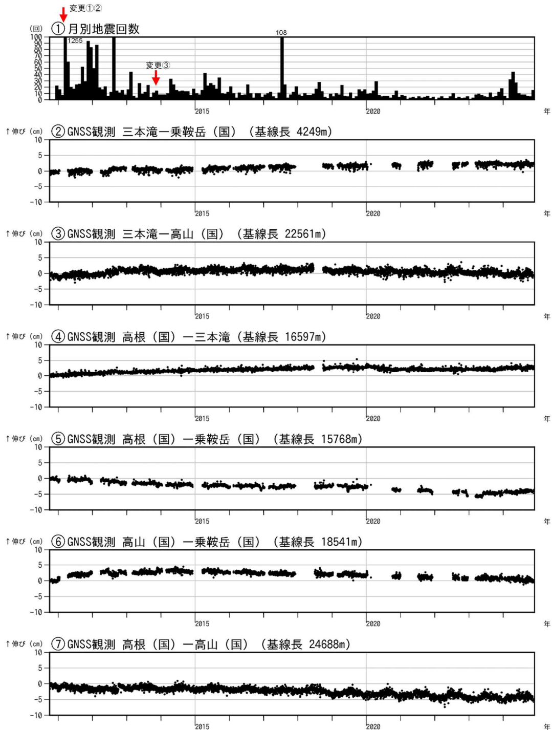
図2 乗鞍岳 火山活動経過図（2010年10月1日～2024年11月30日）
