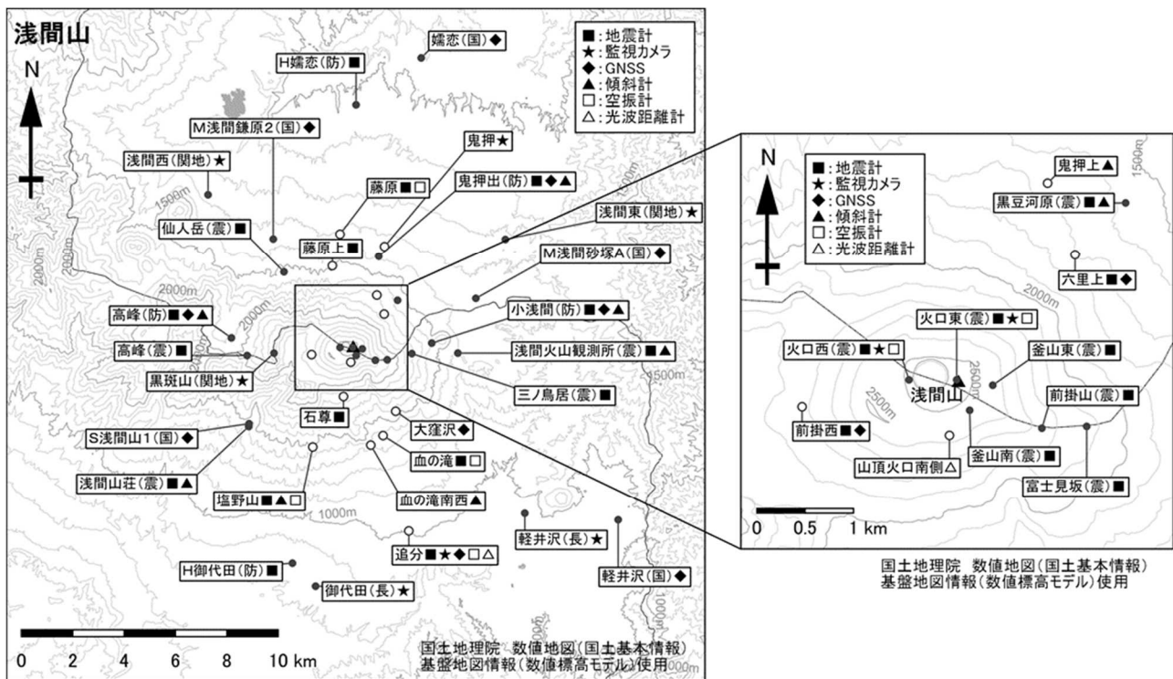
図 10 浅間山 観測点配置図
