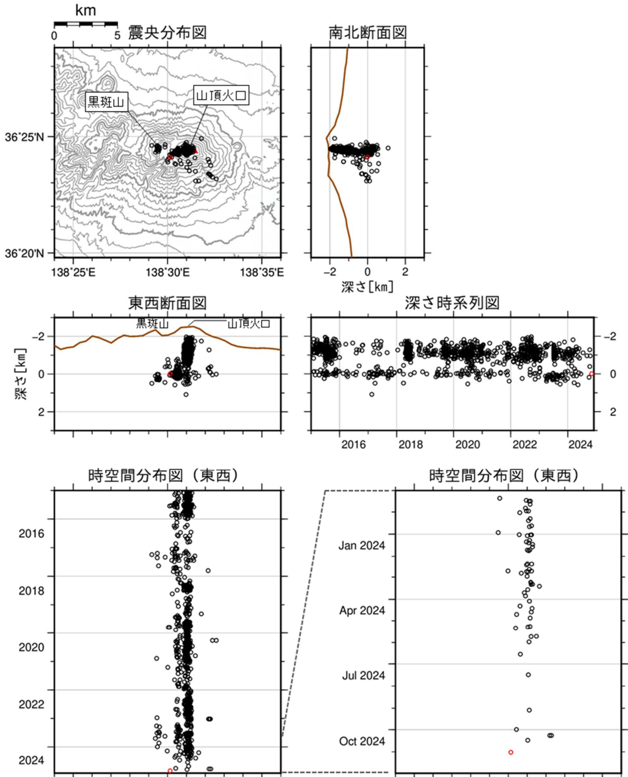
図6 浅間山 震源分布図（2015年1月1日～2024年11月30日）
