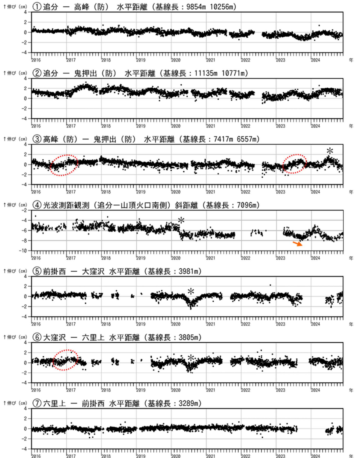
図8-1 浅間山 GNSS 連続観測及び光波測距観測結果(2016年1月1日~2024年11月30日)
