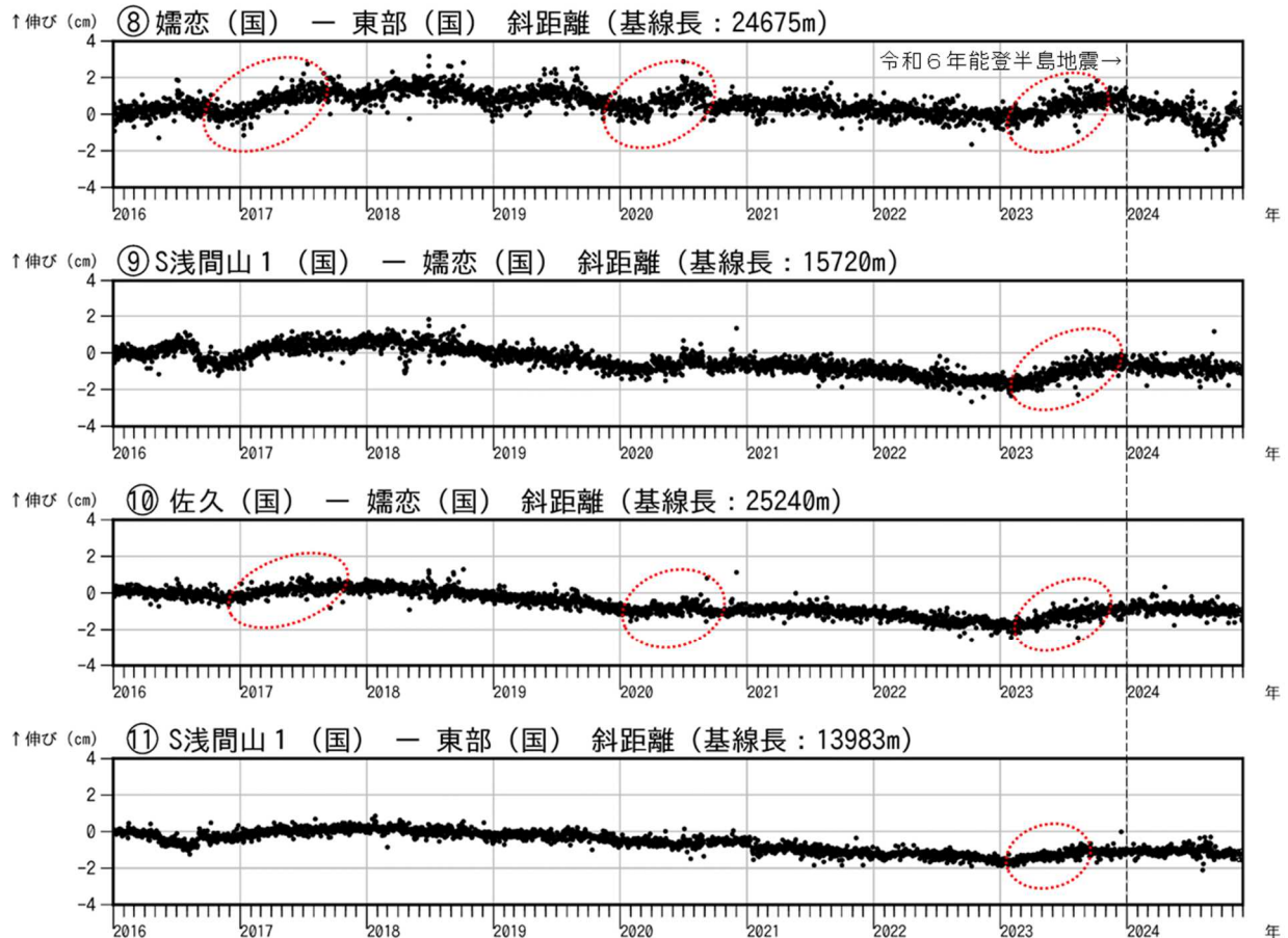
図8-2 浅間山 GNSS 連続観測結果(2016年1月1日～2024年11月30日)
