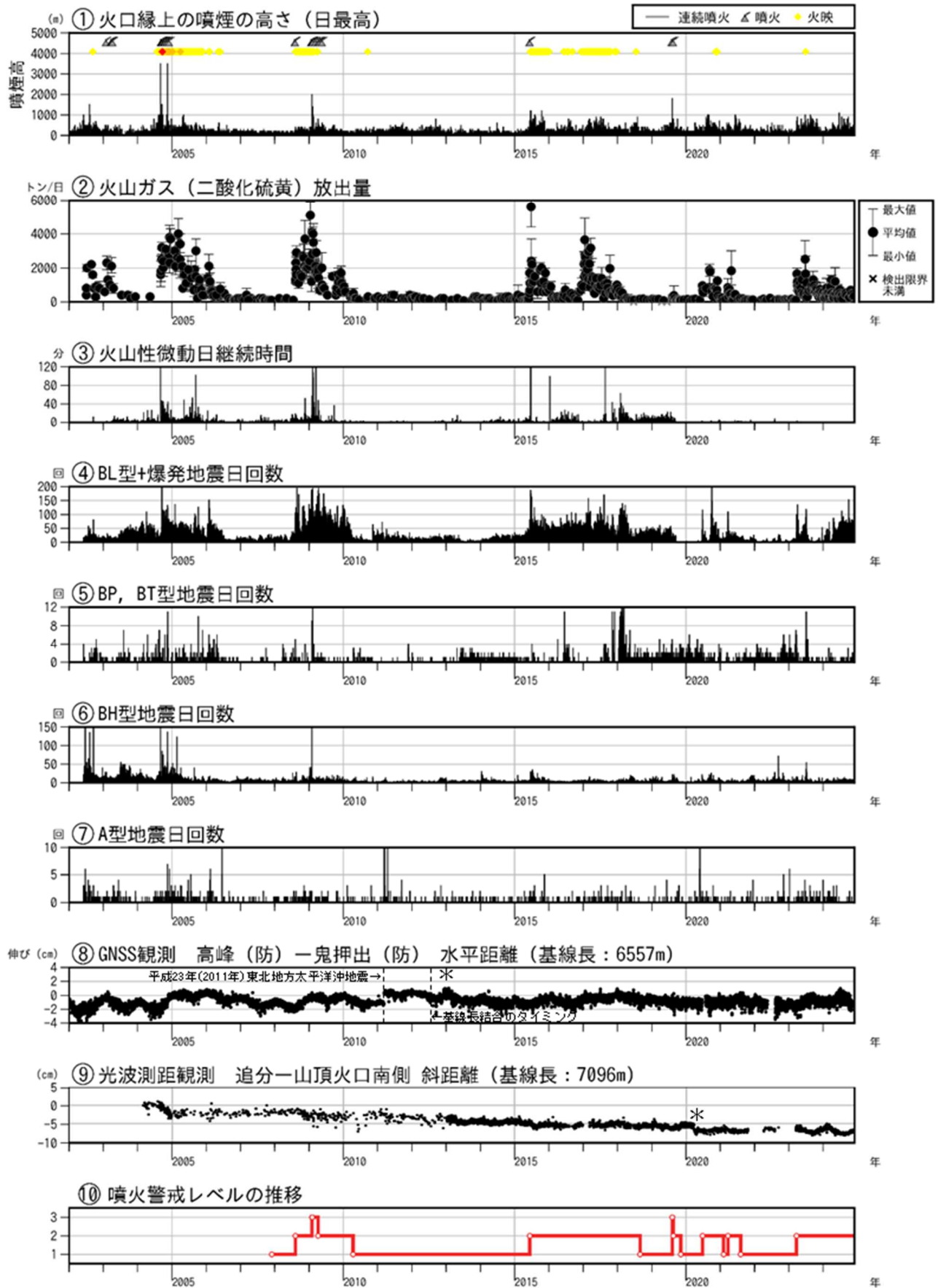
図4 浅間山 長期火山活動経過図（2002年1月1日～2024年11月30日）
