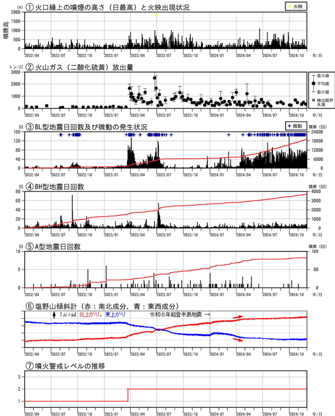
図3 浅間山 短期火山活動経過図（2022年4月1日～2024年11月30日）
