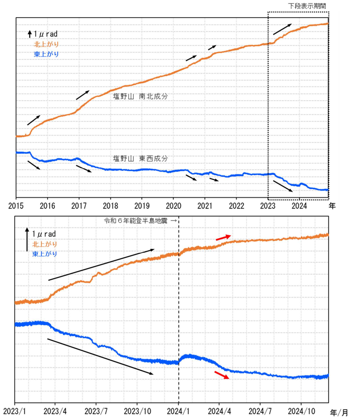
図7 浅間山 塩野山観測点における傾斜データ（2015年1月1日～2024年11月30日）
