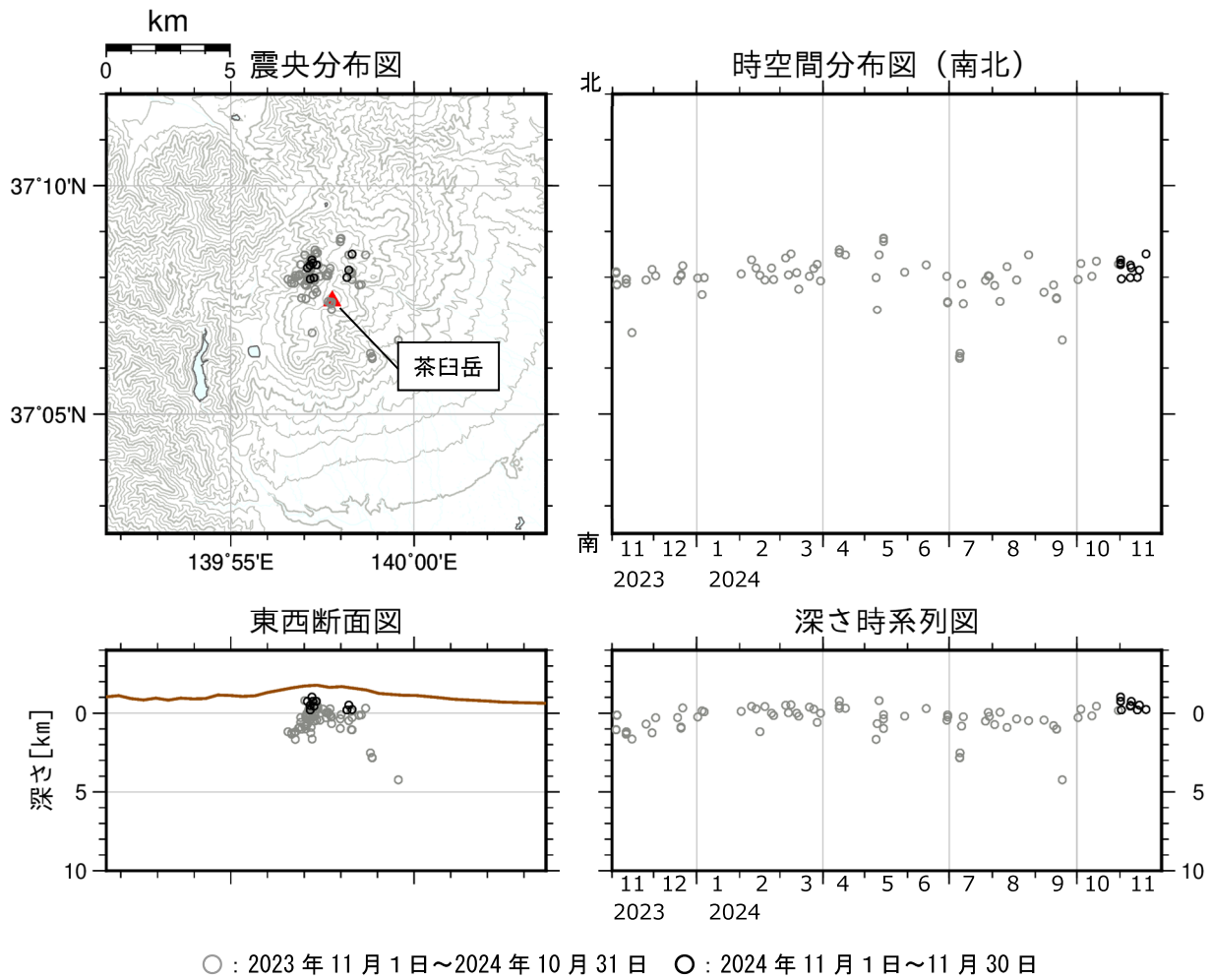
図5 那須岳 震源分布図（2023 年 11 月 1 日～2024 年 11 月 30 日）
