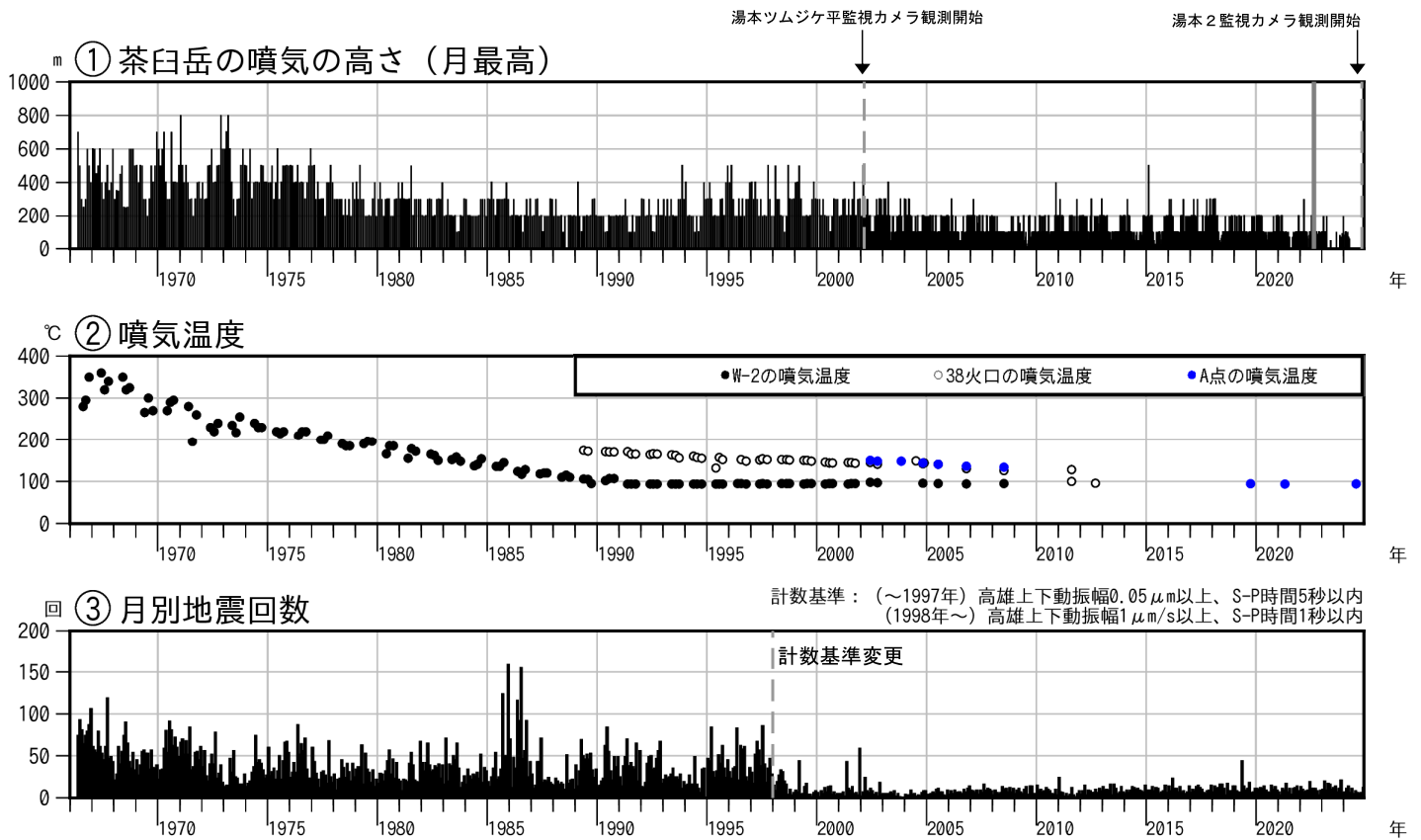
図3-1 那須岳 火山活動経過図（1966年6月～2024年11月）
