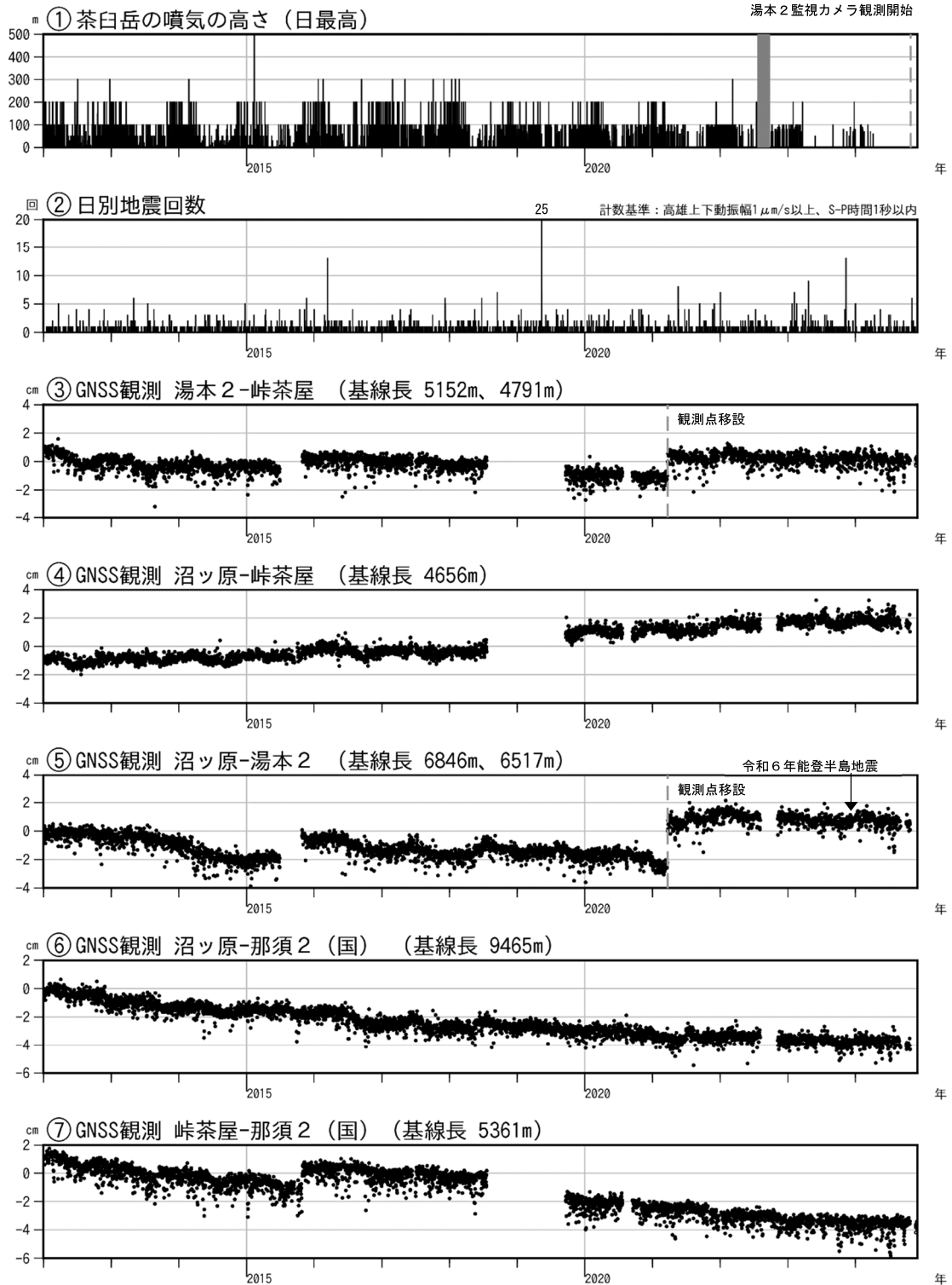
図4 那須岳 火山活動経過図（2012年1月1日～2024年11月30日）
