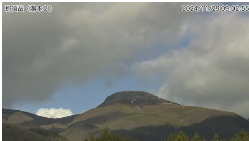
図1 那須岳 茶臼岳の状況（11月29日、湯本2監視カメラによる）
