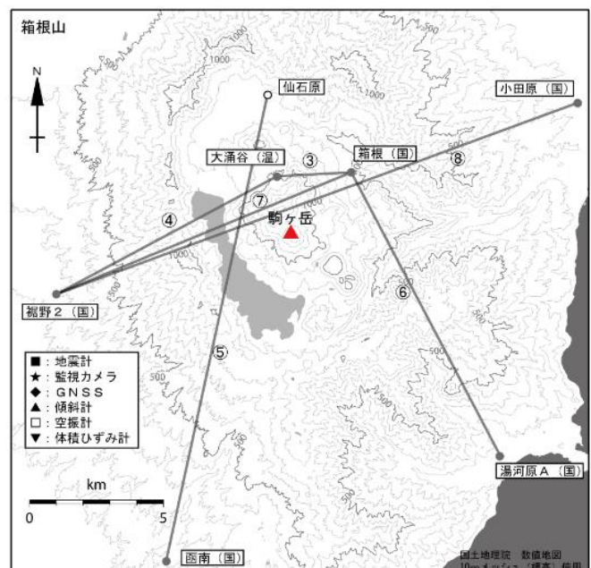
図 3-2 箱根山 GNSS 連続観測による 基線長変化及び観測点配置図 (2012 年 1 月 1 日～2024 年 10 月 31 日) (国)：国土地理院 (温)：神奈川県温泉地学研究所 空白部分は欠測を示します。
