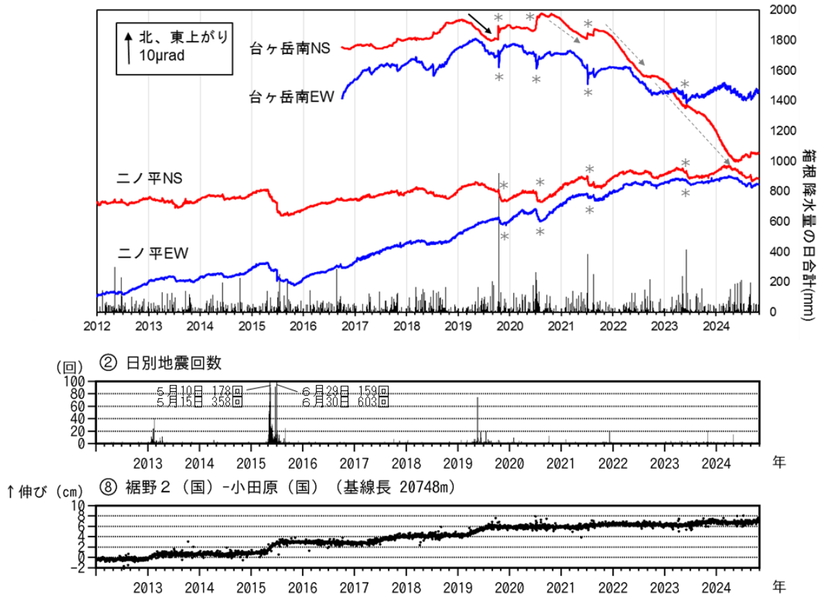
図5 箱根山 傾斜観測及び地震回数・GNSS 観測 (2012 年 1 月 1 日～2024 年 10 月 31 日)
