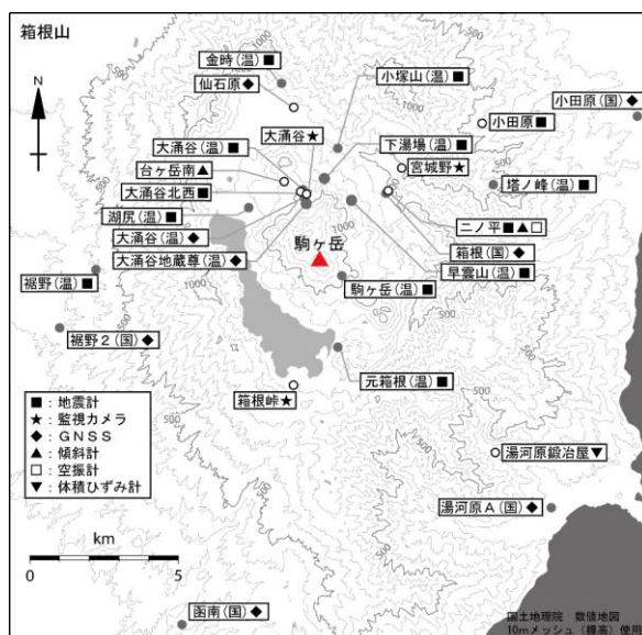
図6 箱根山 観測点配置図
