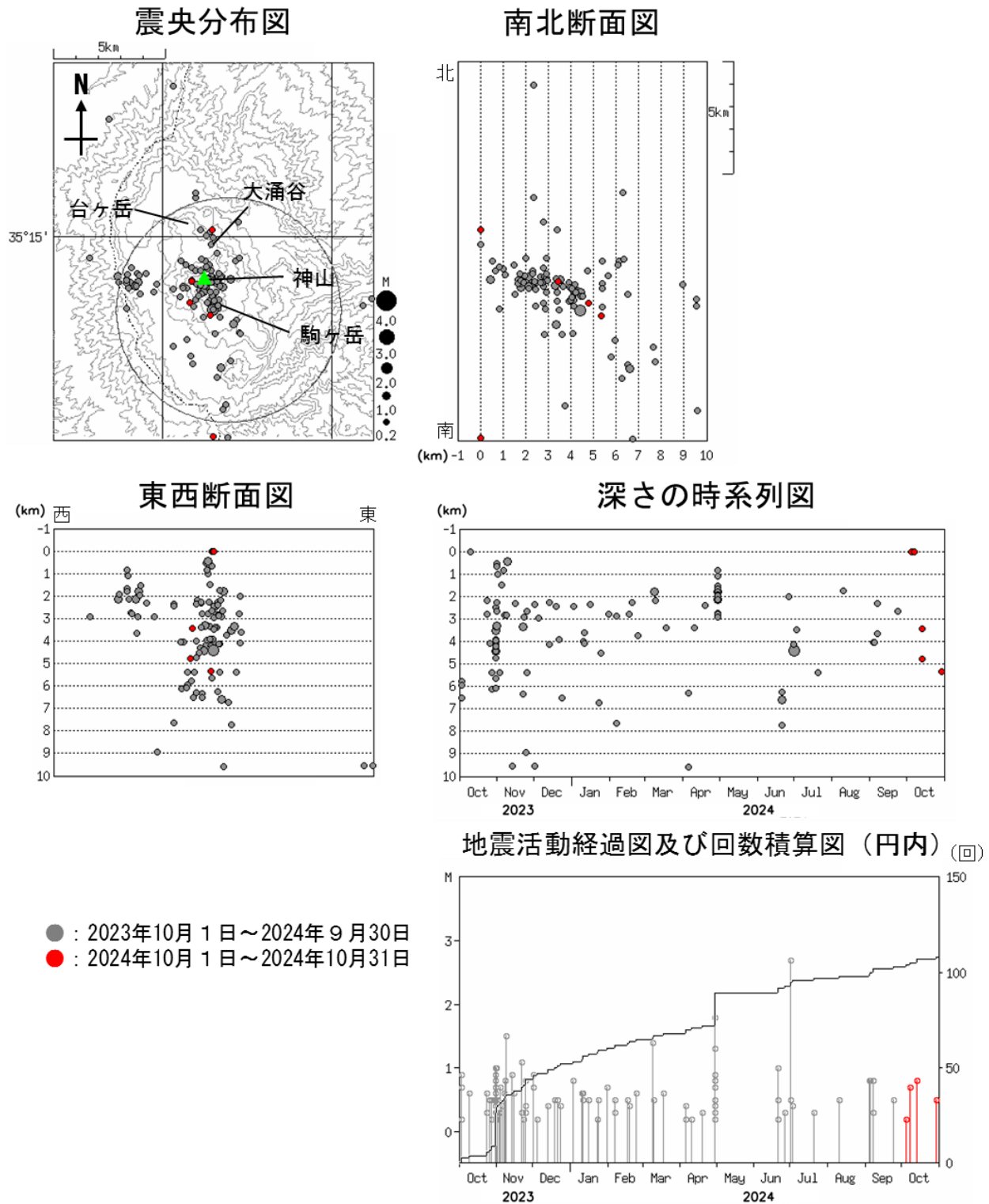
図4 箱根山 広域地震観測網による山体周辺の震源分布図（2023年10月1日～2024年10月31日）
