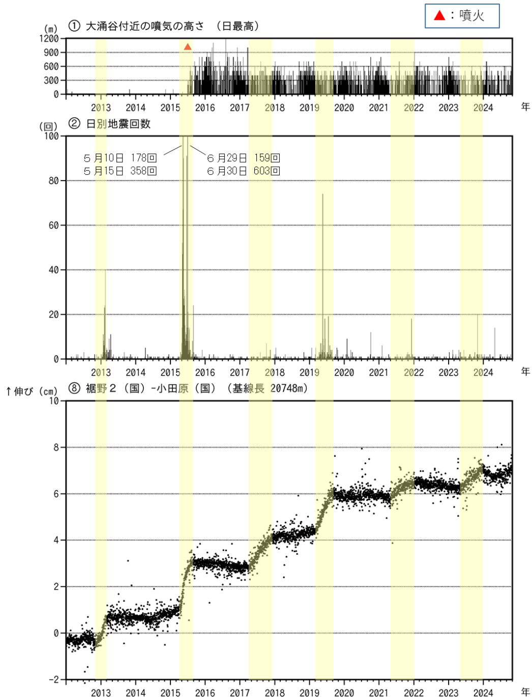
図3-1 箱根山 火山活動経過図（2012年1月1日～2024年10月31日）
