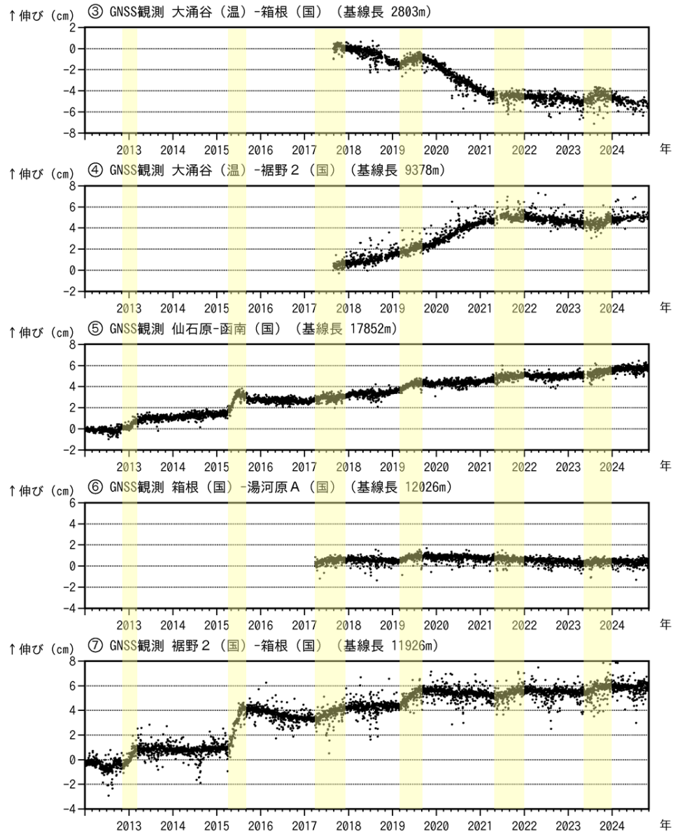
図 3-2 箱根山 GNSS 連続観測による 基線長変化及び観測点配置図 (2012 年 1 月 1 日～2024 年 10 月 31 日) (国)：国土地理院 (温)：神奈川県温泉地学研究所 空白部分は欠測を示します。
