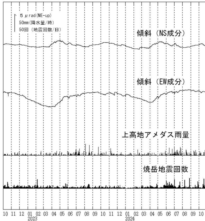
図8 焼岳 南峰南東観測点における傾斜データ（2022年10月1日～2024年10月31日）
