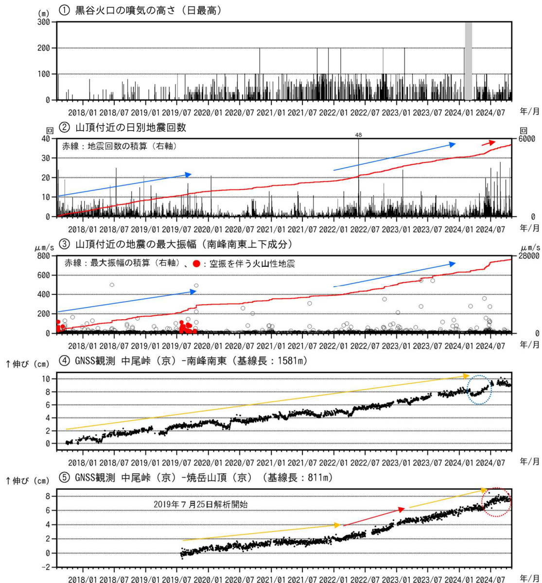
図1-1 焼岳 火山活動経過図（2017年8月1日～2024年10月31日）
