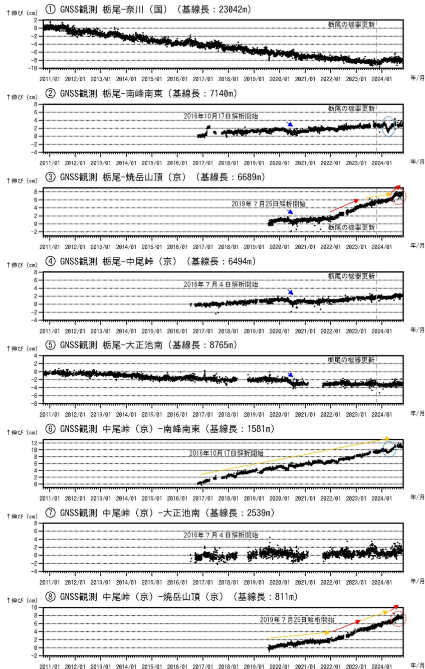
図6 焼岳 GNSS 連続観測による基線長変化（2010年10月1日～2024年10月31日）
