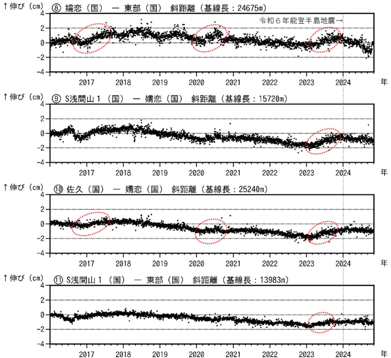
図7-2 浅間山 GNSS 連続観測結果(2016年1月1日～2024年10月31日)
