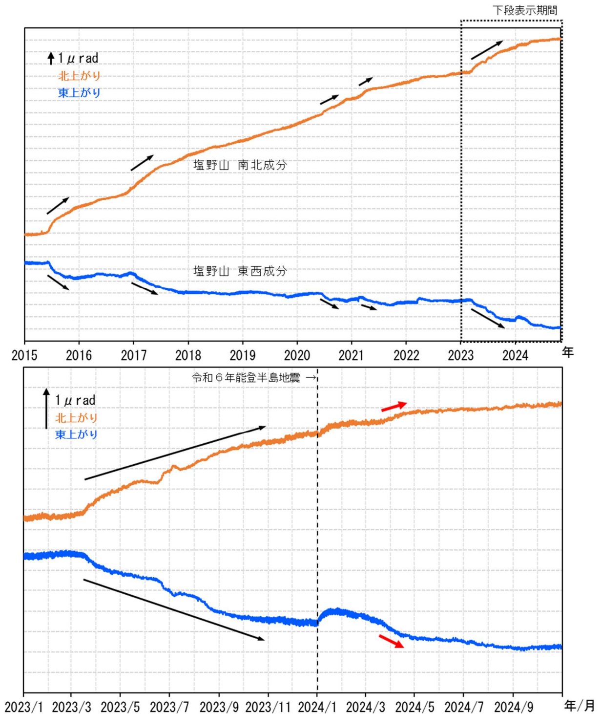
図6 浅間山 塩野山観測点における傾斜データ（2015年1月1日～2024年10月31日）
