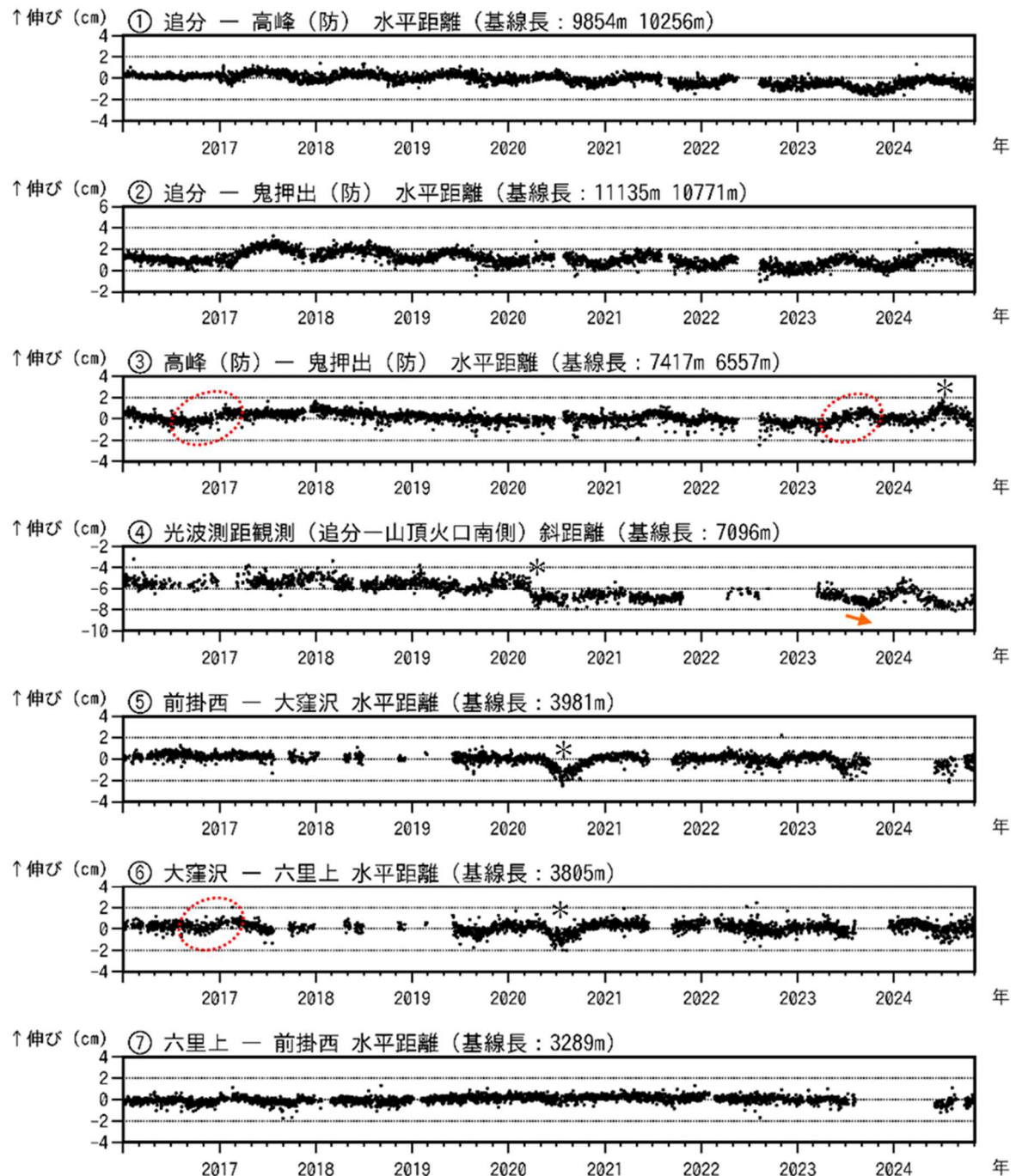
図7-1 浅間山 GNSS 連続観測及び光波測距観測結果(2016年1月1日~2024年10月31日)
