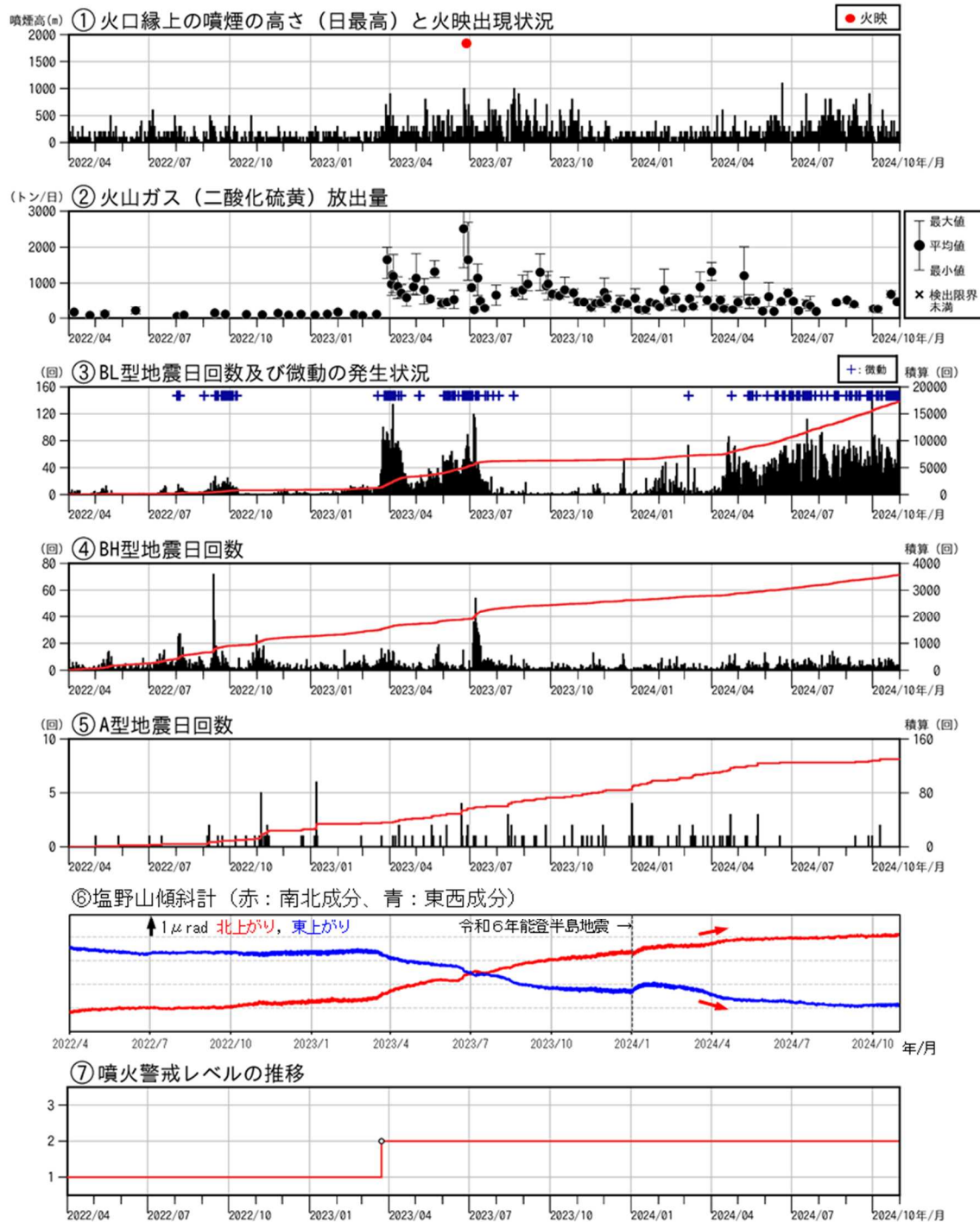
図2 浅間山 短期火山活動経過図（2022年4月1日～2024年10月31日）
