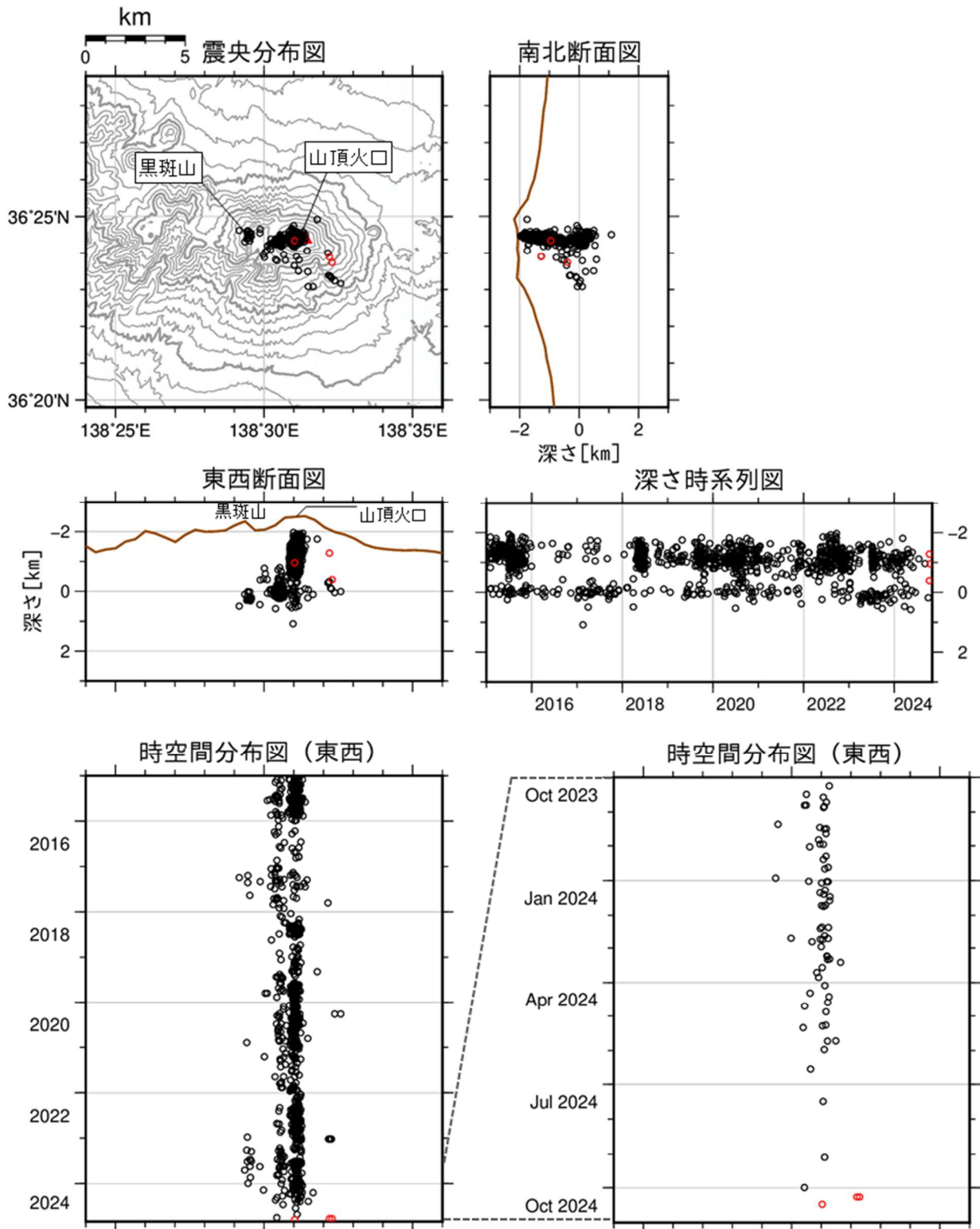
図5 浅間山 震源分布図（2015年1月1日～2024年10月31日）
