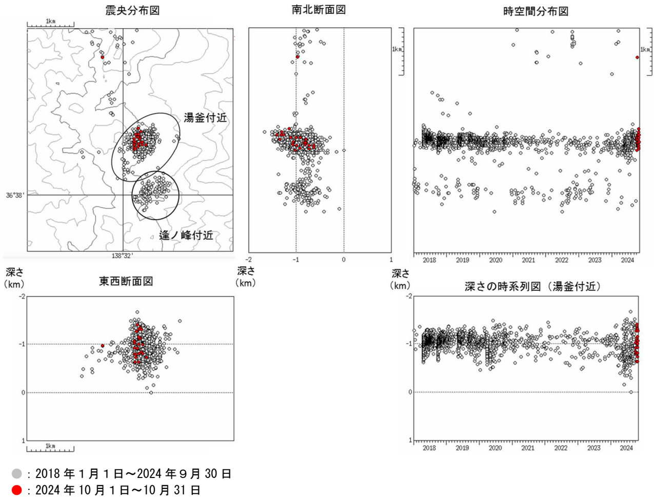
図4 草津白根山 震源分布図（2018 年 1 月 1 日～2024 年 10 月 31 日）
