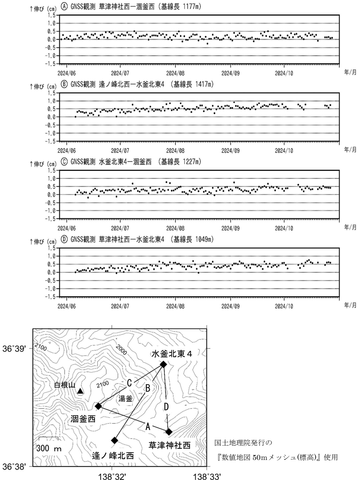
図6－1 草津白根山 湯釜近傍での臨時のGNSS連続観測結果
