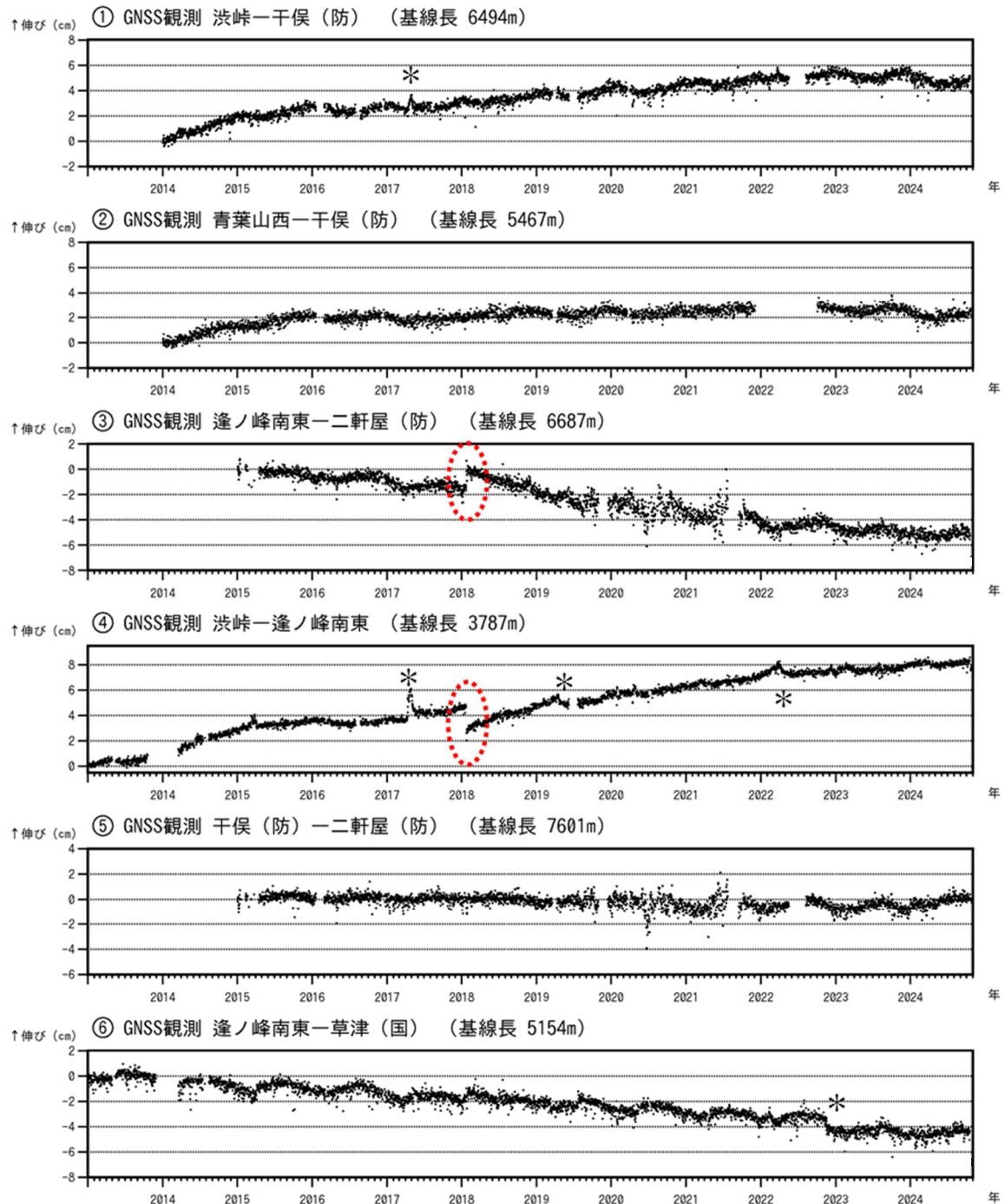
図6－2 草津白根山 GNSS 連続観測の結果（2013年1月1日～2024年10月31日）
