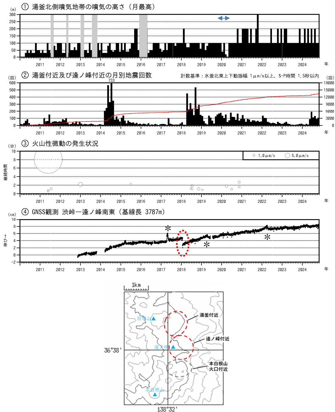
図3 草津白根山（白根山（湯釜付近）） 火山活動経過図（2010年1月1日～2024年10月31日）
