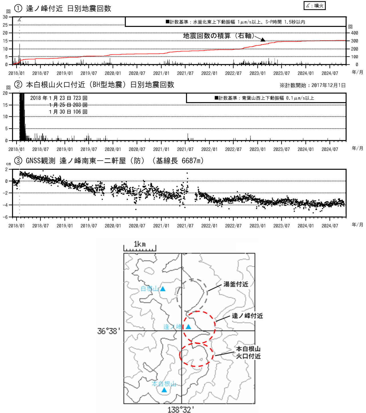
図13 草津白根山（本白根山） 火山活動経過図（2017年12月1日～2024年10月31日）
