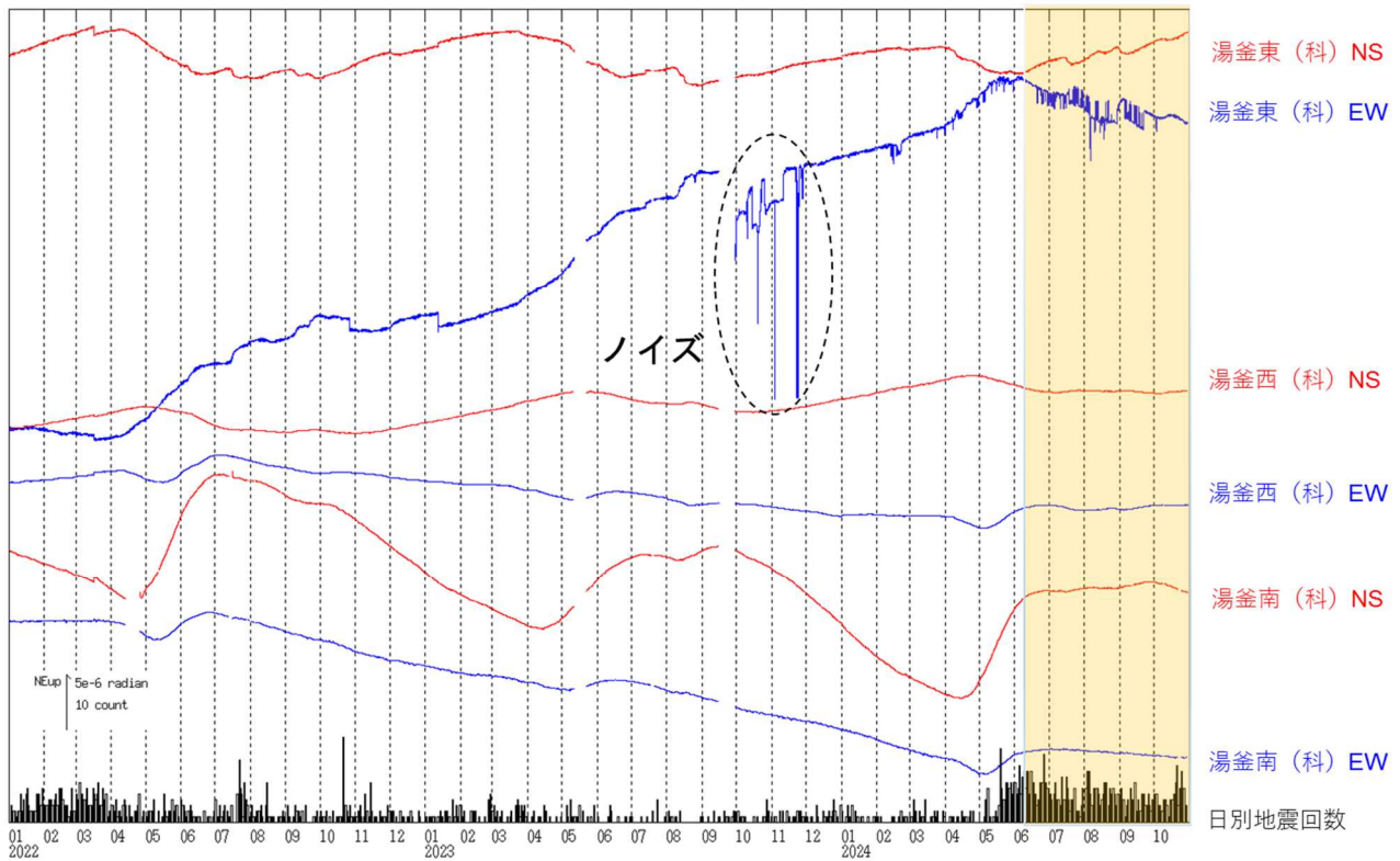
図5 草津白根山（白根山（湯釜付近）） 傾斜変動（2022年1月1日～2024年10月31日）
