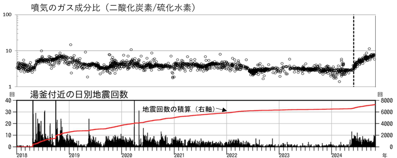
図8 草津白根山（白根山（湯釜付近）） 火山ガス観測結果（2018年1月～2024年10月）
